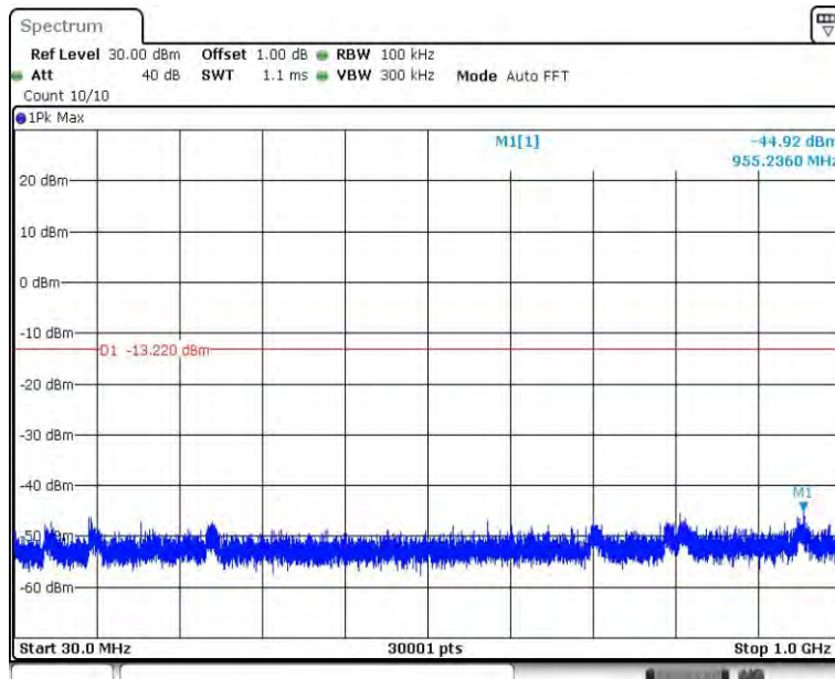
11N20MIMO Ant2 2412 30~1000
