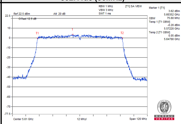
802.11ac (80MHz)
