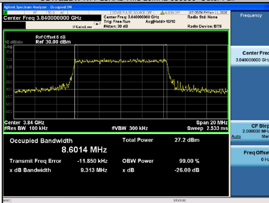
OBW&amp;EBW N77 15KHz TM3 10MHz 656000 Outer Full
