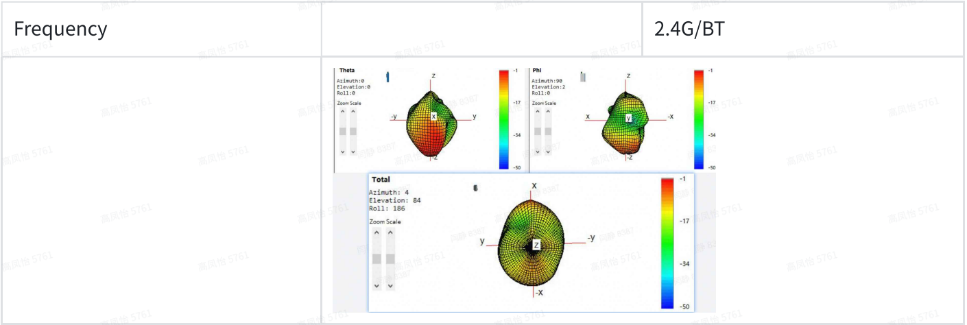
方向图
