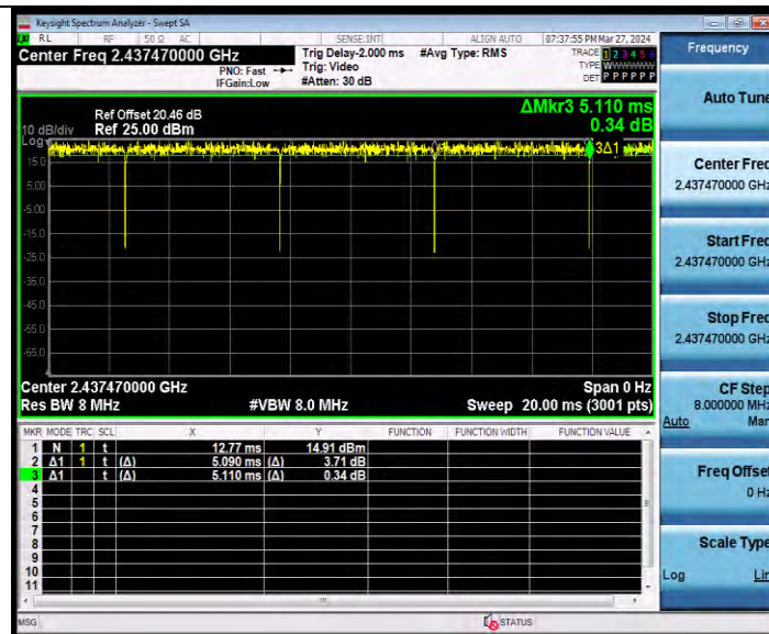
11AX20MIMO_Ant1_2437_52Tone_RU38
