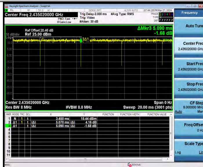
11AX20MIMO_Ant1_2437_106Tone_RU53
