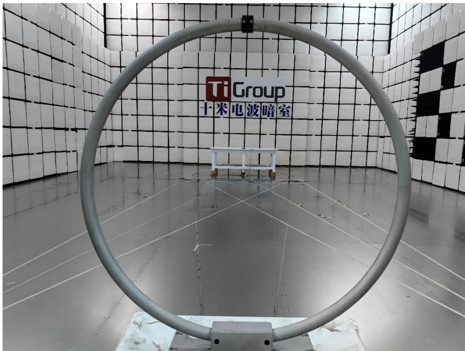
Below 30MHz-BT/WIFI
