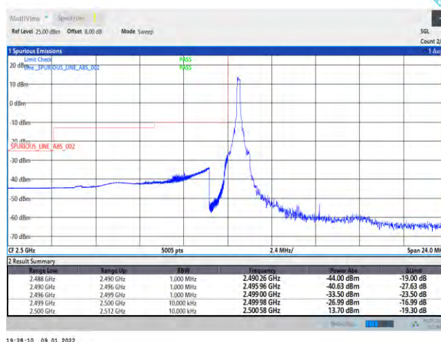
Band7-10MHz-QPSK-20800-50RB#0
