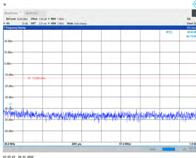
Band2-20MHz-QPSK-19100-1RB#0-Range4:1000~20000MHz
