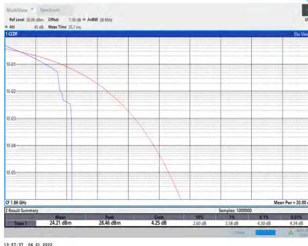
Band2-20MHz-QPSK-18700-100RB#0
