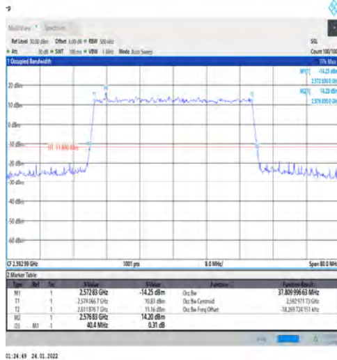
1-N41-PC3-30-40-M-7-CP-16QAM-Outer_Full-106@ 0-Ant1-37.81-40.400-≤40-PASS
