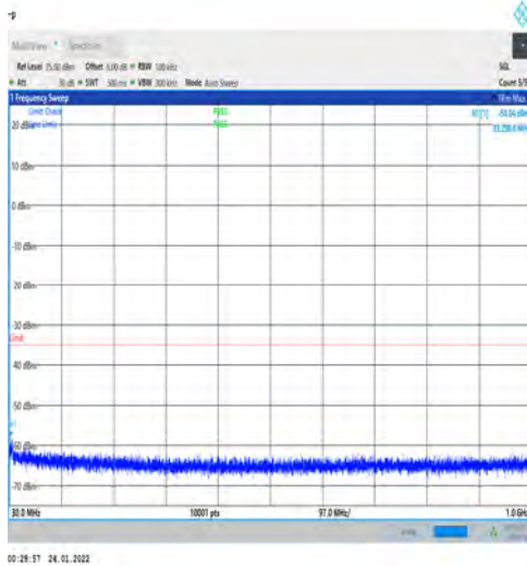
1-N41-PC3-30-100-L-1-DFT-PI2BPSK-Edge_1RB_L eft-1@0-30-1000-Ant1--58.04--35-PASS
