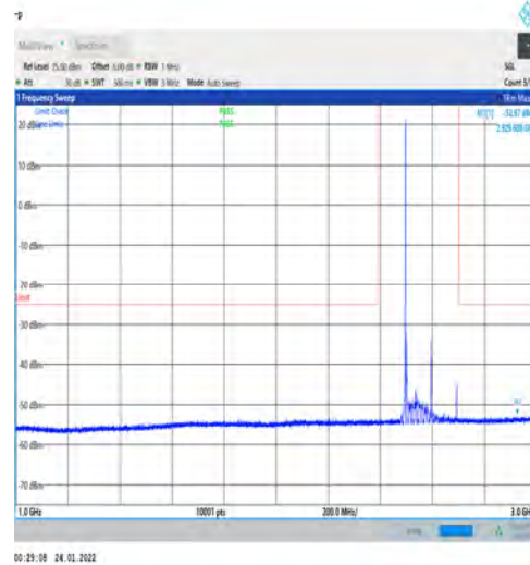
1-N41-PC3-30-100-L-1-DFT-PI2BPSK-Edge_1RB_L eft-1@0-1000-3000-Ant1--52.67--25-PASS
