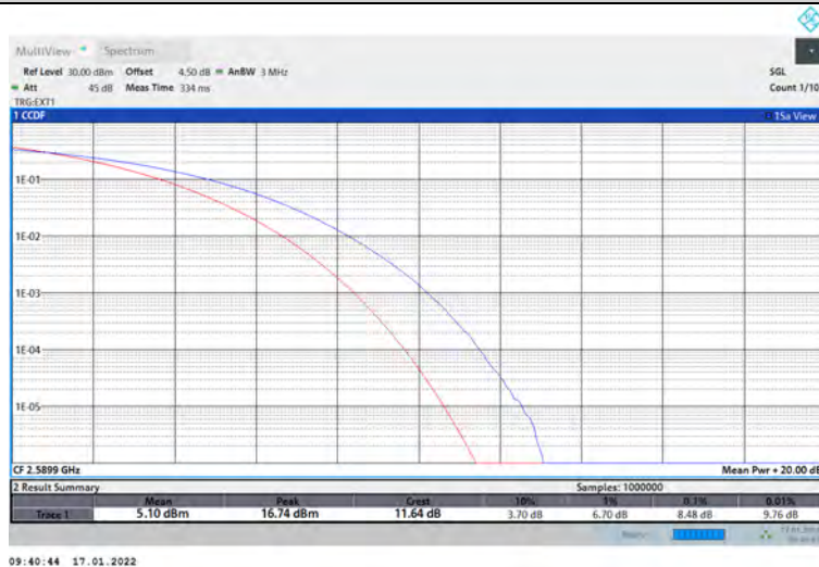
CA_38C-20MHz-20MHz-QPSK-QPSK-37901-38099-100RB#0-100RB#0
