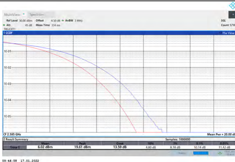
CA_38C-20MHz-20MHz-QPSK-QPSK-37901-38099-100RB#0-100RB#0
