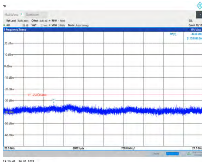
Band41-20MHz-256QAM-41490-1RB#0-Range5:20000~27000MHz
