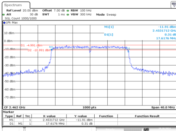
802.11n20_2462MHz 17.618MHz
