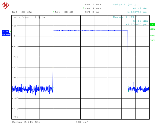
DH3_Hopping
