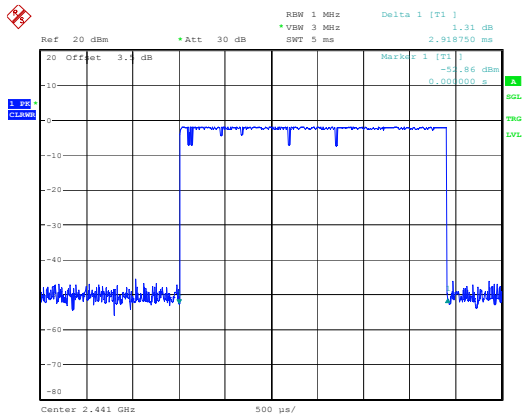
DH5_Hopping
