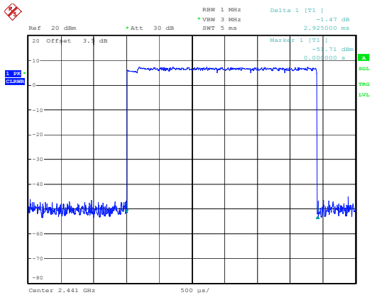
2DH5_Hopping
