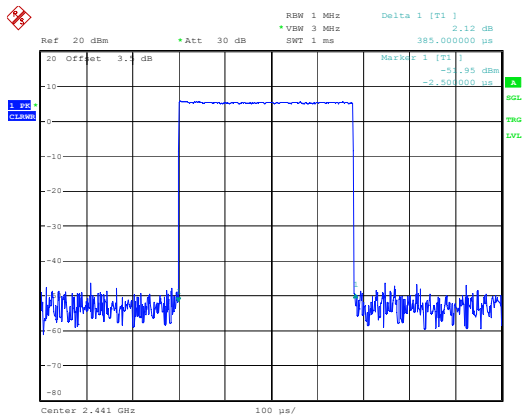
DH1_Hopping
