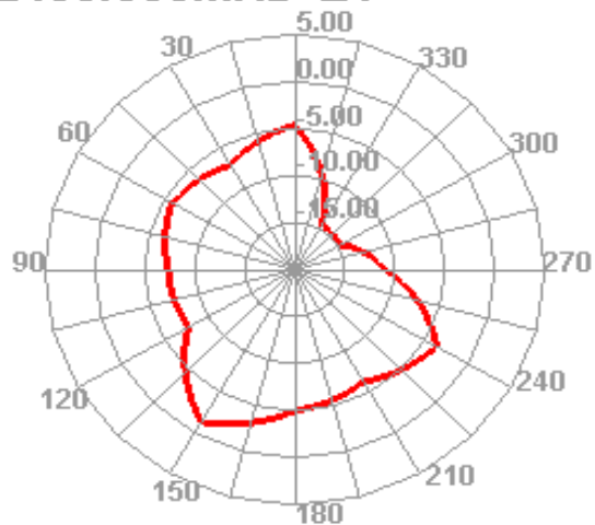
2450.000MHz E1
