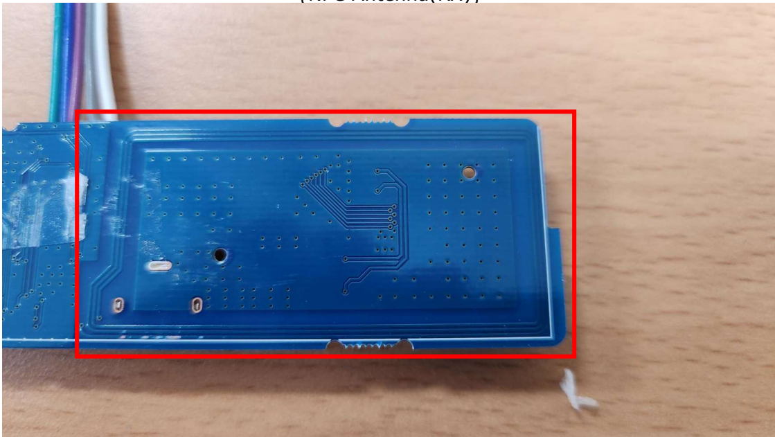
{NFC Antenna(RX)}
