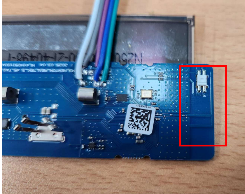
{2401-2480MHz PCB Antenna(TX, RX)}
