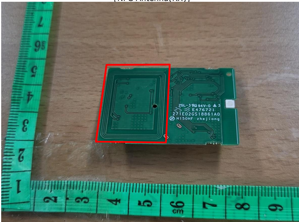
{NFC Antenna(RX)}
