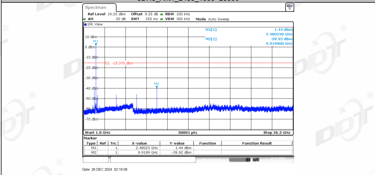
3DH5 Ant1 2480 1000~26500
