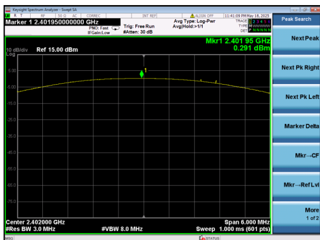
\pi/4 -DQPSK LOW CHANNEL
