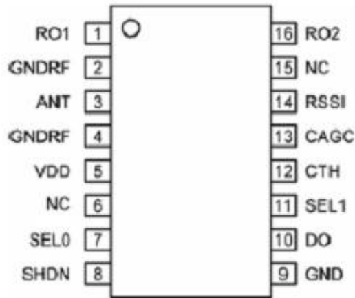
218R SOP16和219R SSOP16封装引脚图
