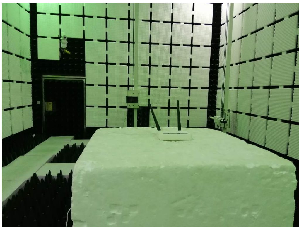
Fig. 3(Model 1:ICP30A-120-1500)
