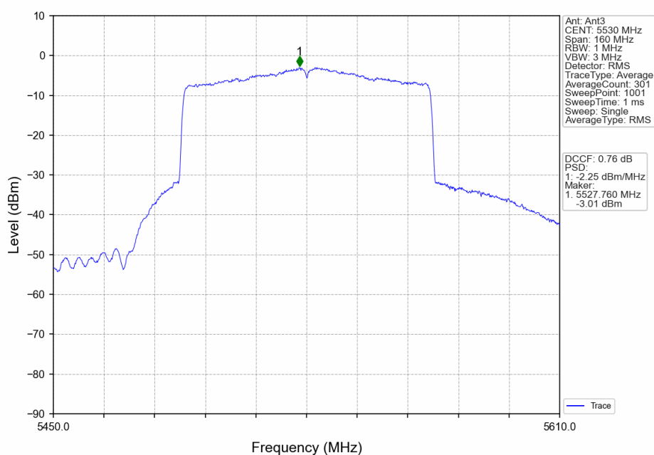
802.11ax(HEW80)_LCH_5530MHz_RU996_Left_Ant3_NTNV
