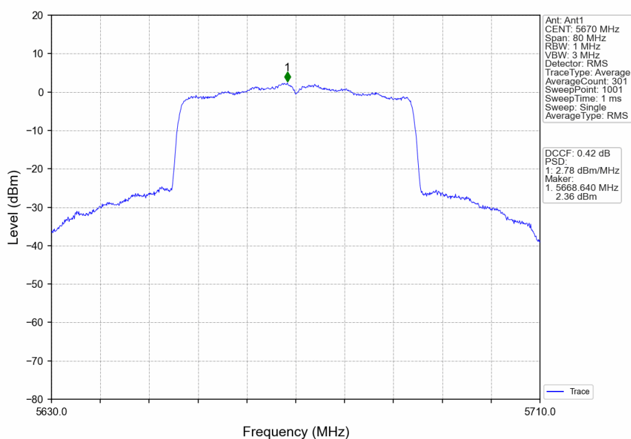
802.11ax(HEW40)_HCH_5670MHz_RU484_Left_Ant1_NTNV
