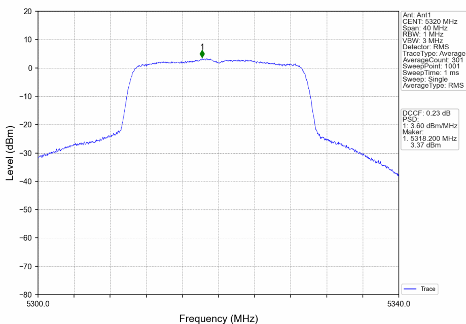
802.11ax(HEW20)_HCH_5320MHz_RU242_Left_Ant1_NTNV
