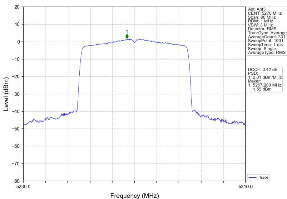
802.11ax(HEW40)_LCH_5270MHz_RU484_Left_Ant3_NTNV
