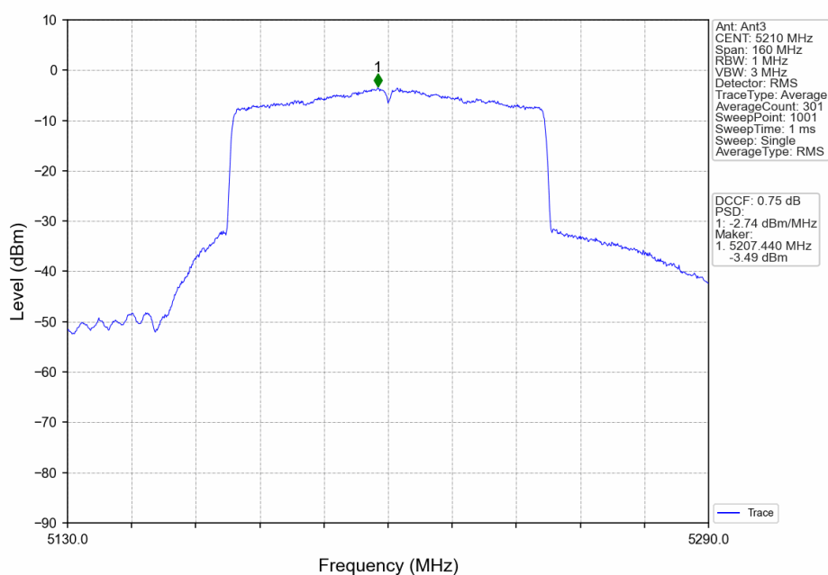
802.11ax(HEW80)_MCH_5210MHz_RU996_Left_Ant3_NTNV
