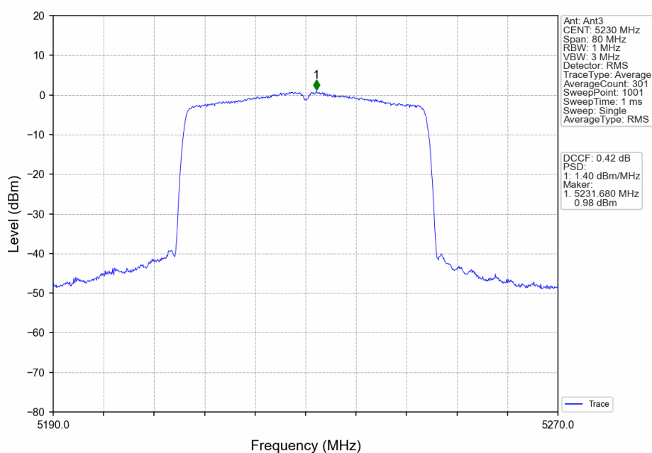
802.11ax(HEW40)_HCH_5230MHz_RU484_Left_Ant3_NTNV
