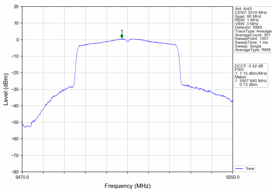
802.11ax(HEW40)_LCH_5510MHz_RU484_Left_Ant3_NTNV
