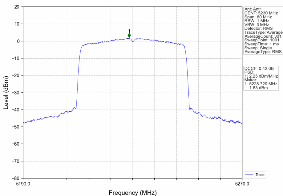
802.11ax(HEW40)_HCH_5230MHz_RU484_Left_Ant1_NTNV
