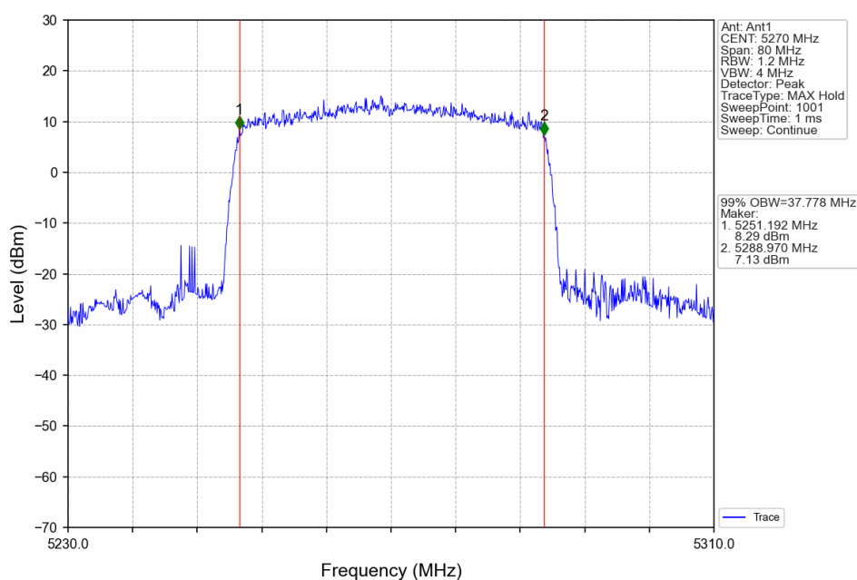
802.11ax(HEW40)_LCH_5270MHz_RU484_Left_Ant1_NTNV
