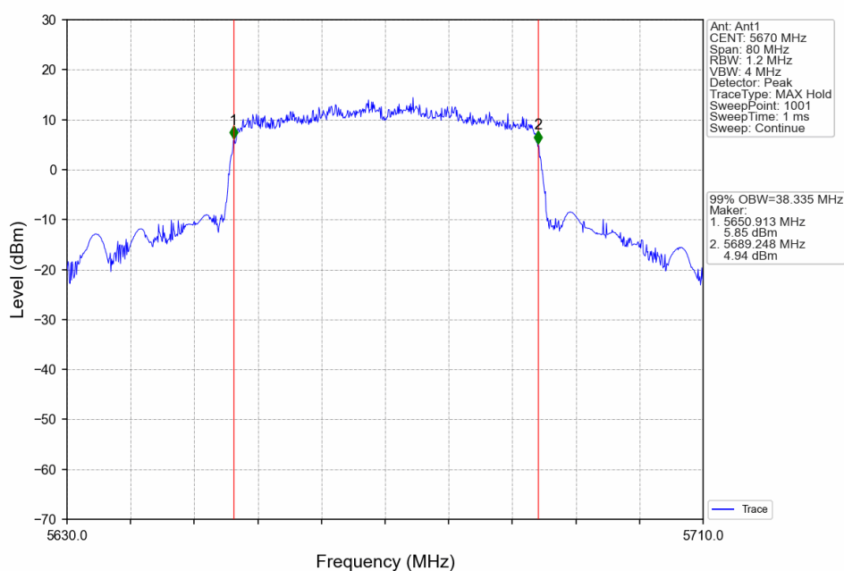
802.11ax(HEW40)_HCH_5670MHz_RU484_Left_Ant1_NTNV
