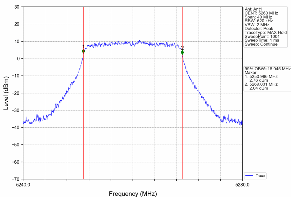
802.11n(HT20)_LCH_5260MHz_Ant1_NTNV
