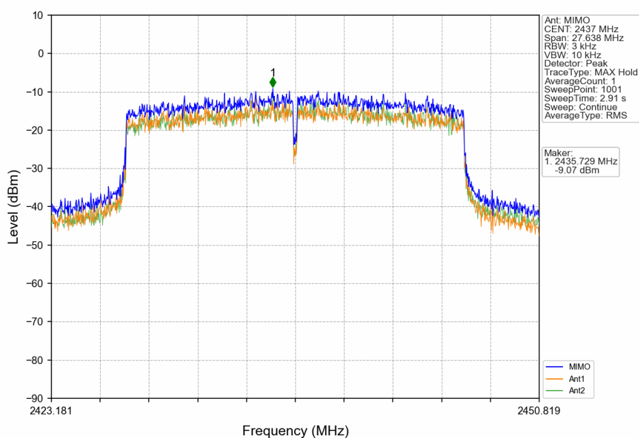
802.11ax(HEW20)_MCH_2437MHz_RU242_Left_MIMO_NTNV
