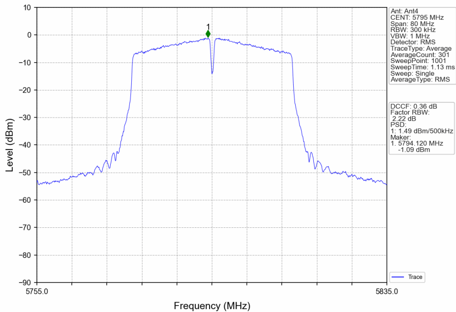
802.11n(HT40)_HCH_5795MHz_Ant4_NTNV
