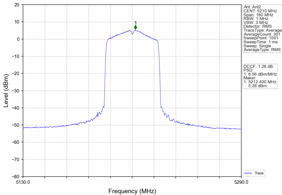
802.11ax(HEW80)_MCH_5210MHz_RU996_Left_Ant2_NTNV
