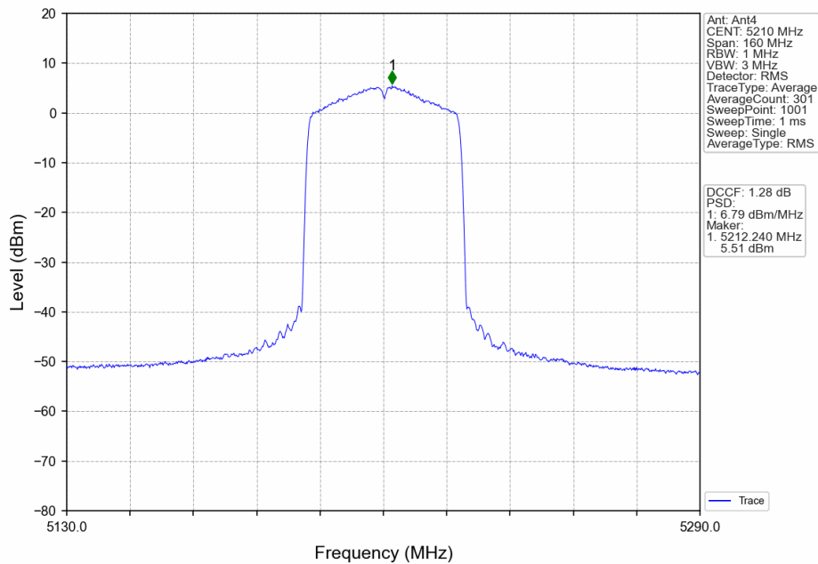
802.11ax(HEW80)_MCH_5210MHz_RU996_Left_Ant4_NTNV
