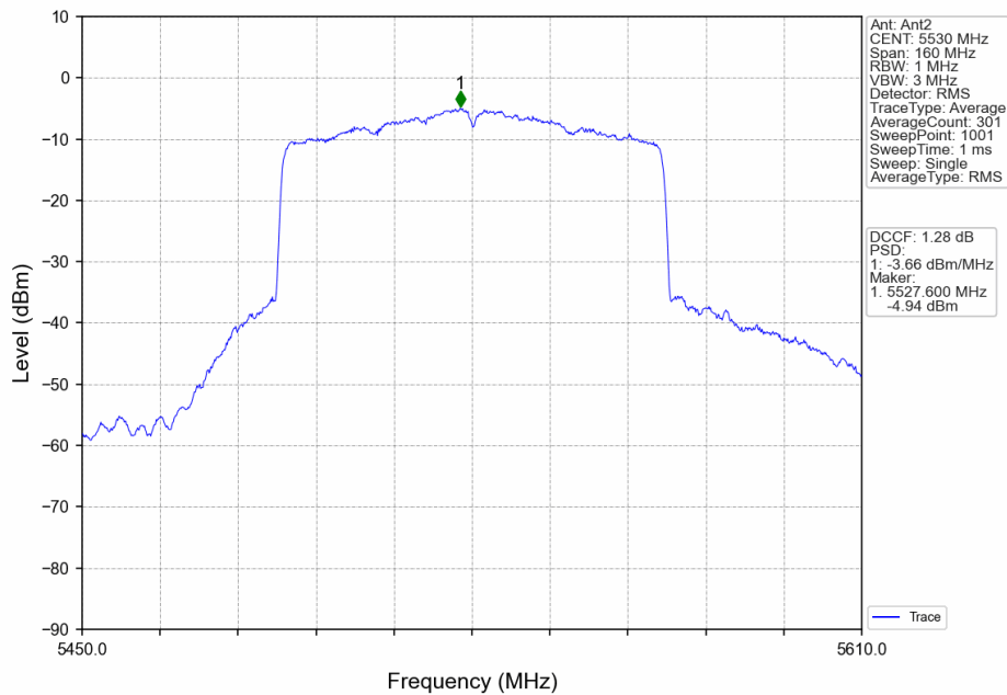
802.11ax(HEW80)_LCH_5530MHz_RU996_Left_Ant2_NTNV
