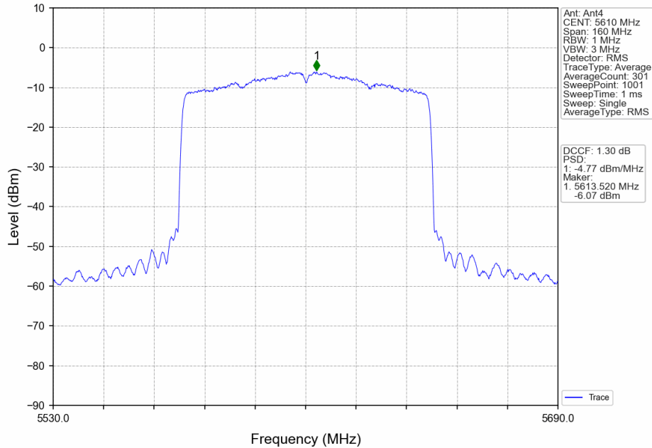
802.11ax(HEW80)_HCH_5610MHz_RU996_Left_MIMO_NTNV
