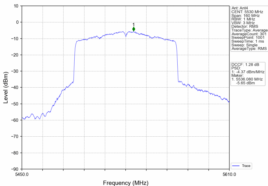
802.11ax(HEW80)_LCH_5530MHz_RU996_Left_Ant4_NTNV
