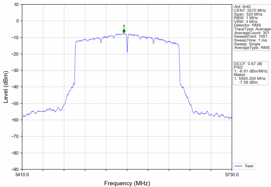
802.11ax(HEW160)_MCH_5570MHz_2xRU996_Left_Ant2_NTNV
