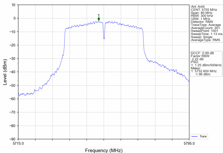
802.11ac(VHT40)_LCH_5755MHz_Ant4_NTNV
