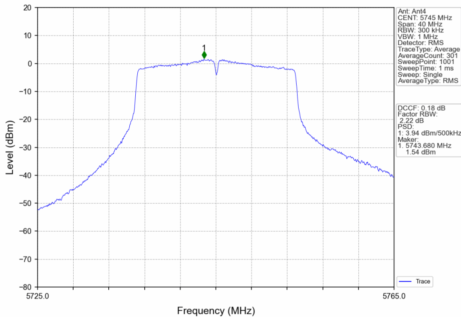
802.11n(HT20)_LCH_5745MHz_Ant4_NTNV
