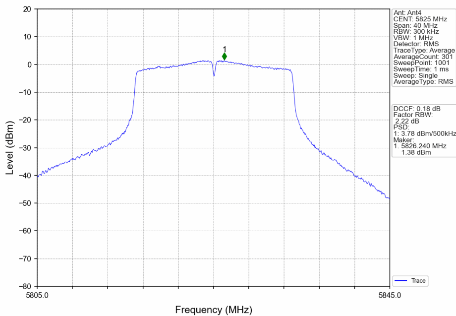
802.11n(HT20)_HCH_5825MHz_Ant4_NTNV
