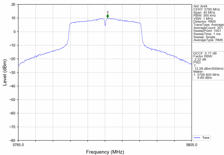
802.11a_MCH_5785MHz_Ant4_NTNV
