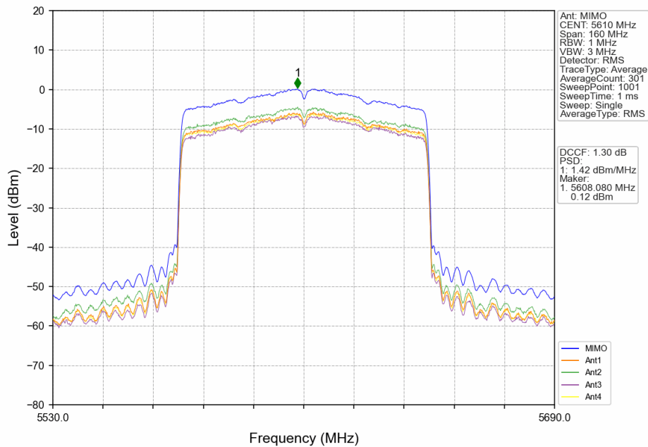
802.11ax(HEW80)_HCH_5610MHz_RU996_Left_MIMO_NTNV
