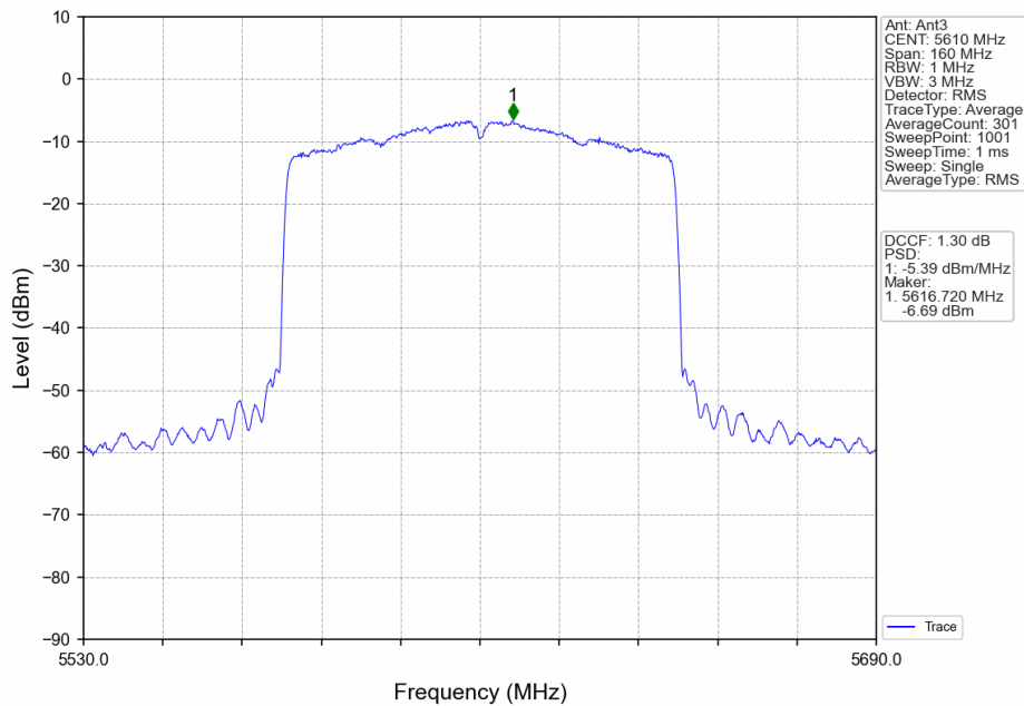
802.11ax(HEW80)_HCH_5610MHz_RU996_Left_Ant3_NTNV
