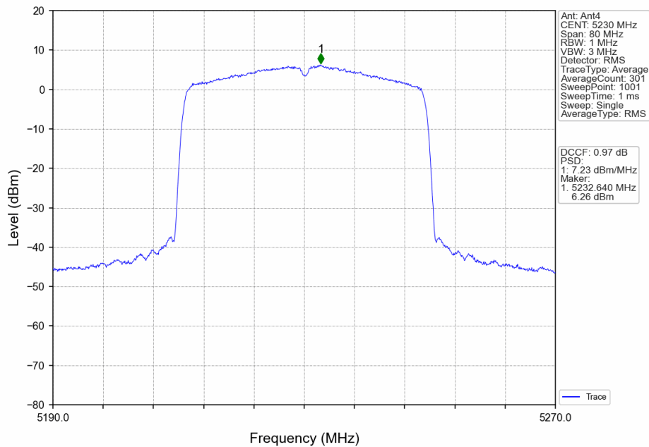
802.11ax(HEW40)_HCH_5230MHz_RU484_Left_Ant4_NTNV
