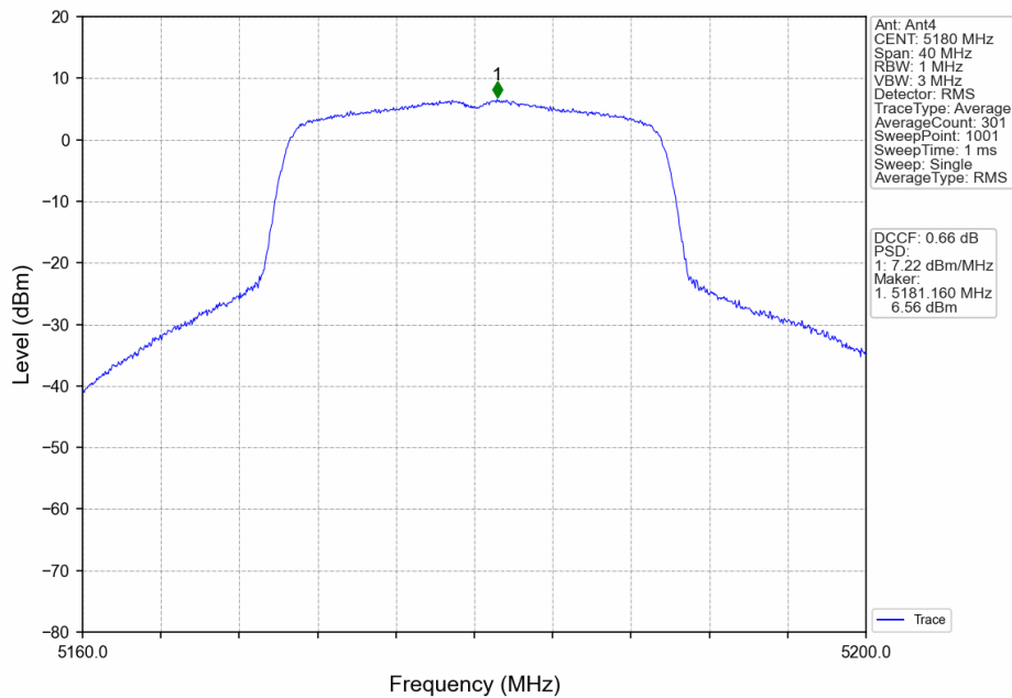
802.11ax(HEW20)_LCH_5180MHz_RU242_Left_Ant4_NTNV
