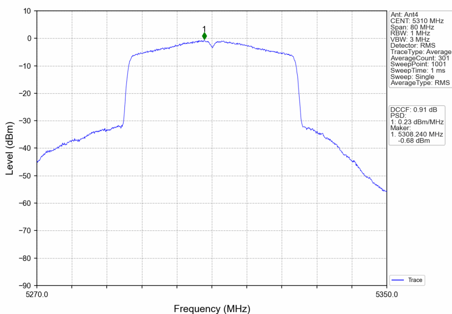
802.11ax(HEW40)_HCH_5310MHz_RU484_Left_Ant4_NTNV
