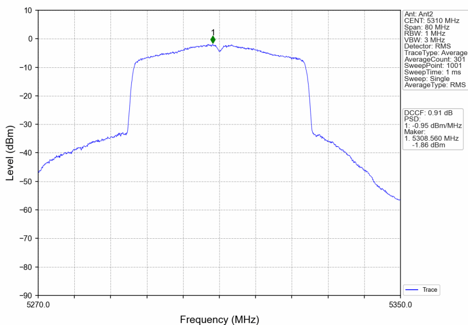
802.11ax(HEW40)_HCH_5310MHz_RU484_Left_Ant2_NTNV
