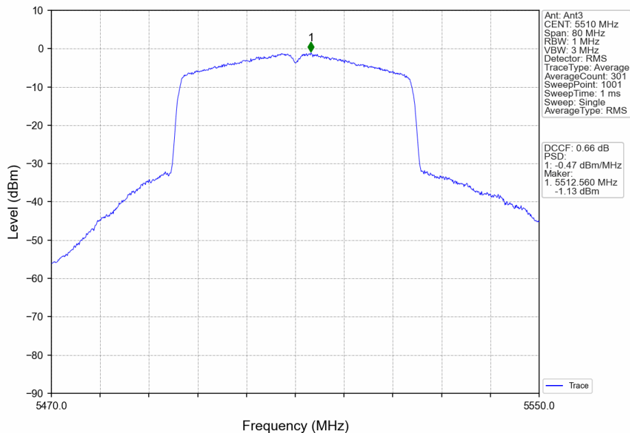
802.11ax(HEW40)_LCH_5510MHz_RU484_Left_Ant3_NTNV
