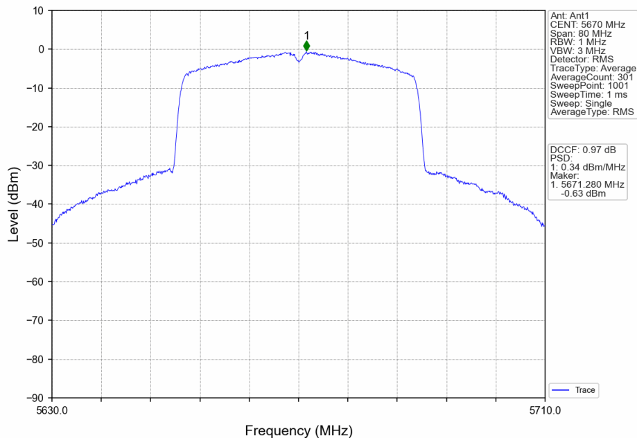
802.11ax(HEW40)_HCH_5670MHz_RU484_Left_Ant1_NTNV
