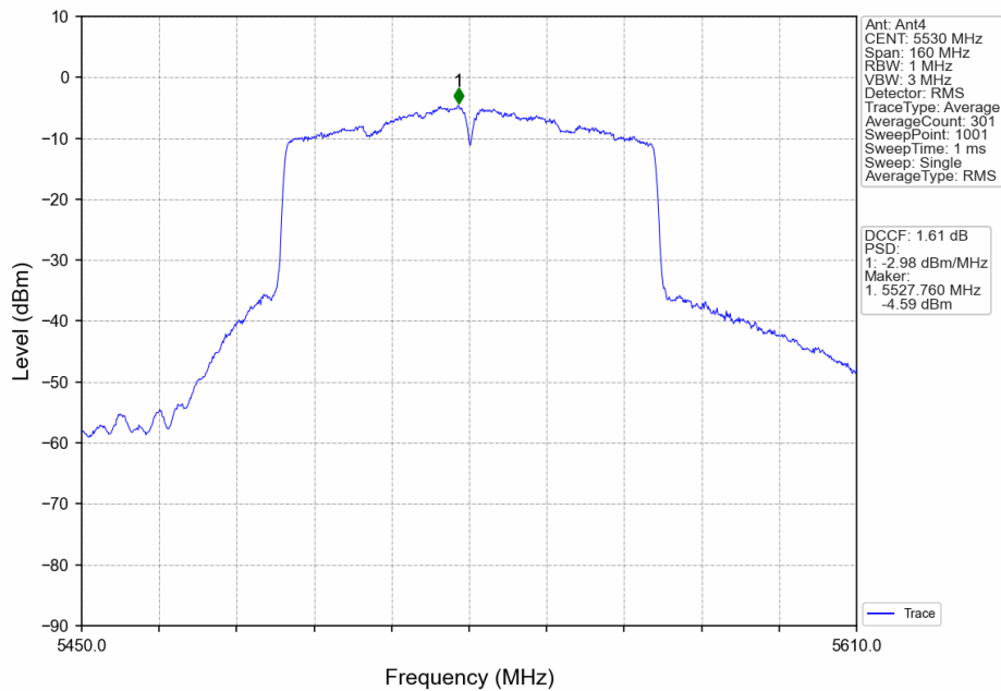
802.11ac(VHT80)_LCH_5530MHz_Ant4_NTNV
