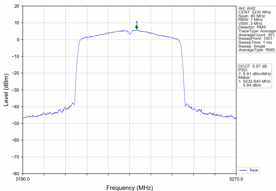
802.11ax(HEW40)_HCH_5230MHz_RU484_Left_Ant2_NTNV
