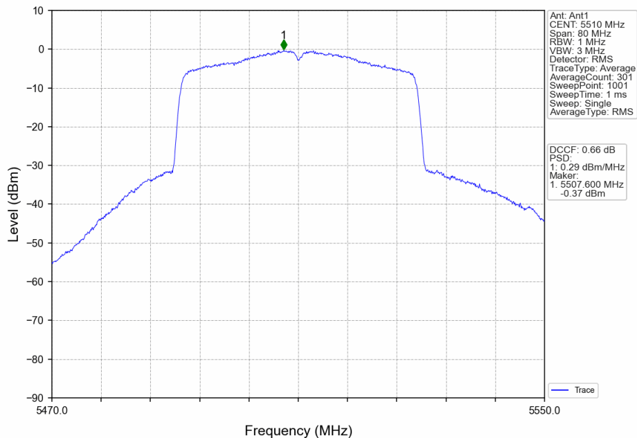
802.11ax(HEW40)_LCH_5510MHz_RU484_Left_Ant1_NTNV
