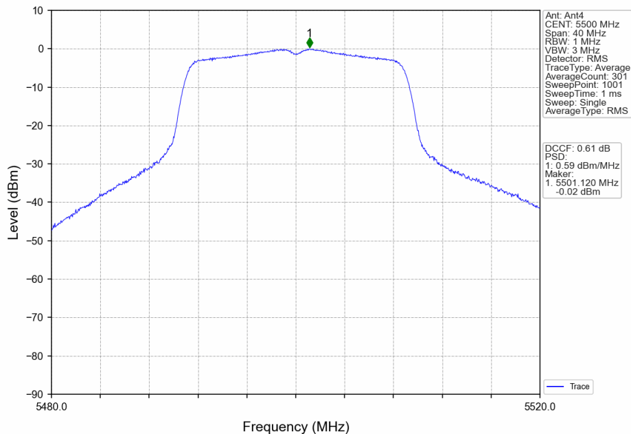
802.11ac(VHT20)_LCH_5500MHz_Ant4_NTNV
