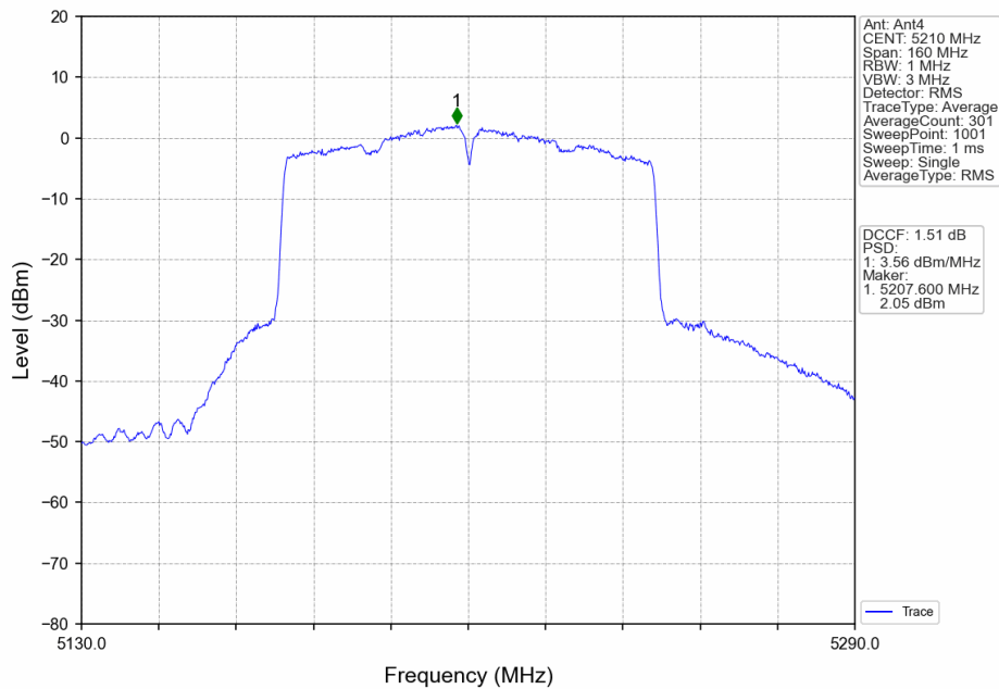
802.11ac(VHT80)_MCH_5210MHz_Ant4_NTNV
