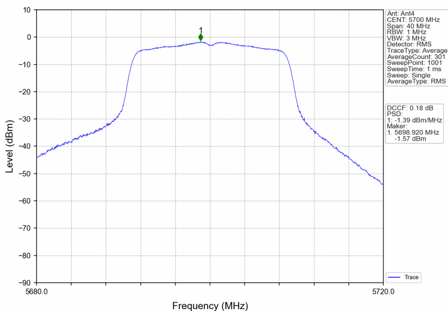
802.11n(HT20)_HCH_5700MHz_Ant4_NTNV
