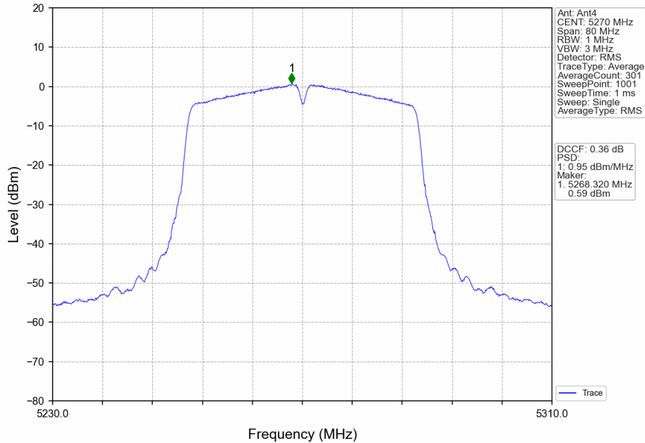
802.11n(HT40)_LCH_5270MHz_MIMO_NTNV
