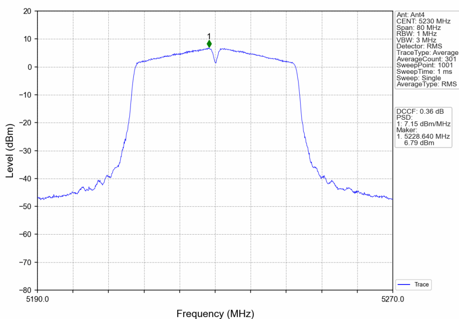
802.11n(HT40)_HCH_5230MHz_Ant4_NTNV
