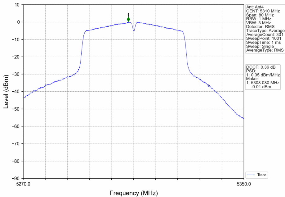
802.11n(HT40)_HCH_5310MHz_Ant4_NTNV
