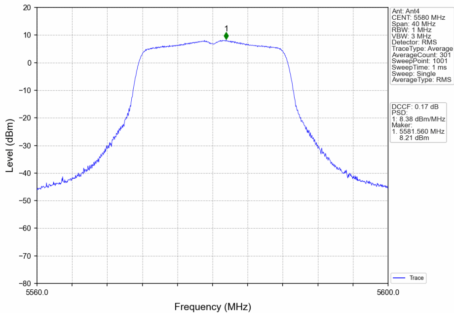
802.11a_MCH_5580MHz_Ant4_NTNV
