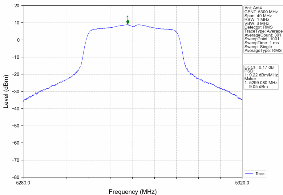
802.11a_MCH_5300MHz_Ant4_NTNV
