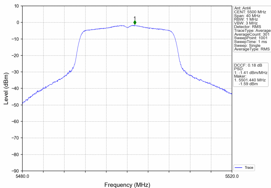
802.11n(HT20)_LCH_5500MHz_Ant4_NTNV
