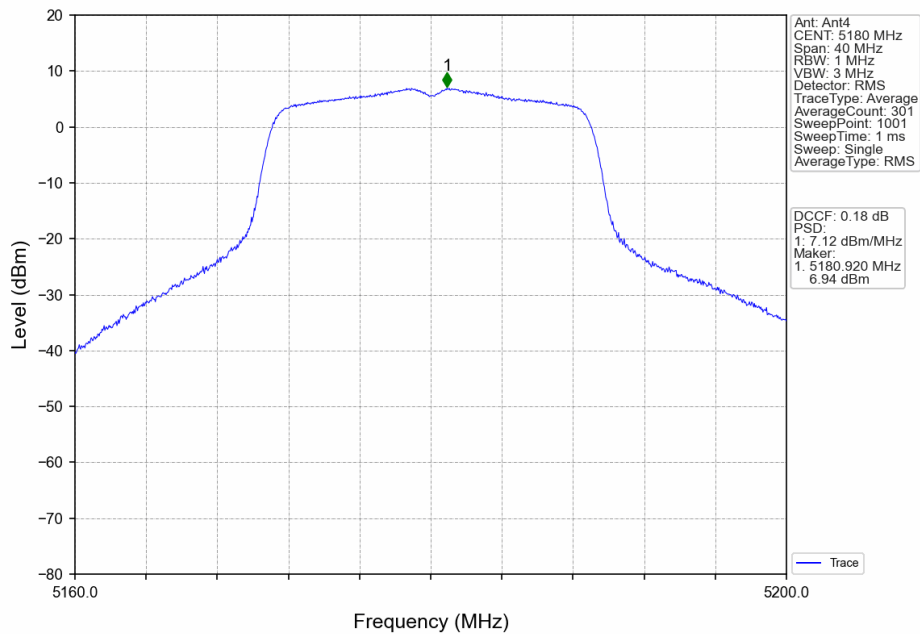
802.11n(HT20)_LCH_5180MHz_Ant4_NTNV
