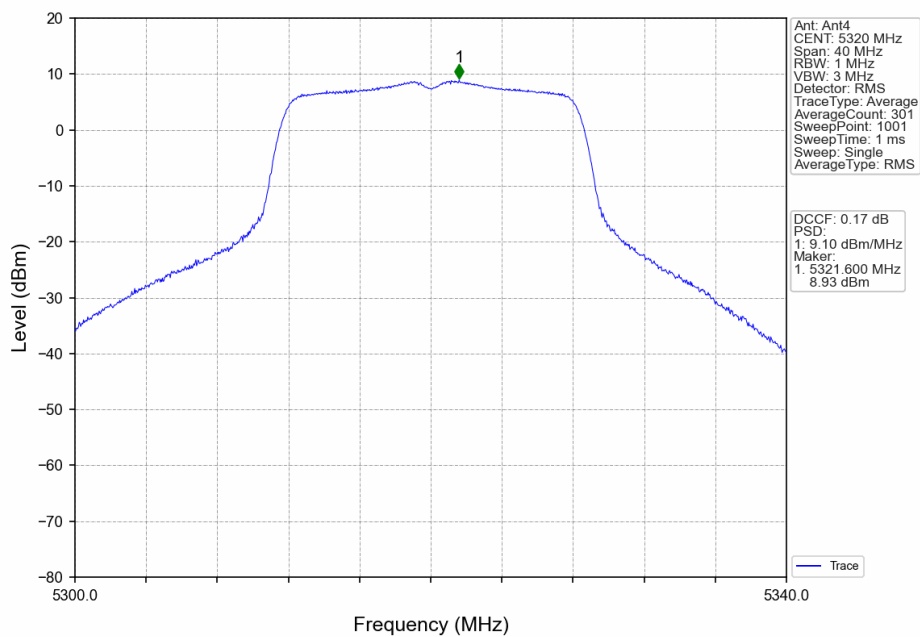
802.11a_HCH_5320MHz_Ant4_NTNV
