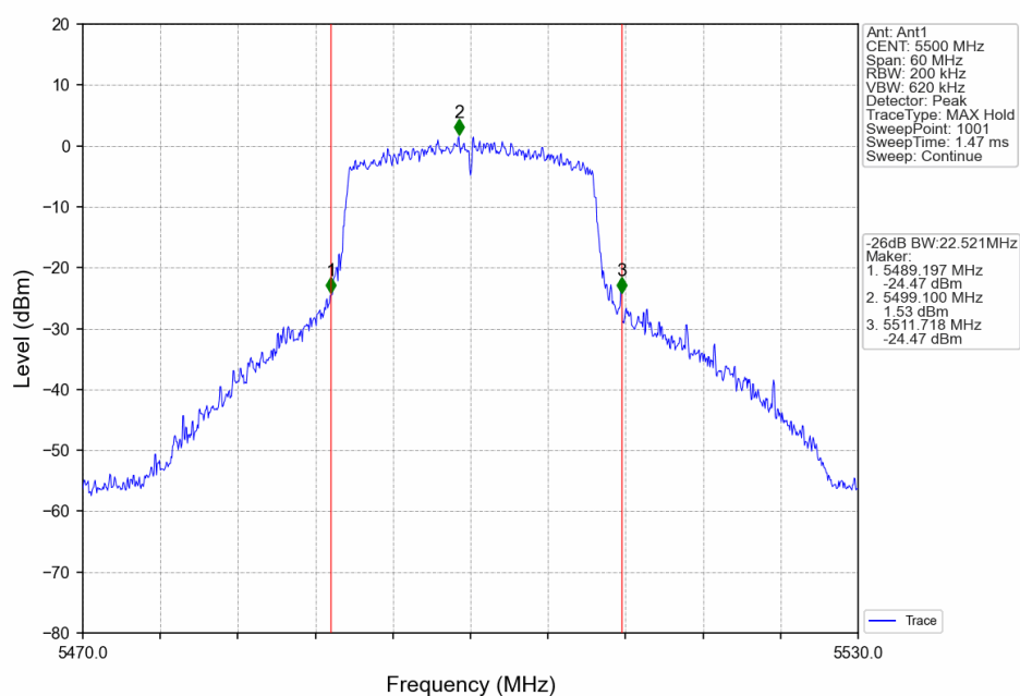
802.11ax(HEW20)_LCH_5500MHz_RU242_Left_Ant1_NTNV
