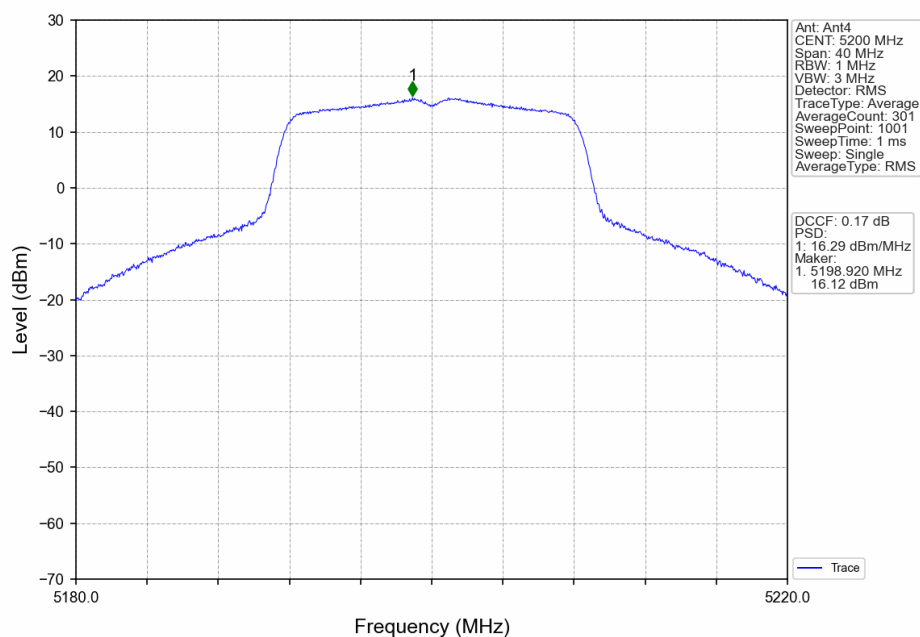
802.11a_MCH_5200MHz_Ant4_NTNV
