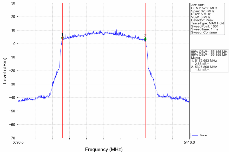
802.11ax(HEW160)_MCH_5250MHz_2xRU996_Left_Ant1_NTNV
