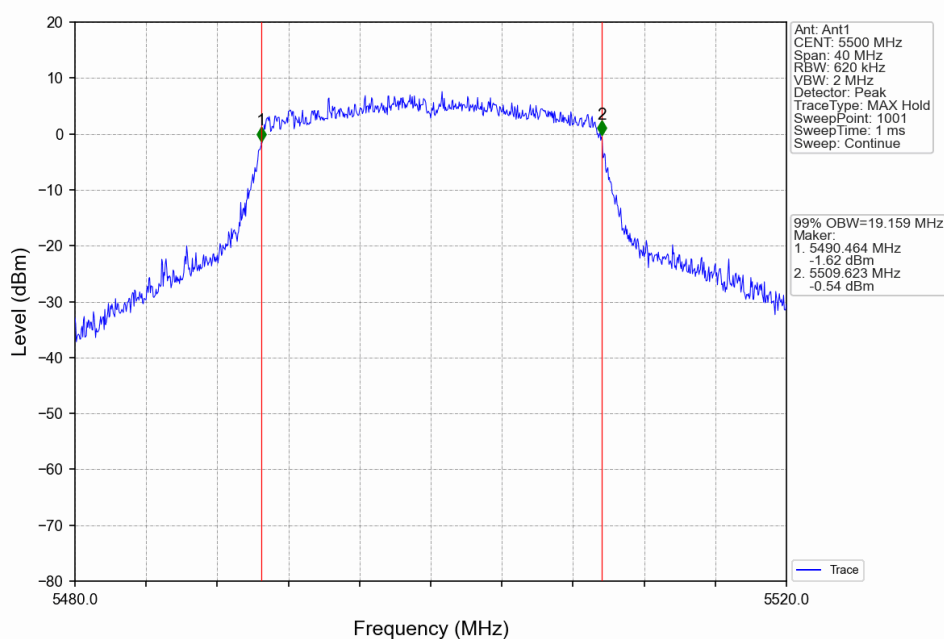
802.11ax(HEW20)_LCH_5500MHz_RU242_Left_Ant1_NTNV
