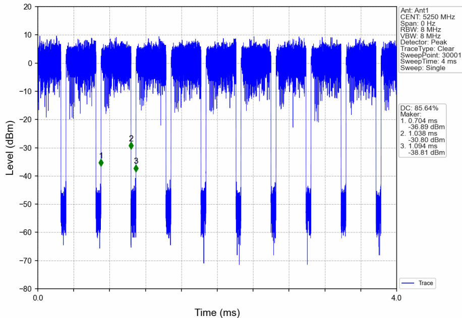
802.11ax(HEW160)_MCH_5250MHz_2xRU996_Left_Ant1_NTNV
