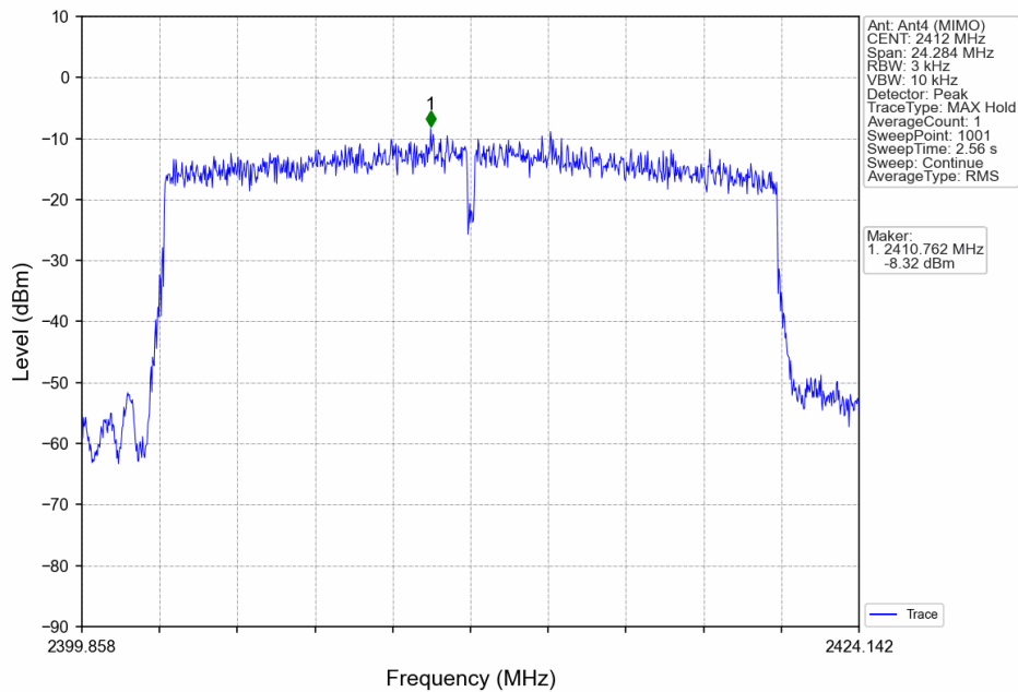
802.11ax(HEW20)_LCH_2412MHz_RU242_Left_Ant4 (MIMO)_NTNV
