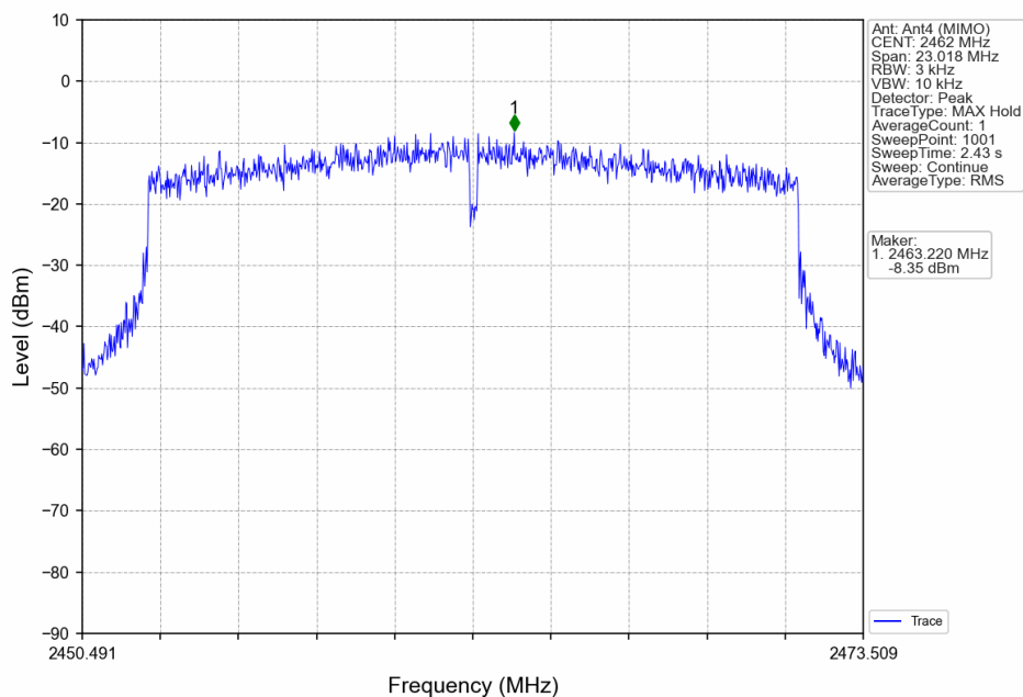
802.11ax(HEW20)_HCH_2462MHz_RU242_Left_Ant4 (MIMO)_NTNV
