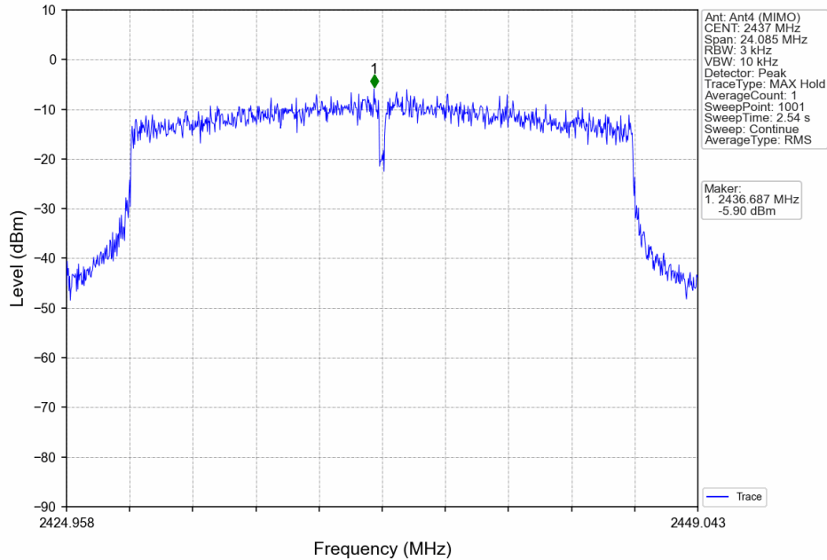
802.11ax(HEW20)_MCH_2437MHz_RU242_Left_MIMO_NTNV
