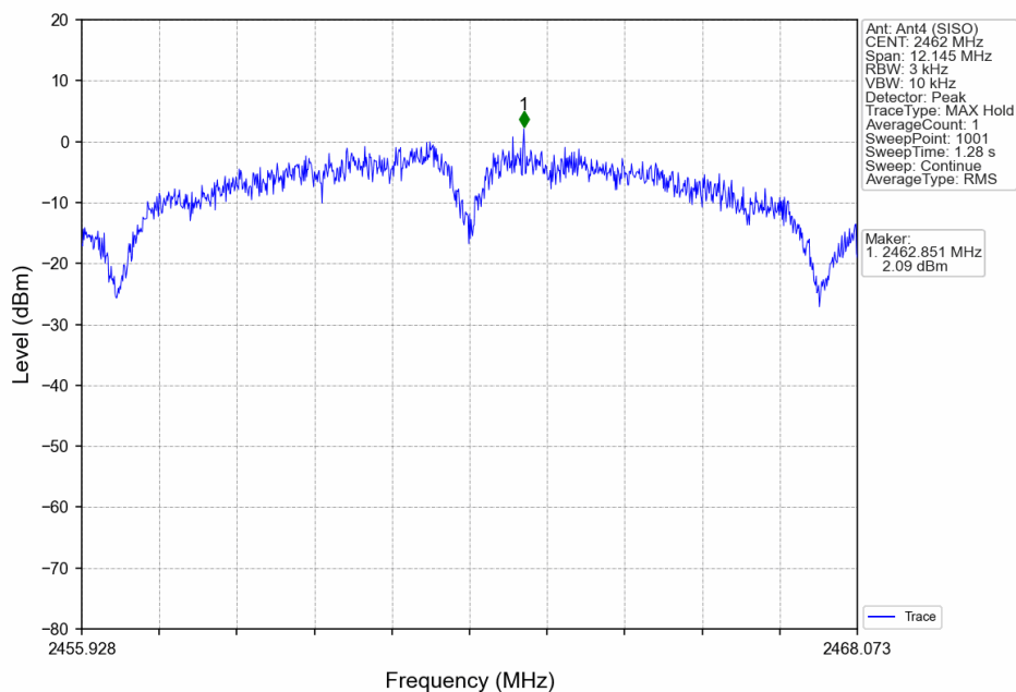
802.11b_HCH_2462MHz_Ant4 (SISO)_NTNV
