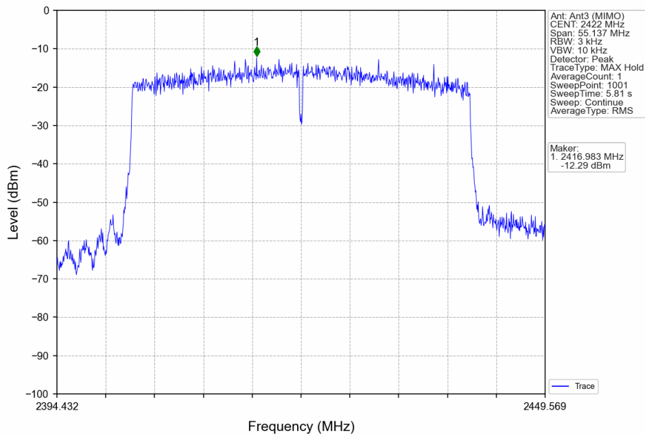
802.11ax(HEW40)_LCH_2422MHz_RU484_Left_Ant3 (MIMO)_NTNV
