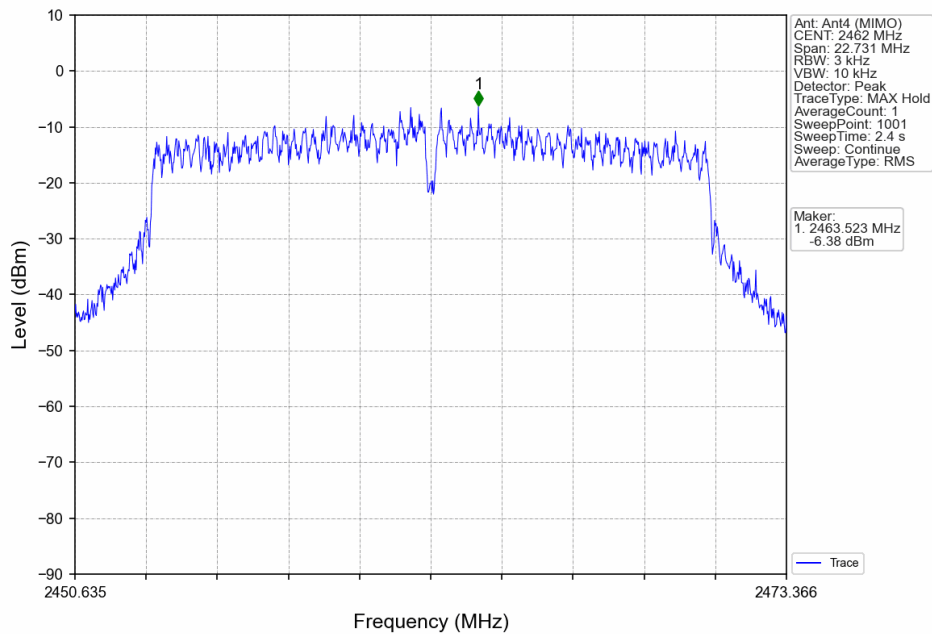
802.11n(HT20)_HCH_2462MHz_Ant4 (MIMO)_NTNV
