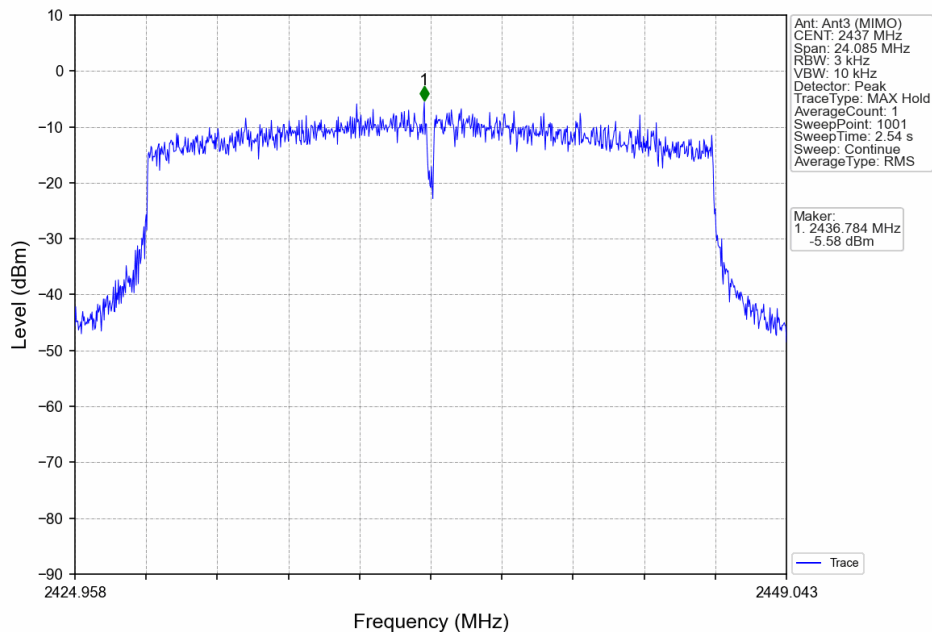
802.11ax(HEW20)_MCH_2437MHz_RU242_Left_Ant3 (MIMO)_NTNV
