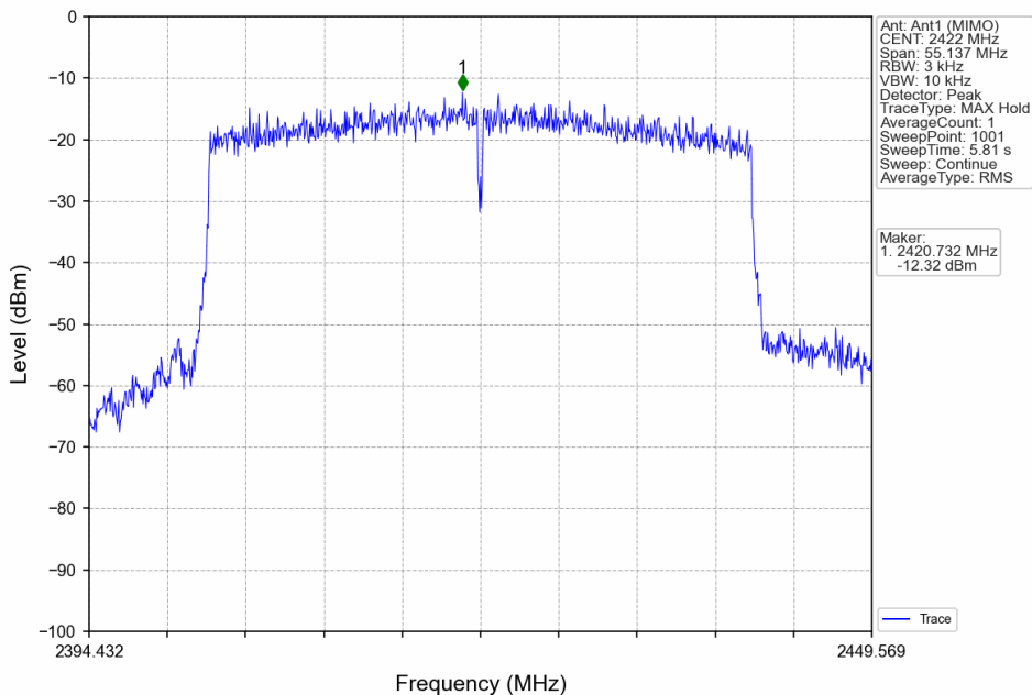
802.11ax(HEW40)_LCH_2422MHz_RU484_Left_Ant1 (MIMO)_NTNV
