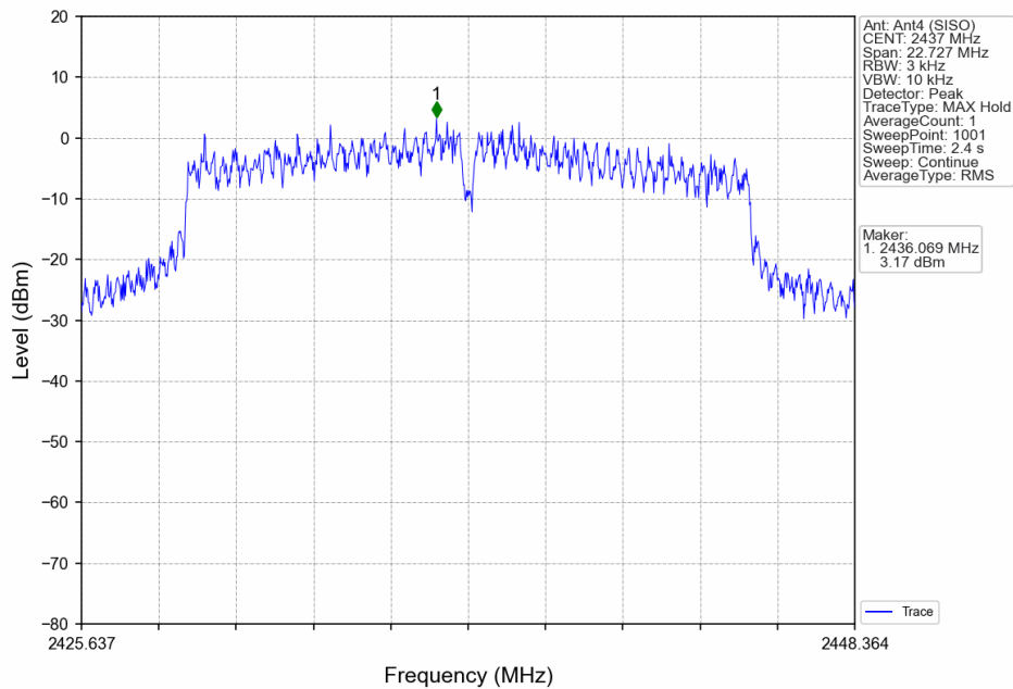
802.11g_MCH_2437MHz_Ant4 (SISO)_NTNV
