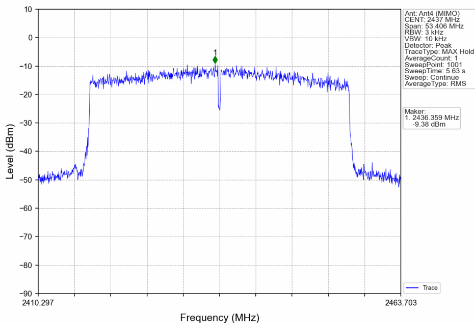
802.11ax(HEW40)_MCH_2437MHz_RU484_Left_Ant4 (MIMO)_NTNV
