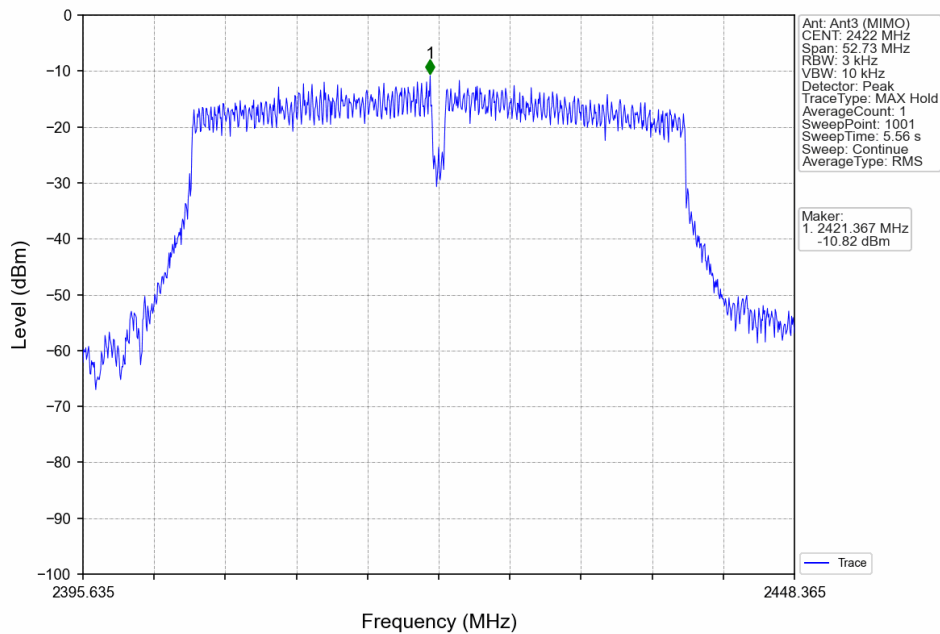
802.11n(HT40)_LCH_2422MHz_Ant3 (MIMO)_NTNV
