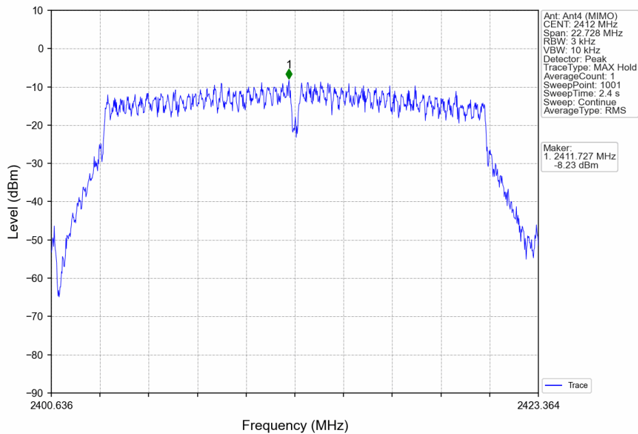
802.11n(HT20)_LCH_2412MHz_Ant4 (MIMO)_NTNV
