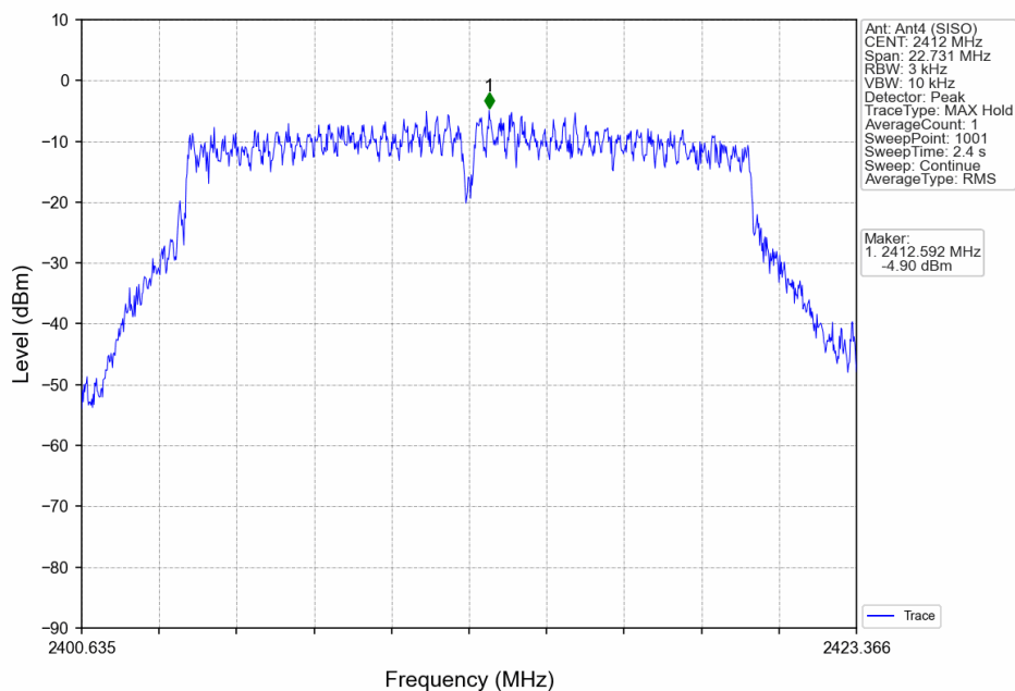
802.11g_LCH_2412MHz_Ant4 (SISO)_NTNV
