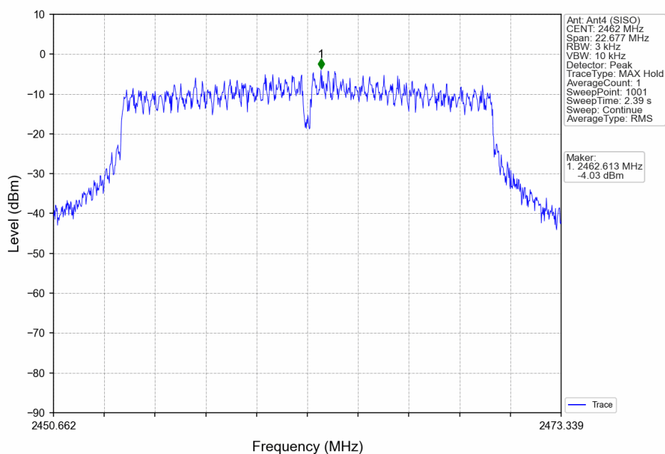
802.11g_HCH_2462MHz_Ant4 (SISO)_NTNV
