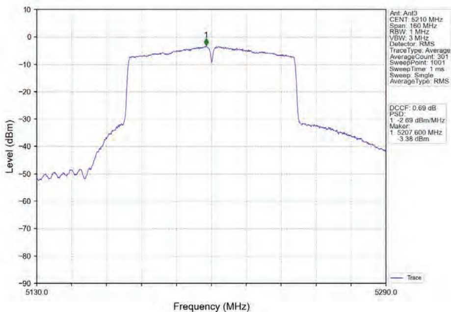
802.11ac(VHT80)_MCH_5210MHz_Ant3_NTNV
