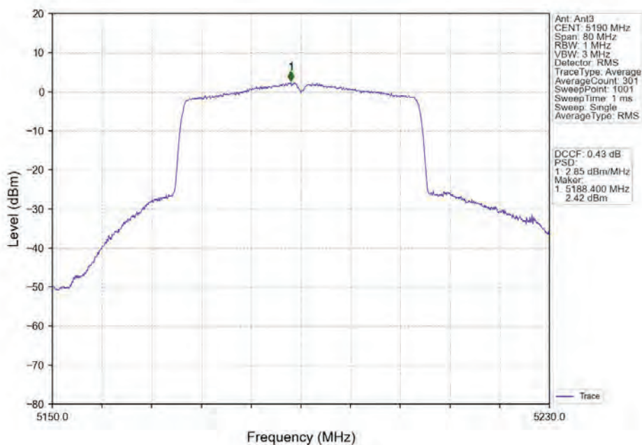
802.11ax(HEW40)_LCH_5190MHz_RU484_Left_Ant3_NTNV
