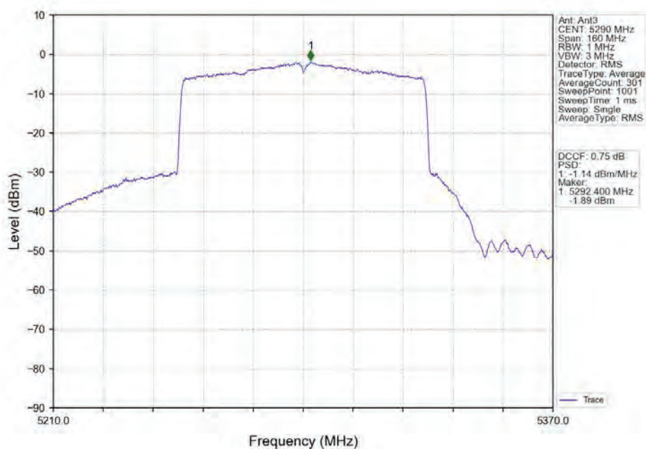
802.11ax(HEW80)_MCH_5290MHz_RU996_Left_Ant3_NTNV
