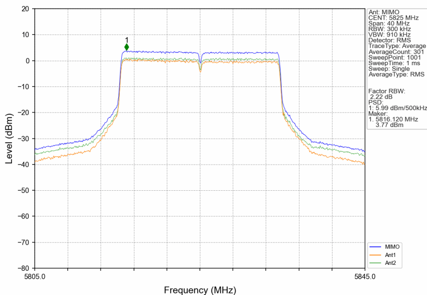
802.11be(EHT20)_HCH_5825MHz_RU242_Left_MIMO_NTNV
