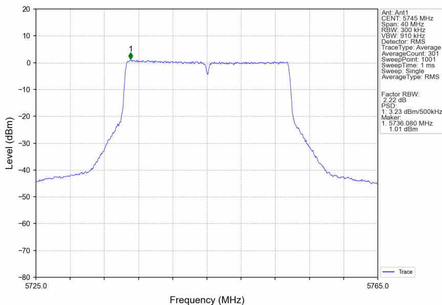
802.11be(EHT20)_LCH_5745MHz_RU242_Left_Ant1_NTNV
