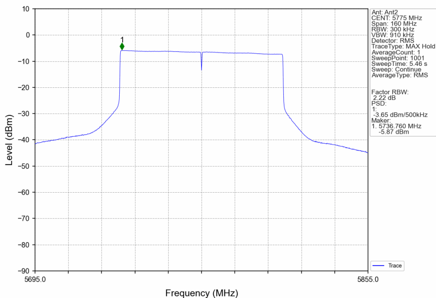
802.11be(EHT80)_MCH_5775MHz_RU996_Left_Ant2_NTNV
