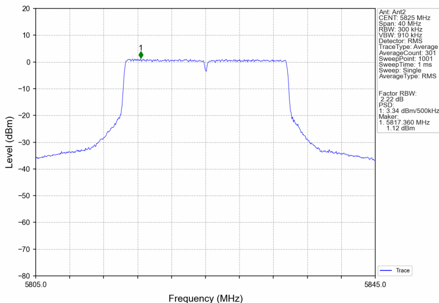
802.11be(EHT20)_HCH_5825MHz_RU242_Left_Ant2_NTNV
