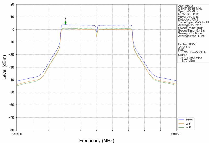
802.11n(HT20)_MCH_5785MHz_MIMO_NTNV
