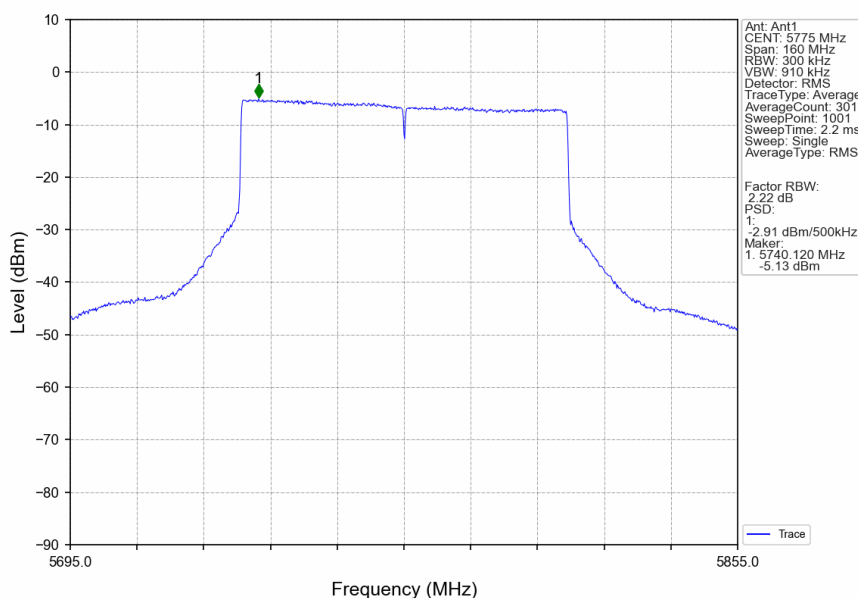
802.11ax(HEW80)_MCH_5775MHz_RU996_Left_Ant1_NTNV
