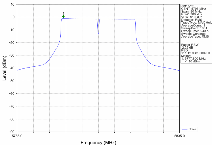
802.11n(HT40)_HCH_5795MHz_Ant2_NTNV
