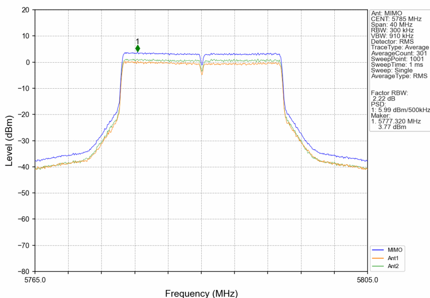
802.11be(EHT20)_MCH_5785MHz_RU242_Left_MIMO_NTNV
