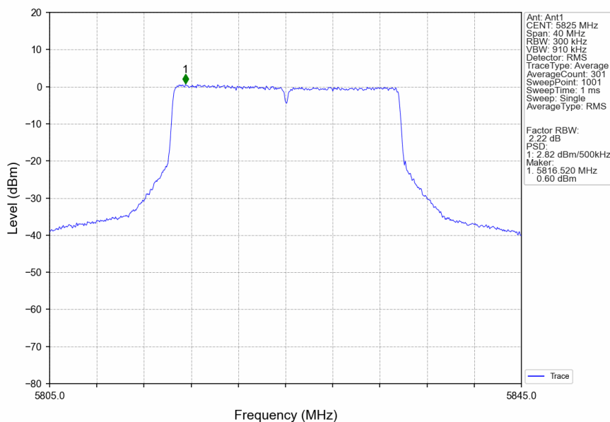
802.11be(EHT20)_HCH_5825MHz_RU242_Left_Ant1_NTNV
