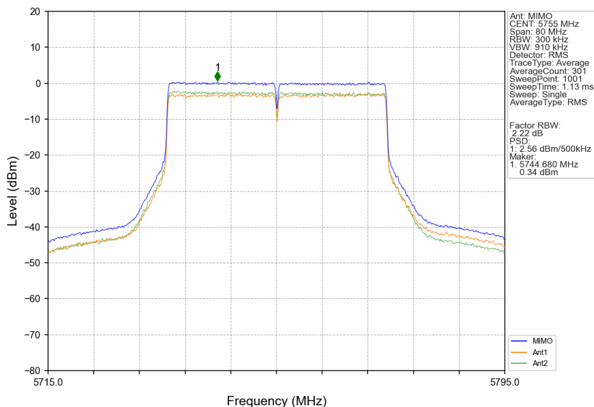
802.11be(EHT40)_LCH_5755MHz_RU484_Left_MIMO_NTNV
