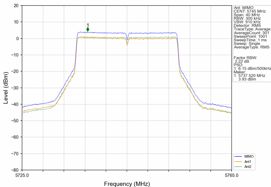
802.11be(EHT20)_LCH_5745MHz_RU242_Left_MIMO_NTNV
