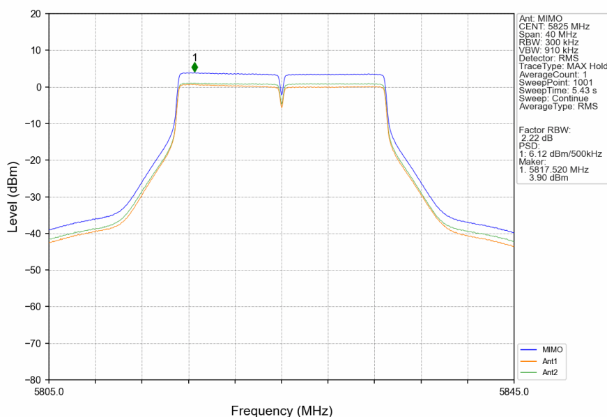
802.11n(HT20)_HCH_5825MHz_MIMO_NTNV
