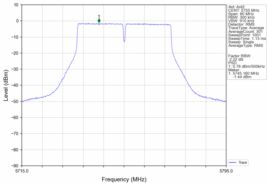
802.11ac(VHT40)_LCH_5755MHz_Ant2_NTNV
