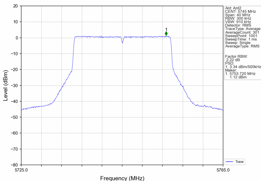
802.11be(EHT20)_LCH_5745MHz_RU242_Left_Ant2_NTNV
