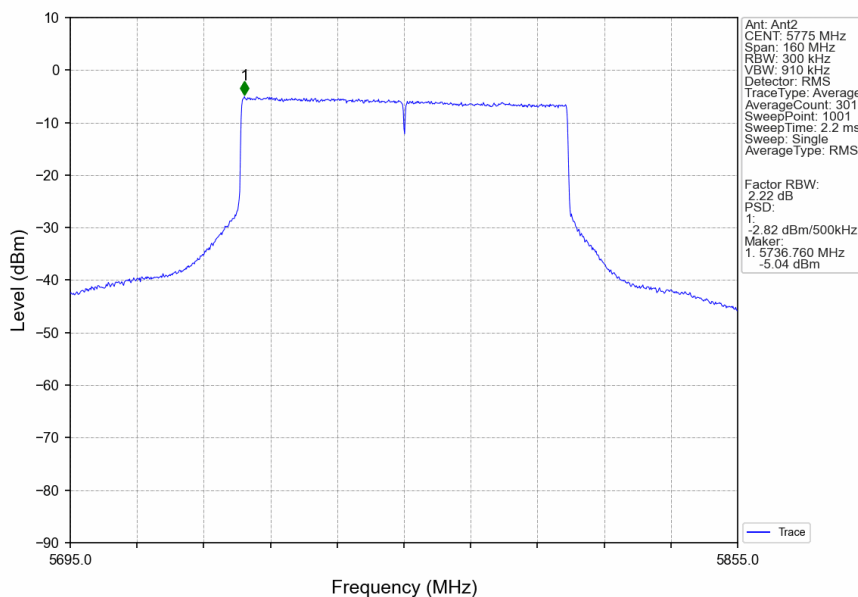
802.11ax(HEW80)_MCH_5775MHz_RU996_Left_Ant2_NTNV
