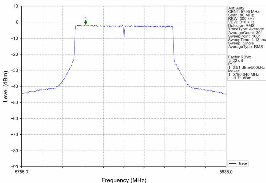
802.11ax(HEW40)_HCH_5795MHz_RU484_Left_Ant2_NTNV
