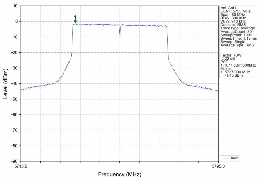
802.11ax(HEW40)_LCH_5755MHz_RU484_Left_Ant1_NTNV
