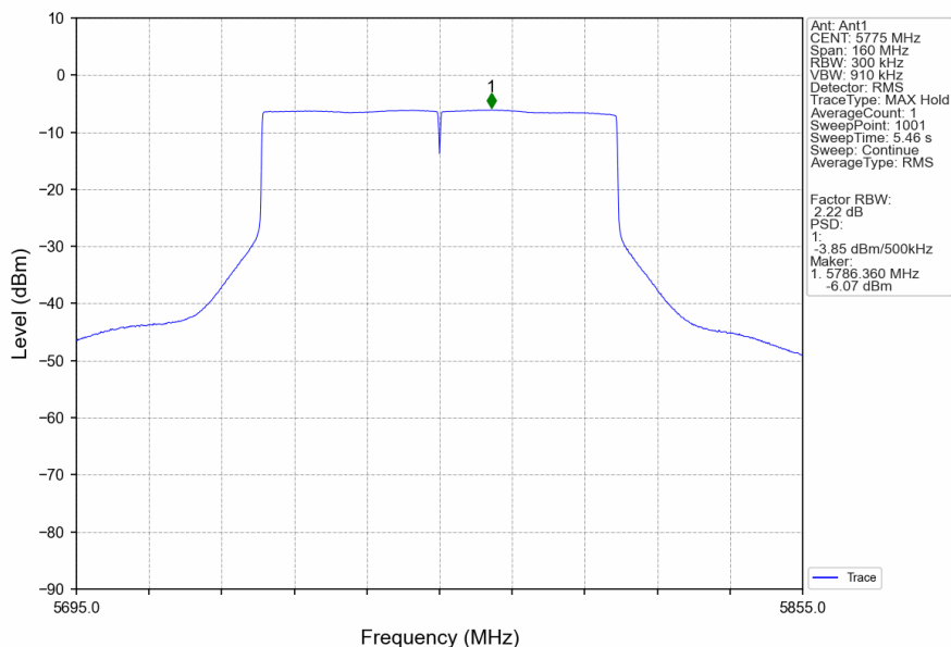
802.11be(EHT80)_MCH_5775MHz_RU996_Left_Ant1_NTNV
