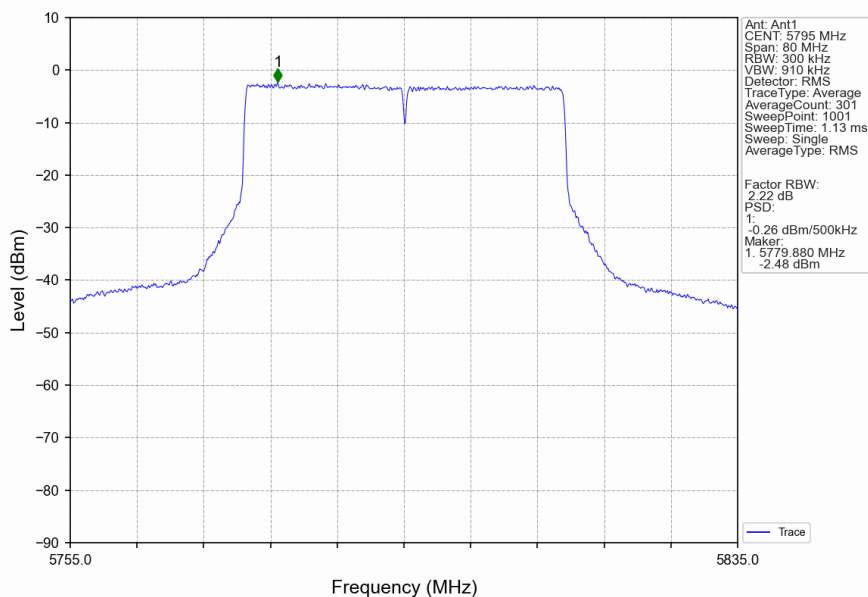
802.11ax(HEW40)_HCH_5795MHz_RU484_Left_Ant1_NTNV
