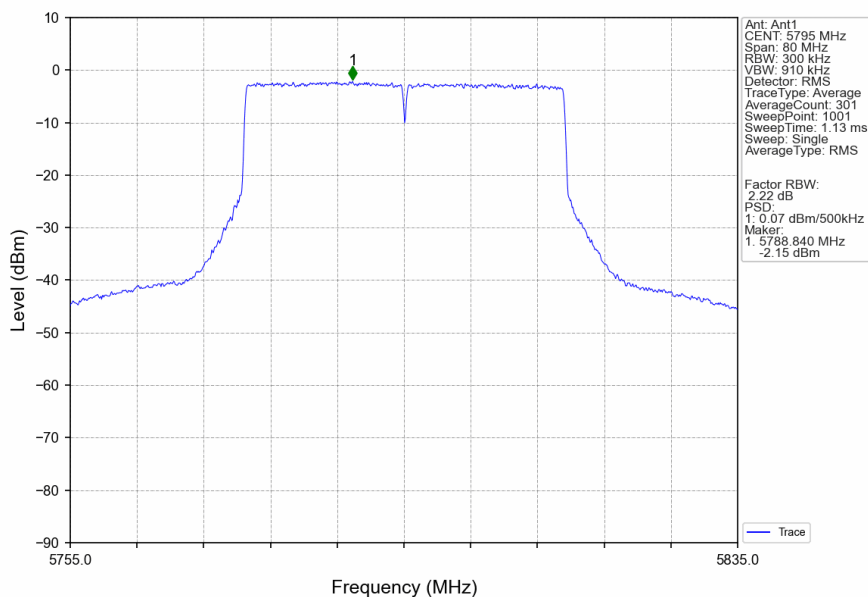
802.11be(EHT40)_HCH_5795MHz_RU484_Left_Ant1_NTNV
