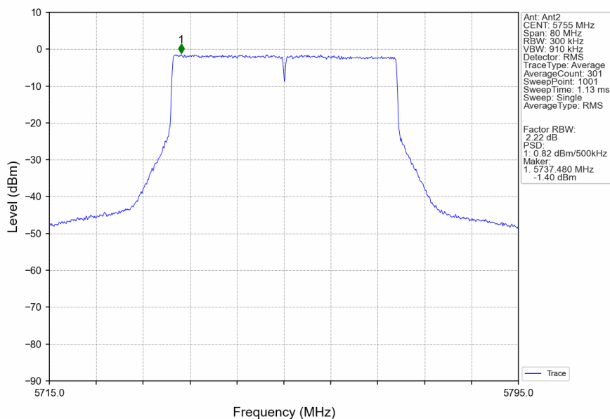
802.11ax(HEW40)_LCH_5755MHz_RU484_Left_Ant2_NTNV
