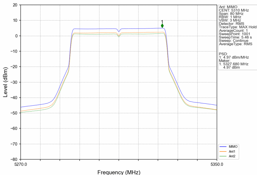
802.11be(EHT40)_HCH_5310MHz_RU484_Left_MIMO_NTNV
