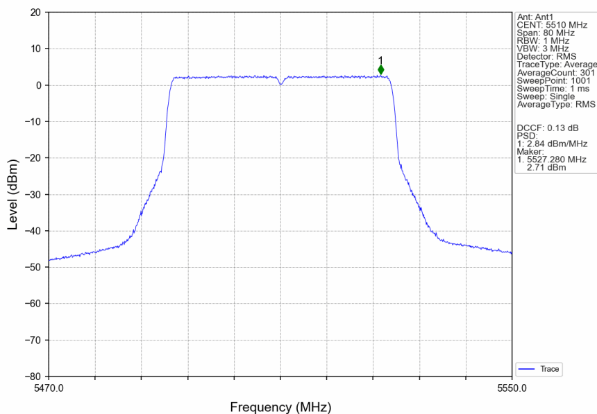
802.11be(EHT40)_LCH_5510MHz_RU484_Left_Ant1_NTNV
