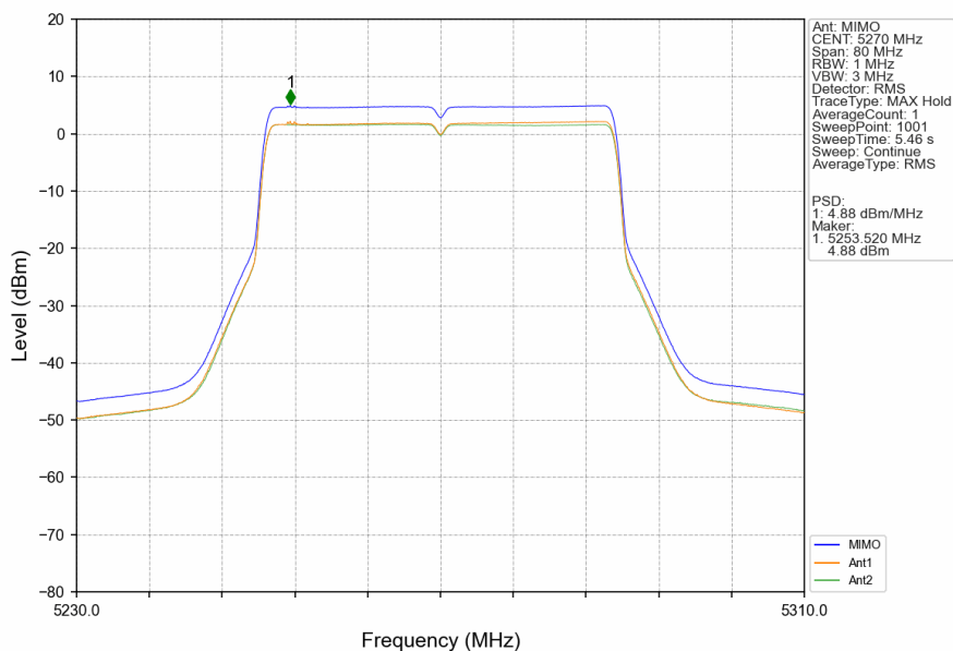
802.11be(EHT40)_LCH_5270MHz_RU484_Left_MIMO_NTNV
