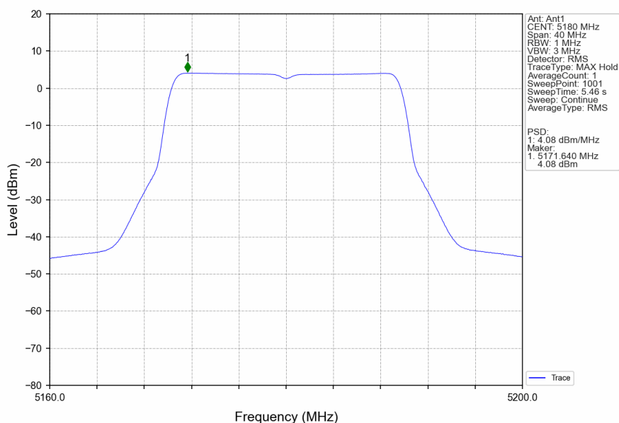
802.11be(EHT20)_LCH_5180MHz_RU242_Left_Ant1_NTNV
