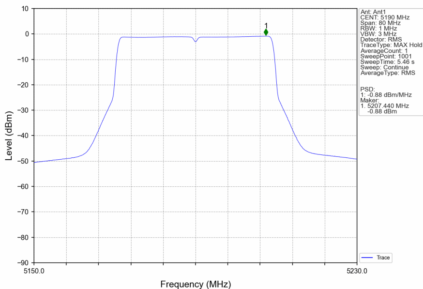
802.11be(EHT40)_LCH_5190MHz_RU484_Left_Ant1_NTNV
