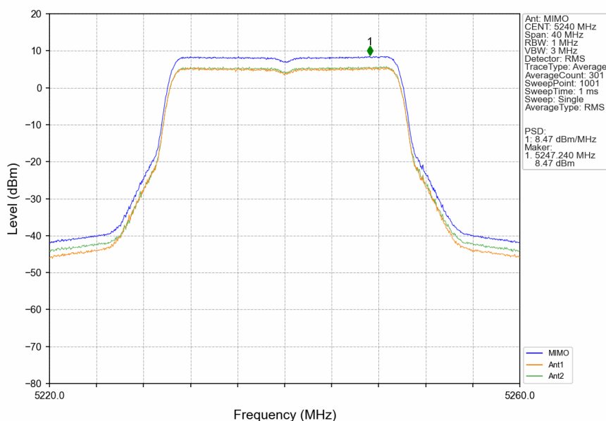
802.11be(EHT20)_HCH_5240MHz_RU242_Left_MIMO_NTNV
