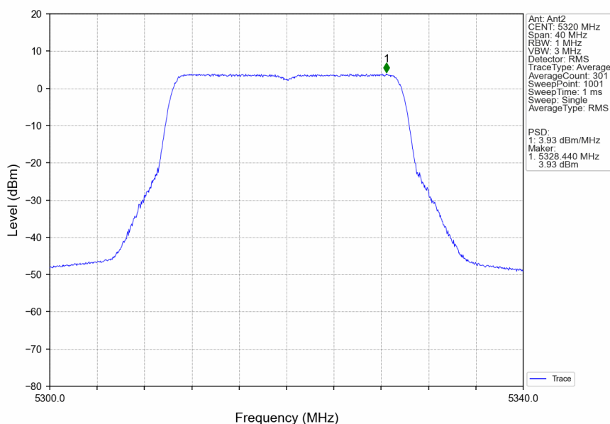
802.11be(EHT20)_HCH_5320MHz_RU242_Left_Ant2_NTNV
