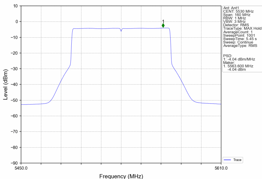
802.11ax(HEW80)_LCH_5530MHz_RU996_Left_Ant1_NTNV
