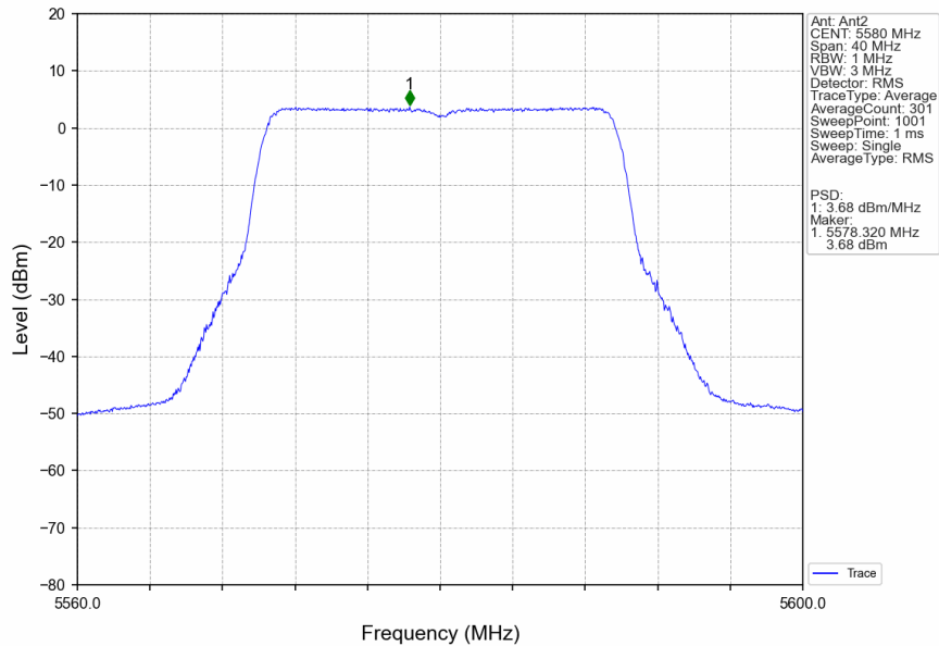
802.11be(EHT20)_MCH_5580MHz_RU242_Left_Ant2_NTNV
