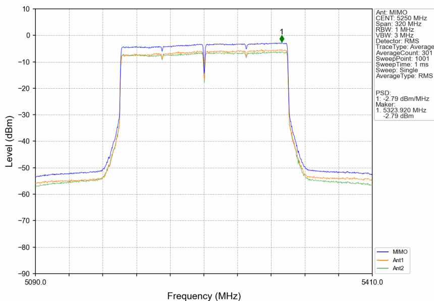
802.11be(EHT160)_MCH_5250MHz_2xRU996_Left_MIMO_NTNV
