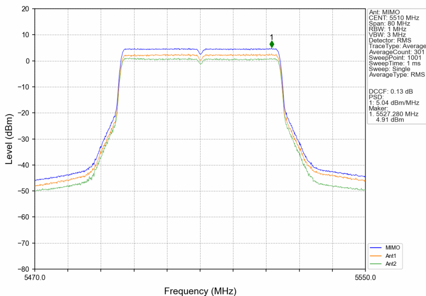
802.11be(EHT40)_LCH_5510MHz_RU484_Left_MIMO_NTNV
