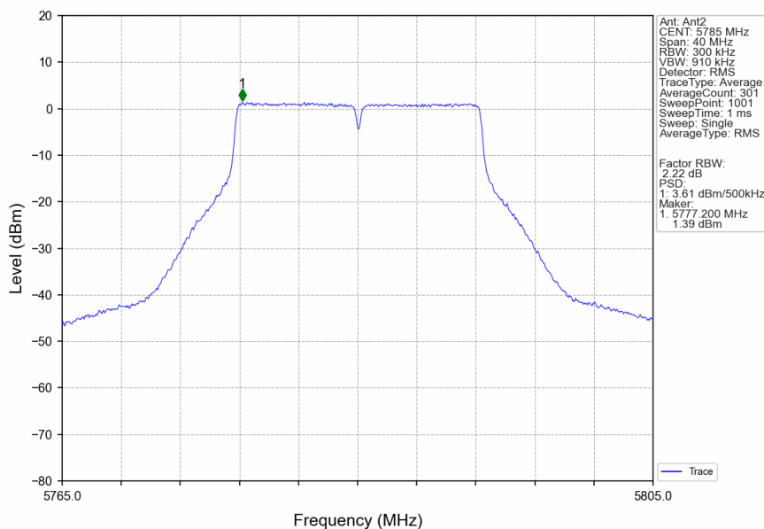
802.11a_MCH_5785MHz_Ant2_NTNV
