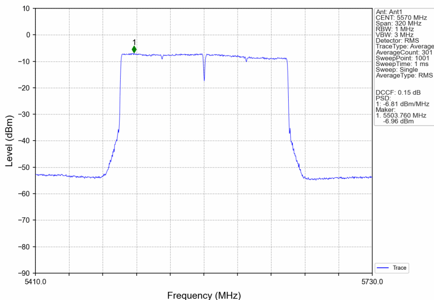
802.11be(EHT160)_MCH_5570MHz_2xRU996_Left_Ant1_NTNV
