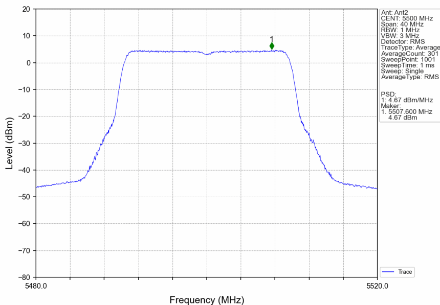
802.11be(EHT20)_LCH_5500MHz_RU242_Left_Ant2_NTNV
