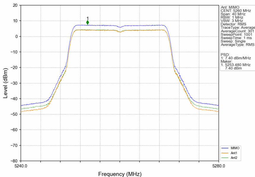
802.11be(EHT20)_LCH_5260MHz_RU242_Left_MIMO_NTNV
