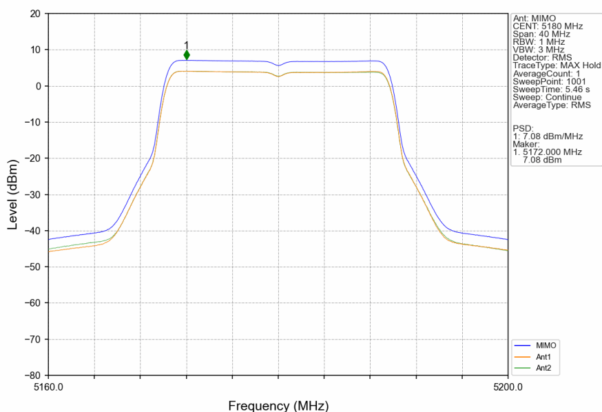
802.11be(EHT20)_LCH_5180MHz_RU242_Left_MIMO_NTNV
