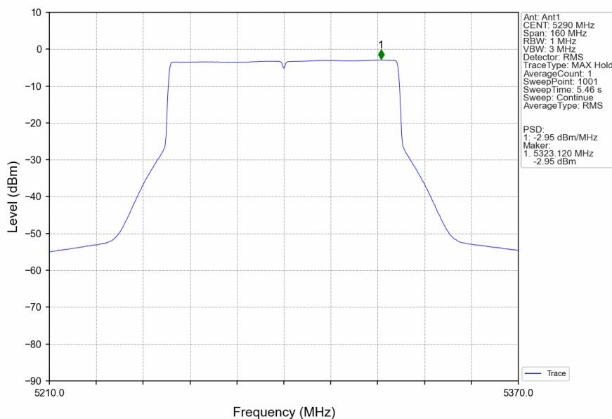
802.11be(EHT80)_MCH_5290MHz_RU996_Left_Ant1_NTNV
