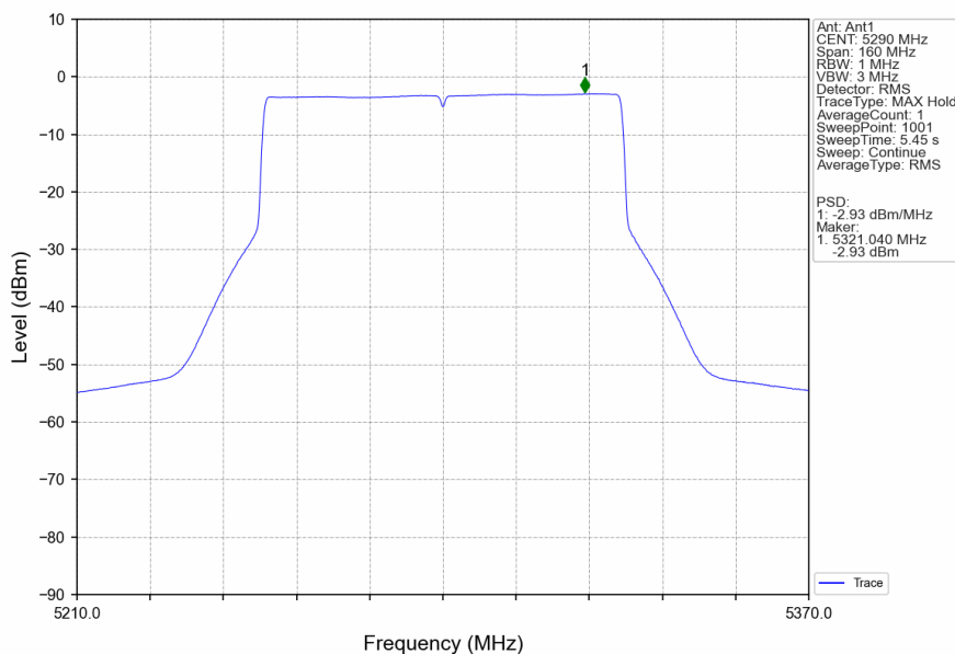
802.11ax(HEW80)_MCH_5290MHz_RU996_Left_Ant1_NTNV
