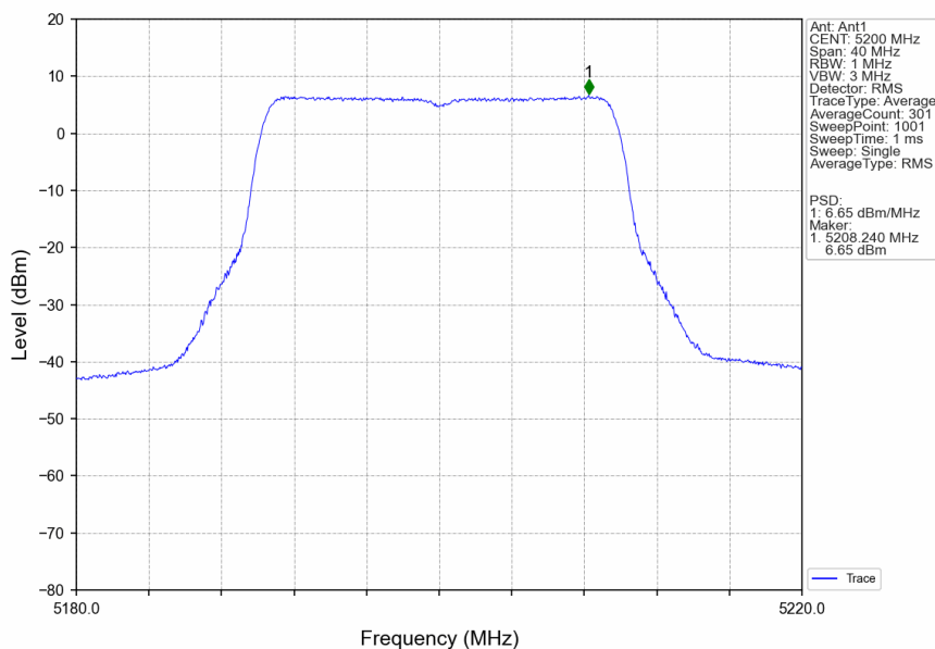
802.11be(EHT20)_MCH_5200MHz_RU242_Left_Ant1_NTNV
