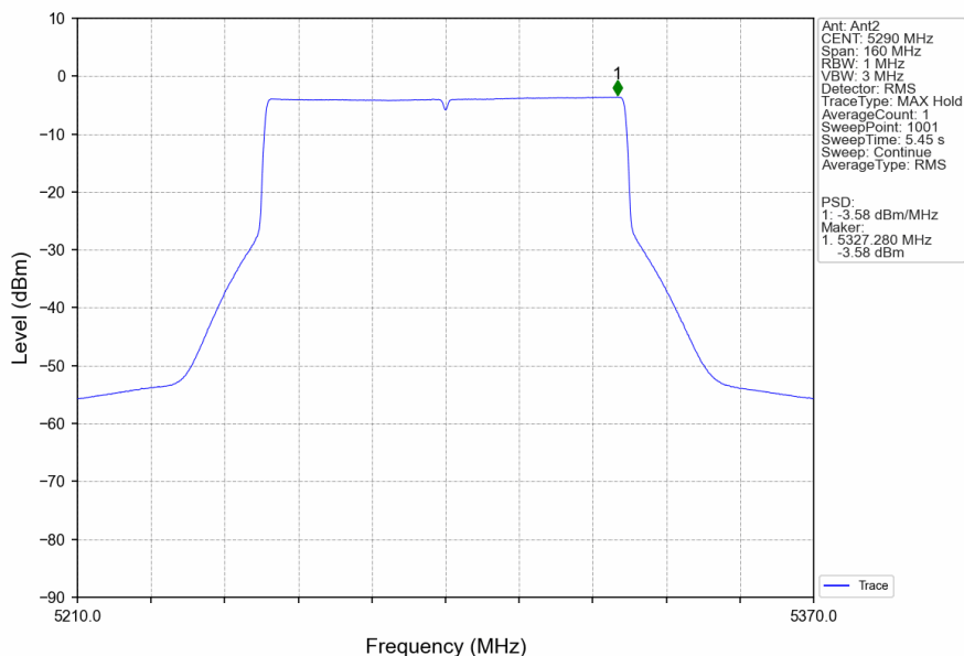
802.11ax(HEW80)_MCH_5290MHz_RU996_Left_Ant2_NTNV
