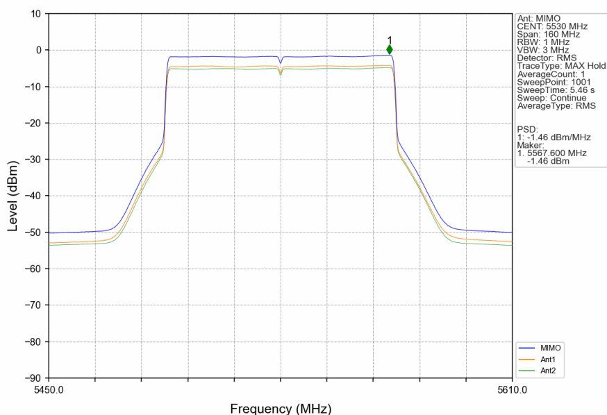
802.11be(EHT80)_LCH_5530MHz_RU996_Left_MIMO_NTNV
