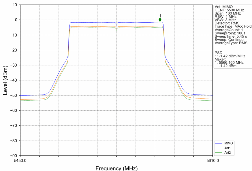
802.11ax(HEW80)_LCH_5530MHz_RU996_Left_MIMO_NTNV
