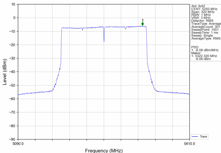
802.11be(EHT160)_MCH_5250MHz_2xRU996_Left_Ant2_NTNV
