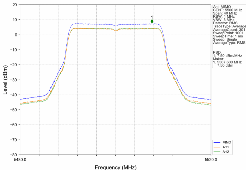
802.11be(EHT20)_LCH_5500MHz_RU242_Left_MIMO_NTNV
