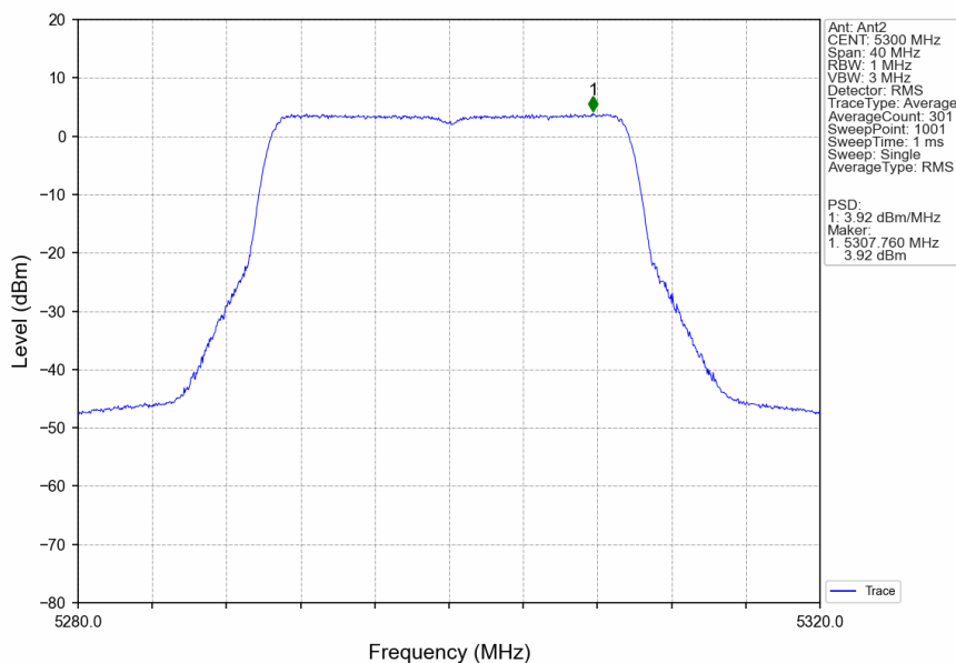
802.11be(EHT20)_MCH_5300MHz_RU242_Left_Ant2_NTNV
