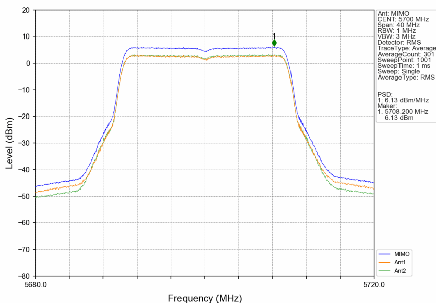
802.11be(EHT20)_HCH_5700MHz_RU242_Left_MIMO_NTNV
