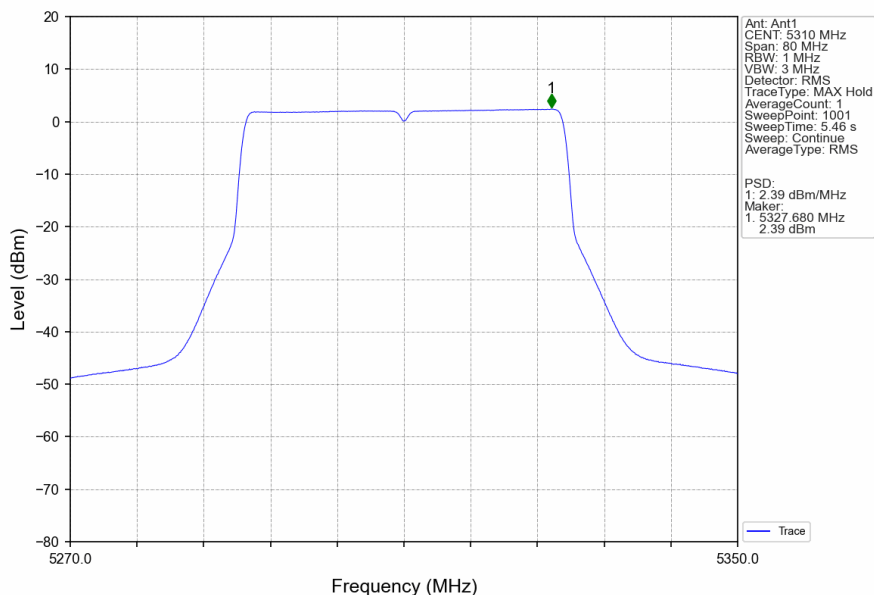
802.11be(EHT40)_HCH_5310MHz_RU484_Left_Ant1_NTNV
