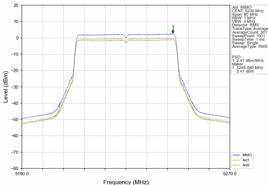
802.11be(EHT40)_HCH_5230MHz_RU484_Left_MIMO_NTNV
