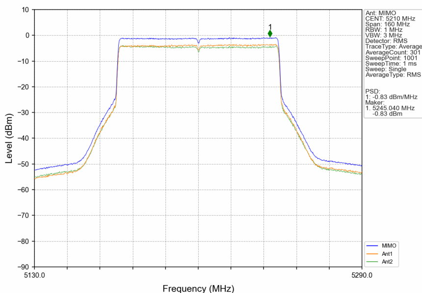
802.11ax(HEW80)_MCH_5210MHz_RU996_Left_MIMO_NTNV
