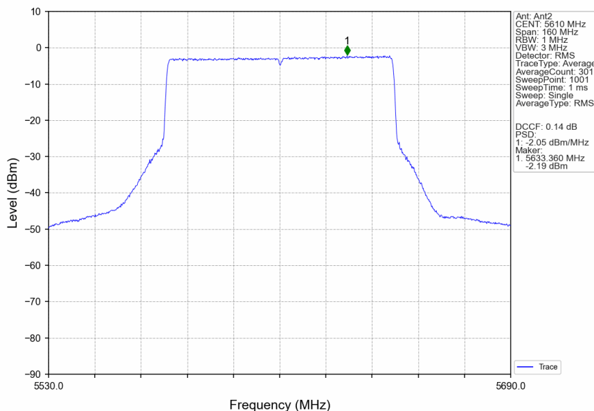
802.11be(EHT80)_HCH_5610MHz_RU996_Left_Ant2_NTNV
