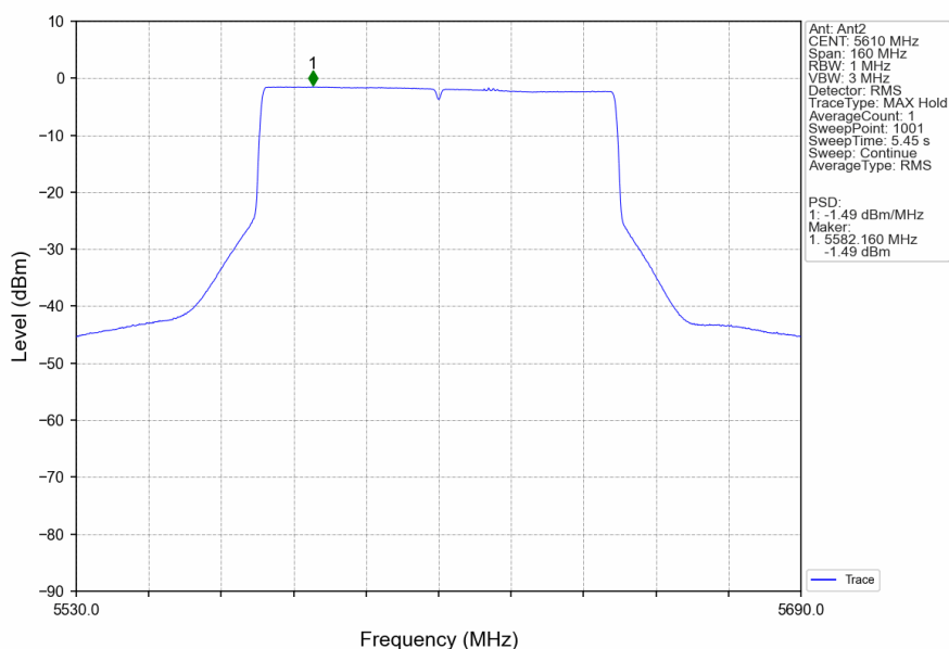
802.11ax(HEW80)_HCH_5610MHz_RU996_Left_Ant2_NTNV
