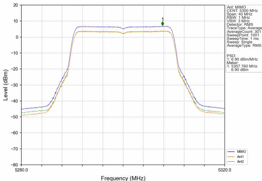
802.11be(EHT20)_MCH_5300MHz_RU242_Left_MIMO_NTNV
