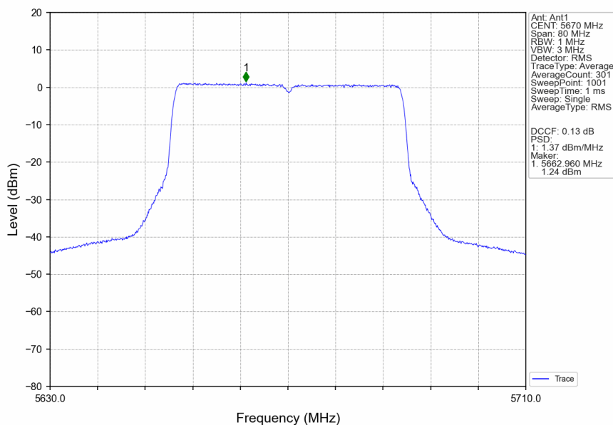
802.11be(EHT40)_HCH_5670MHz_RU484_Left_Ant1_NTNV
