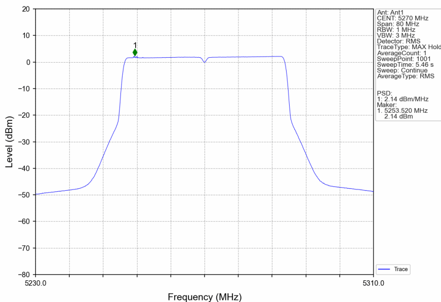
802.11be(EHT40)_LCH_5270MHz_RU484_Left_Ant1_NTNV
