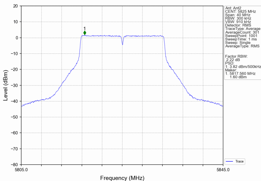
802.11a_HCH_5825MHz_Ant2_NTNV
