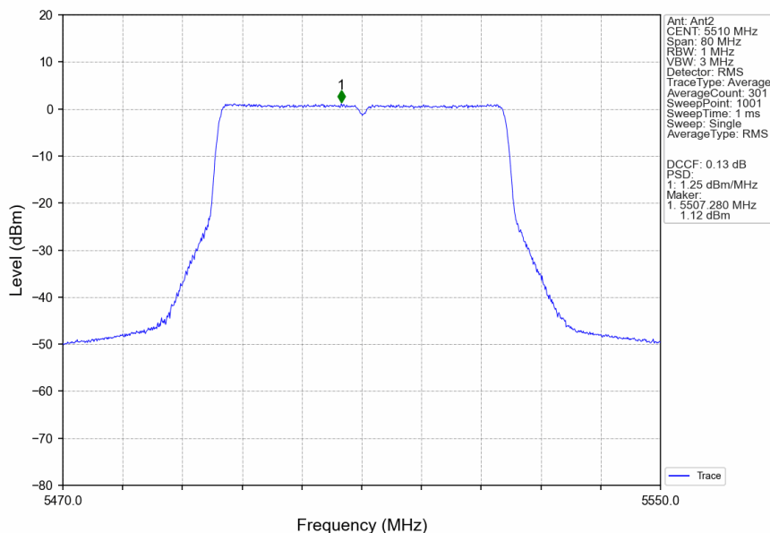
802.11be(EHT40)_LCH_5510MHz_RU484_Left_Ant2_NTNV
