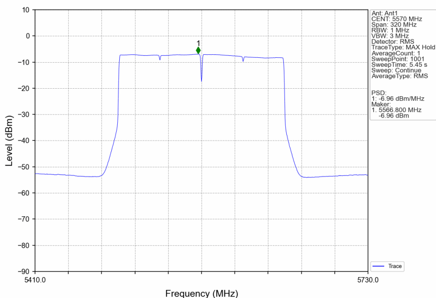
802.11ax(HEW160)_MCH_5570MHz_2xRU996_Left_Ant1_NTNV
