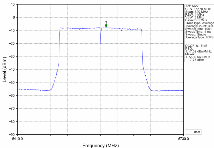
802.11be(EHT160)_MCH_5570MHz_2xRU996_Left_Ant2_NTNV
