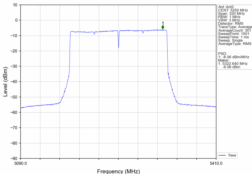
802.11ax(HEW160)_MCH_5250MHz_2xRU996_Left_Ant2_NTNV
