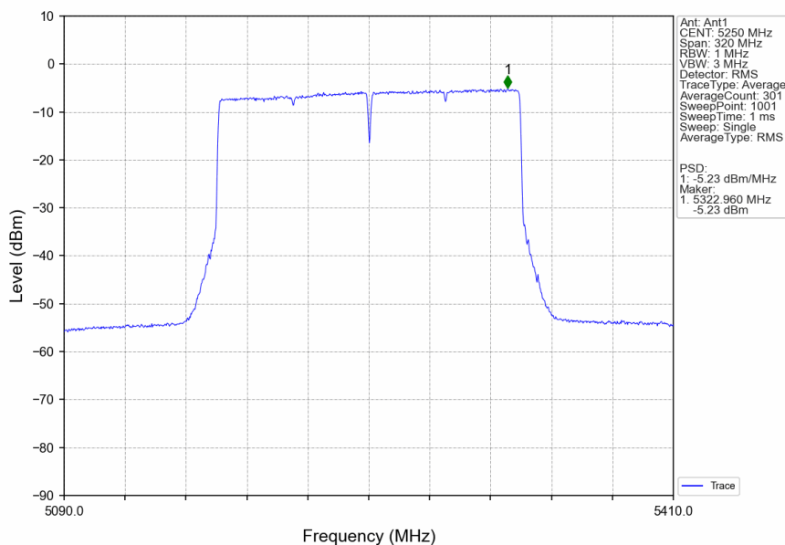
802.11ax(HEW160)_MCH_5250MHz_2xRU996_Left_Ant1_NTNV
