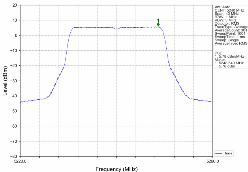
802.11be(EHT20)_HCH_5240MHz_RU242_Left_Ant2_NTNV
