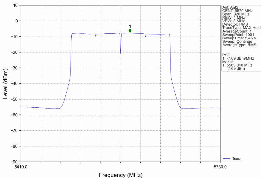
802.11ax(HEW160)_MCH_5570MHz_2xRU996_Left_Ant2_NTNV
