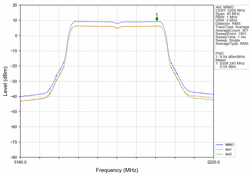
802.11be(EHT20)_MCH_5200MHz_RU242_Left_MIMO_NTNV
