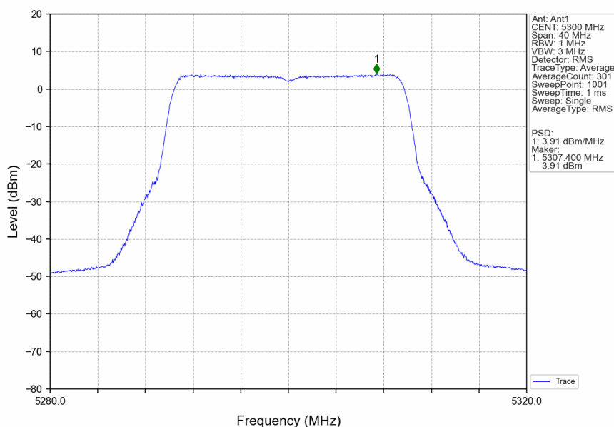
802.11be(EHT20)_MCH_5300MHz_RU242_Left_Ant1_NTNV
