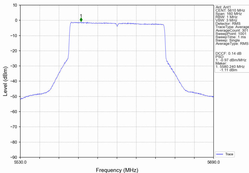
802.11be(EHT80)_HCH_5610MHz_RU996_Left_Ant1_NTNV
