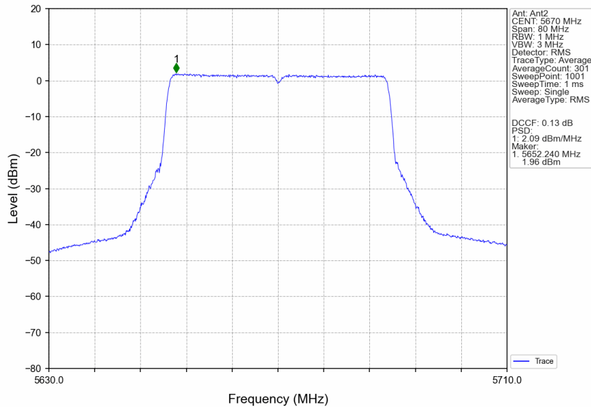
802.11be(EHT40)_HCH_5670MHz_RU484_Left_Ant2_NTNV
