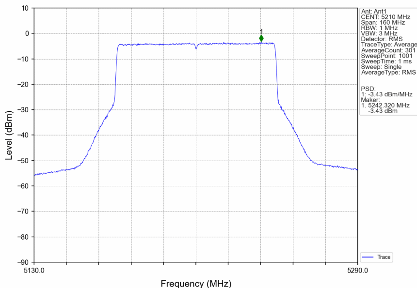
802.11be(EHT80)_MCH_5210MHz_RU996_Left_Ant1_NTNV
