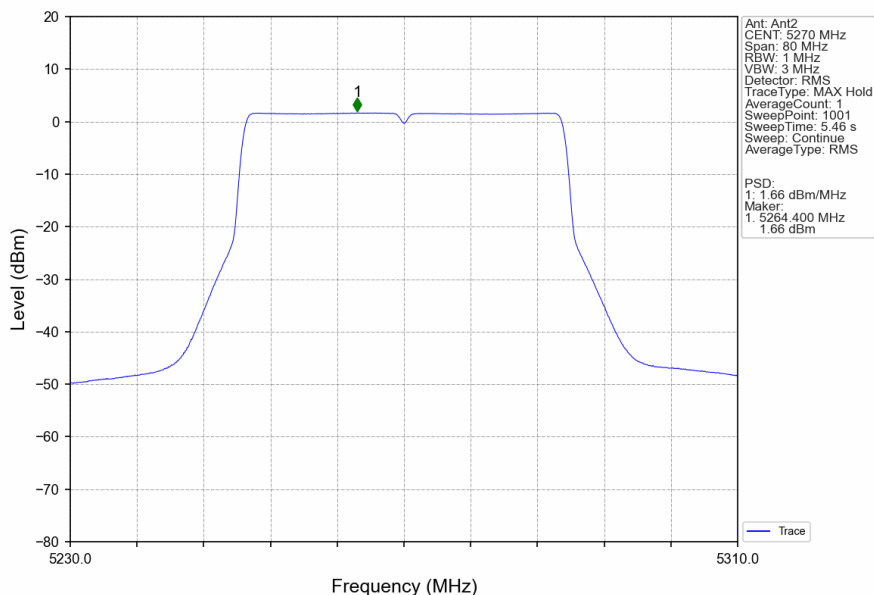
802.11be(EHT40)_LCH_5270MHz_RU484_Left_Ant2_NTNV
