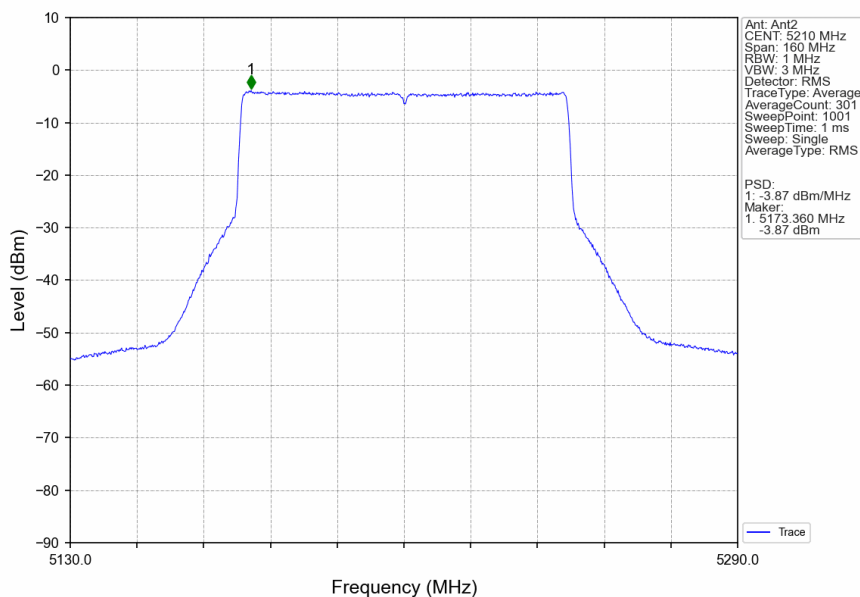
802.11ax(HEW80)_MCH_5210MHz_RU996_Left_Ant2_NTNV
