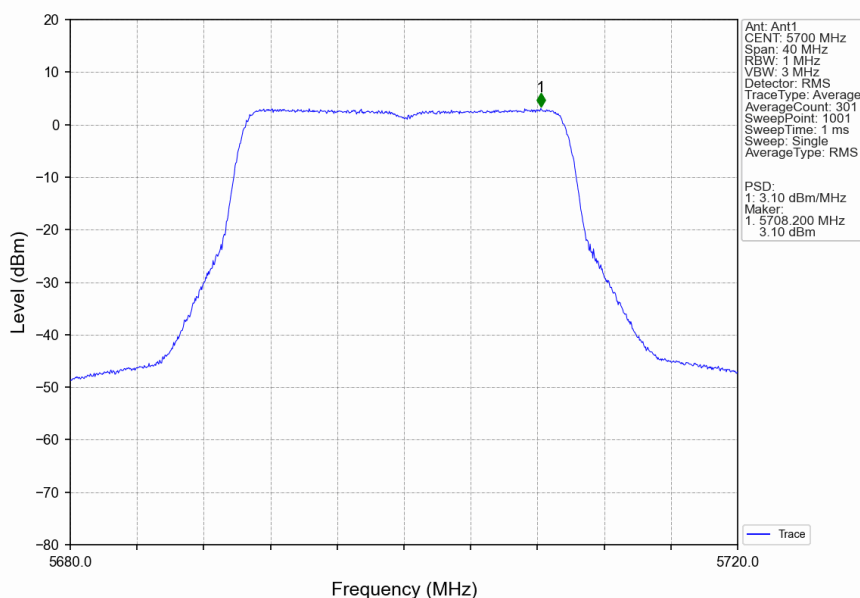
802.11be(EHT20)_HCH_5700MHz_RU242_Left_Ant1_NTNV
