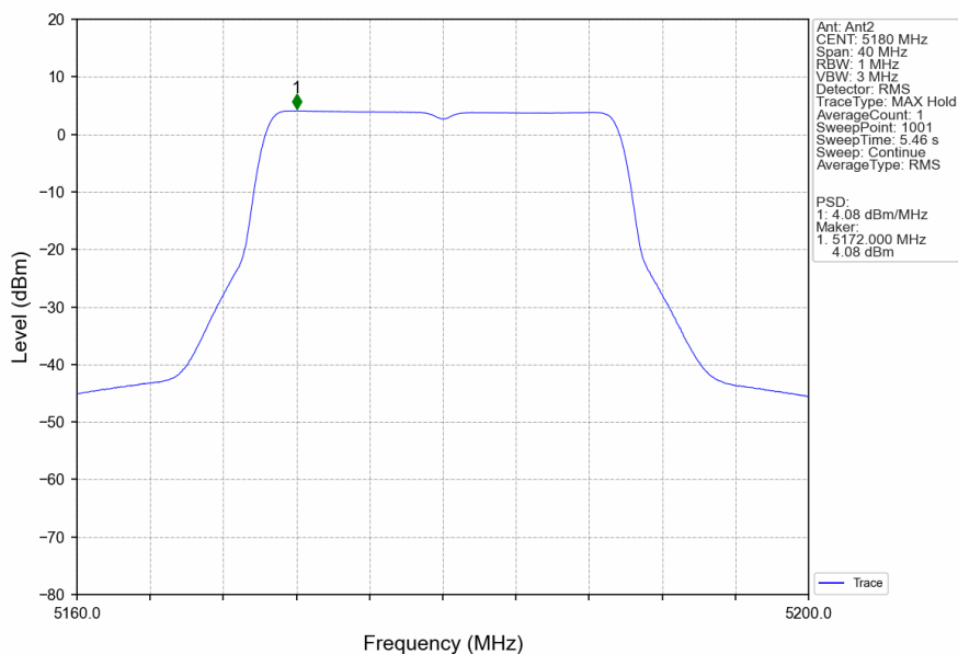
802.11be(EHT20)_LCH_5180MHz_RU242_Left_Ant2_NTNV
