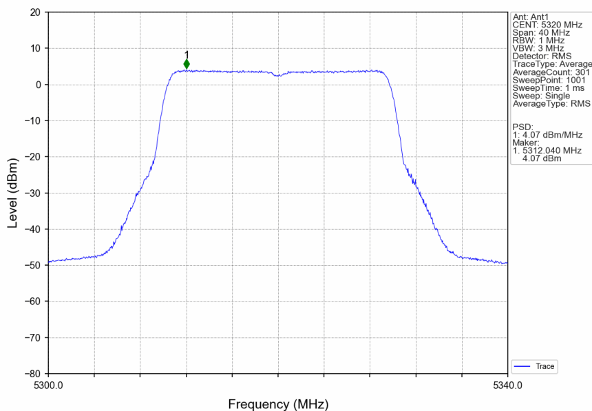
802.11be(EHT20)_HCH_5320MHz_RU242_Left_Ant1_NTNV
