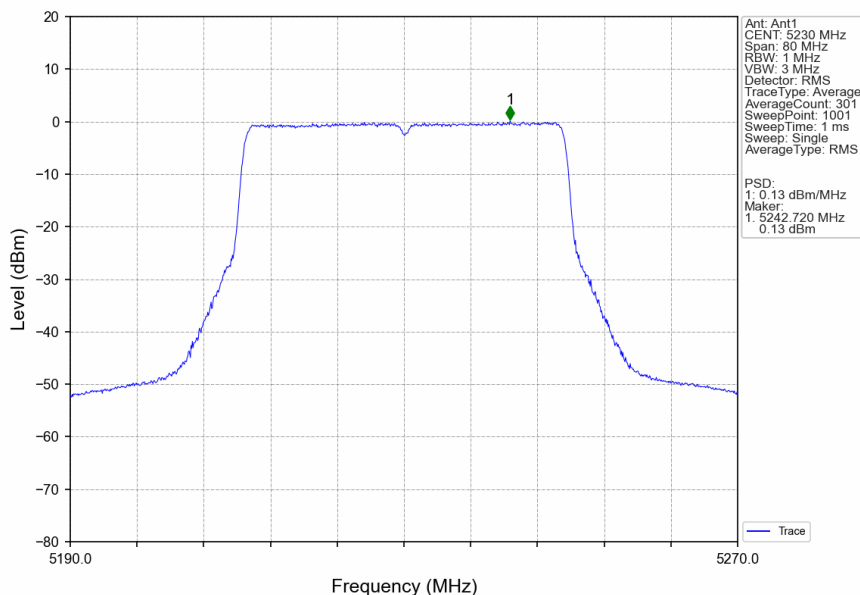
802.11be(EHT40)_HCH_5230MHz_RU484_Left_Ant1_NTNV
