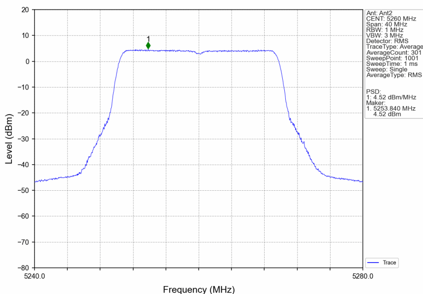
802.11be(EHT20)_LCH_5260MHz_RU242_Left_Ant2_NTNV
