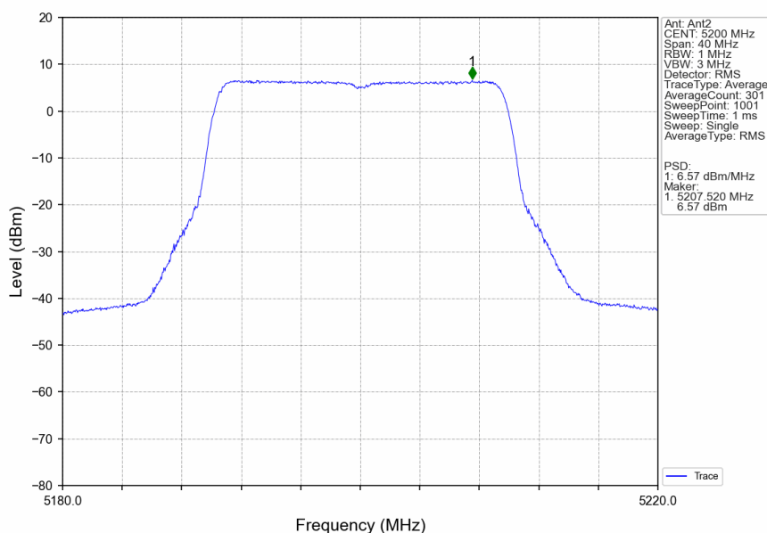
802.11be(EHT20)_MCH_5200MHz_RU242_Left_Ant2_NTNV
