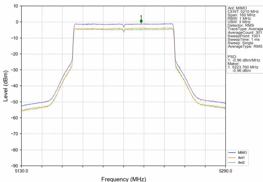
802.11be(EHT80)_MCH_5210MHz_RU996_Left_MIMO_NTNV
