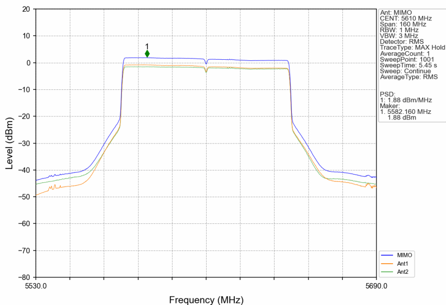
802.11ax(HEW80)_HCH_5610MHz_RU996_Left_MIMO_NTNV
