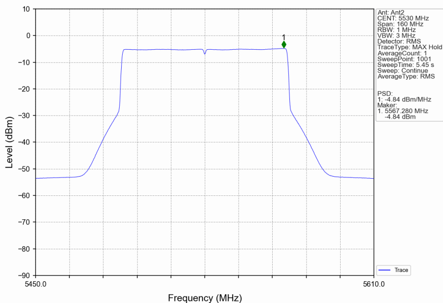
802.11ax(HEW80)_LCH_5530MHz_RU996_Left_Ant2_NTNV
