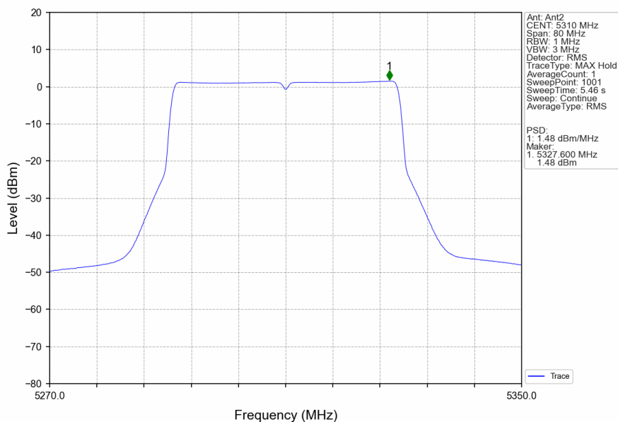
802.11be(EHT40)_HCH_5310MHz_RU484_Left_Ant2_NTNV
