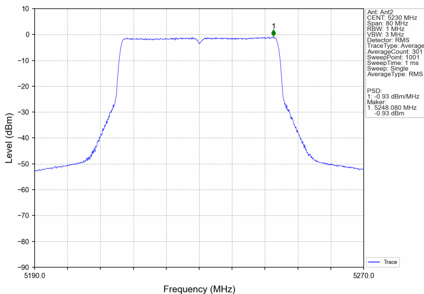
802.11be(EHT40)_HCH_5230MHz_RU484_Left_Ant2_NTNV
