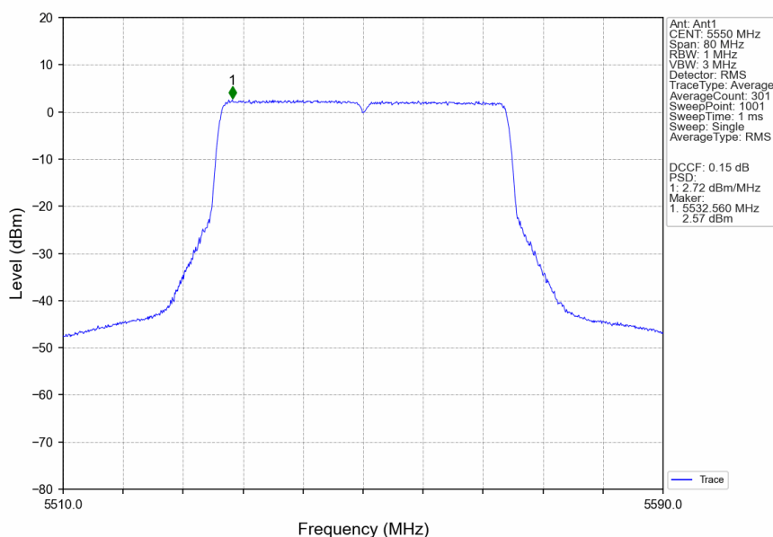
802.11be(EHT40)_MCH_5550MHz_RU484_Left_Ant1_NTNV
