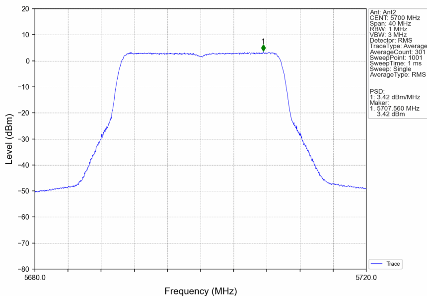
802.11be(EHT20)_HCH_5700MHz_RU242_Left_Ant2_NTNV
