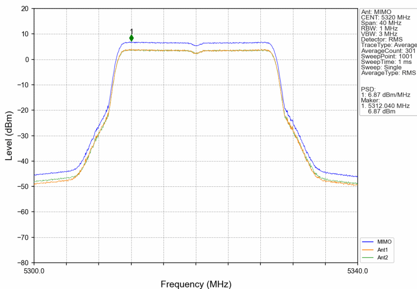
802.11be(EHT20)_HCH_5320MHz_RU242_Left_MIMO_NTNV
