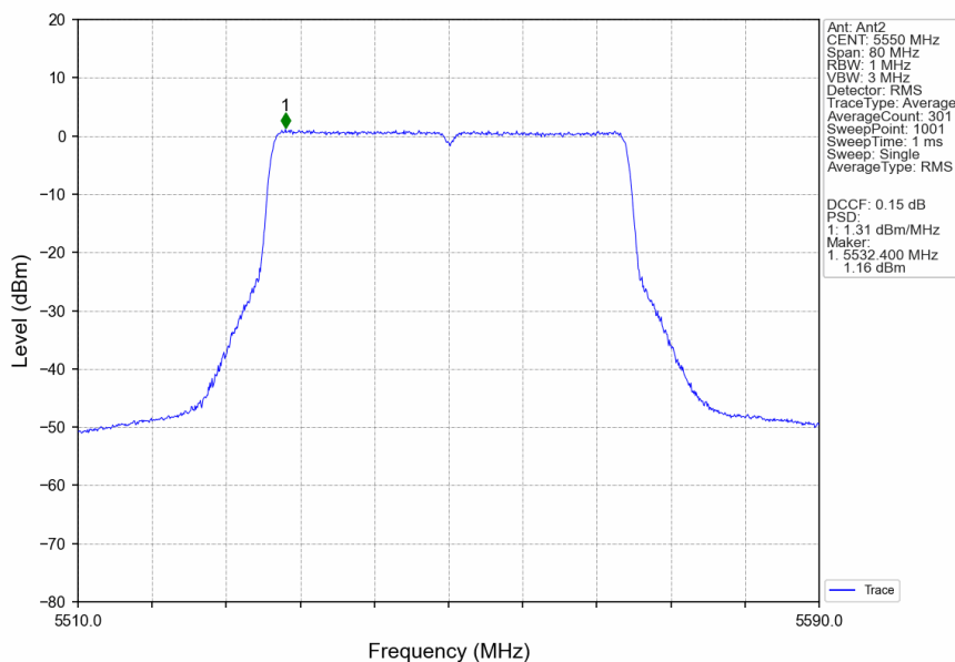
802.11be(EHT40)_MCH_5550MHz_RU484_Left_Ant2_NTNV
