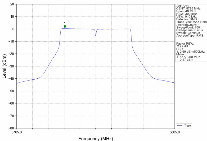
802.11n(HT20)_MCH_5785MHz_Ant1_NTNV
