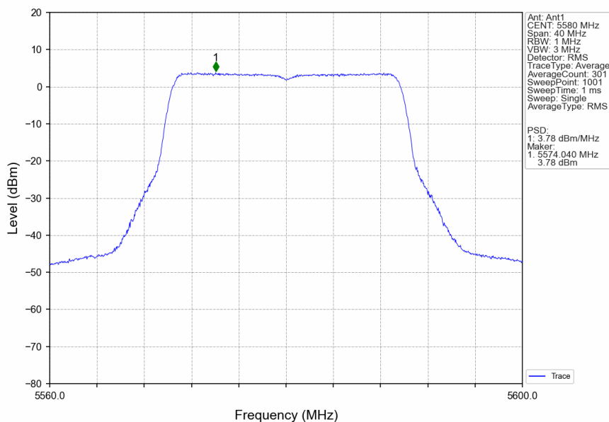
802.11be(EHT20)_MCH_5580MHz_RU242_Left_Ant1_NTNV
