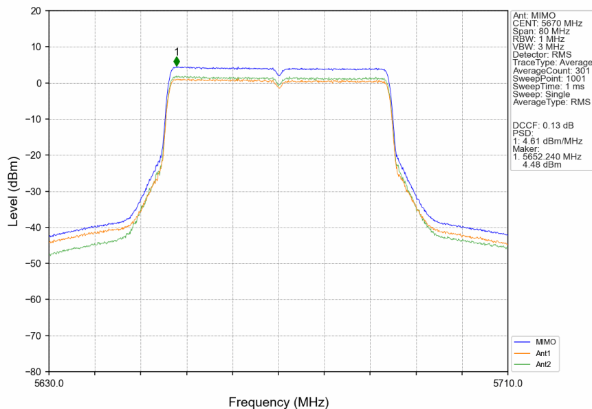
802.11be(EHT40)_HCH_5670MHz_RU484_Left_MIMO_NTNV
