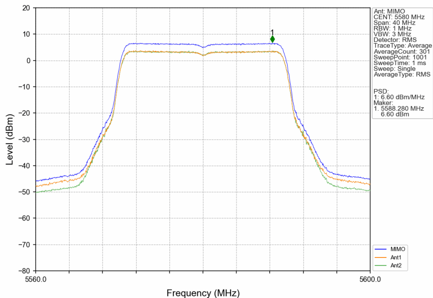
802.11be(EHT20)_MCH_5580MHz_RU242_Left_MIMO_NTNV
