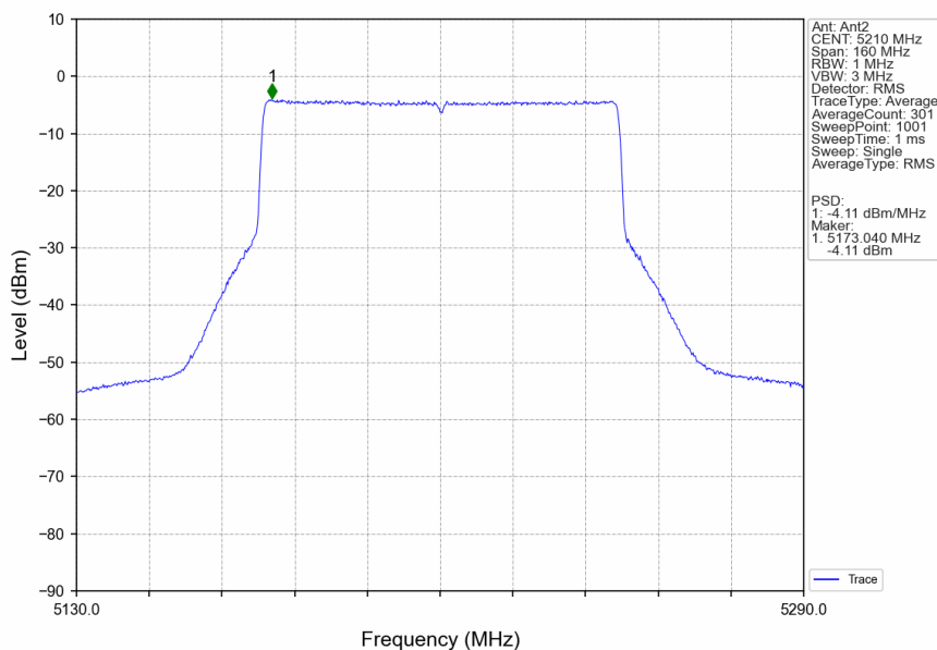
802.11be(EHT80)_MCH_5210MHz_RU996_Left_Ant2_NTNV
