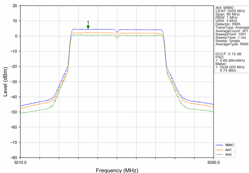
802.11be(EHT40)_MCH_5550MHz_RU484_Left_MIMO_NTNV
