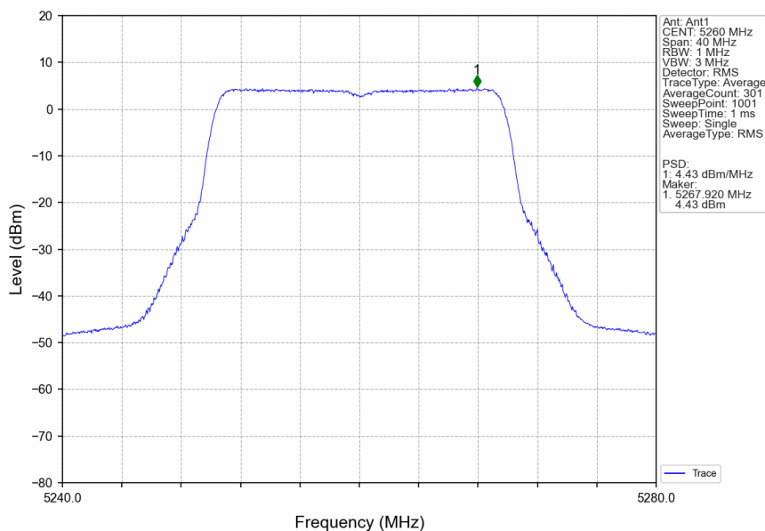
802.11be(EHT20)_LCH_5260MHz_RU242_Left_Ant1_NTNV
