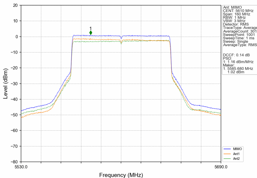
802.11be(EHT80)_HCH_5610MHz_RU996_Left_MIMO_NTNV
