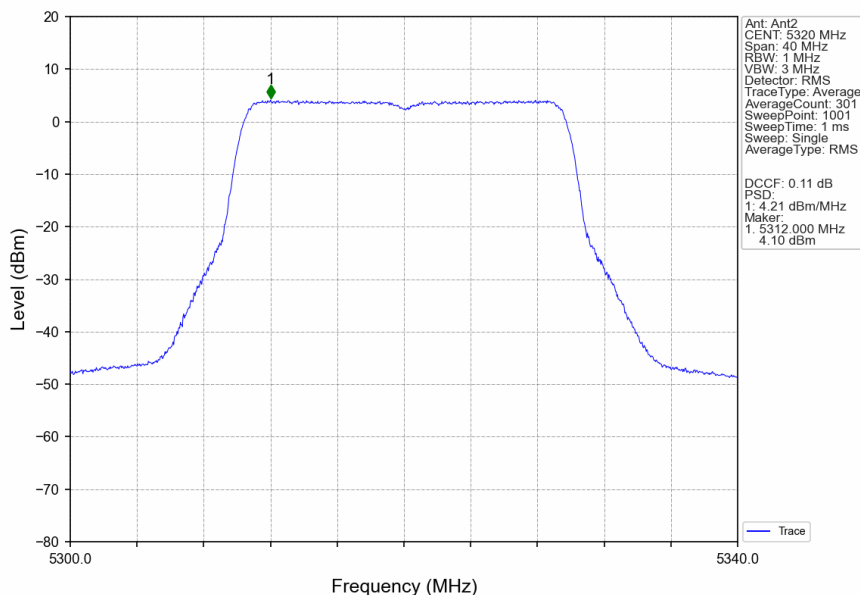
802.11ax(HEW20)_HCH_5320MHz_RU242_Left_Ant2_NTNV
