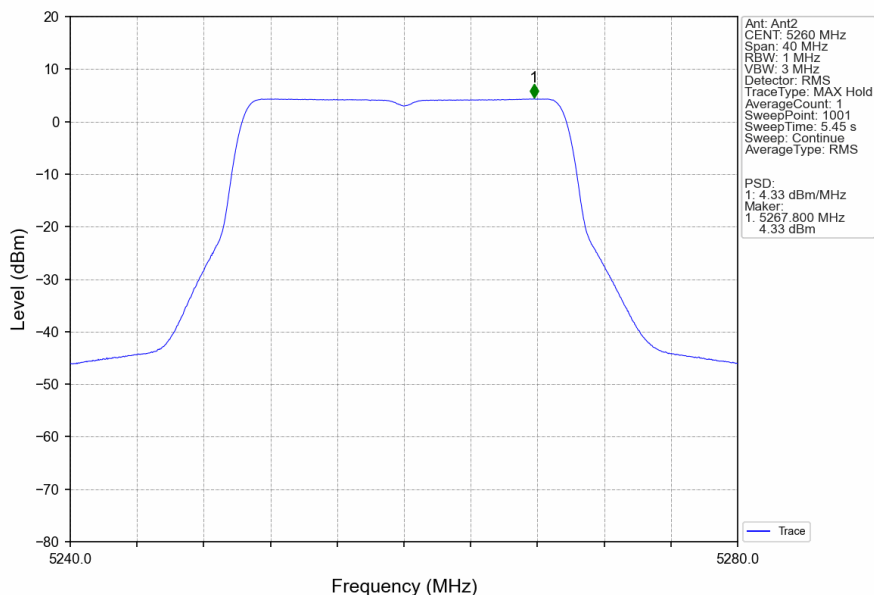
802.11ax(HEW20)_LCH_5260MHz_RU242_Left_Ant2_NTNV
