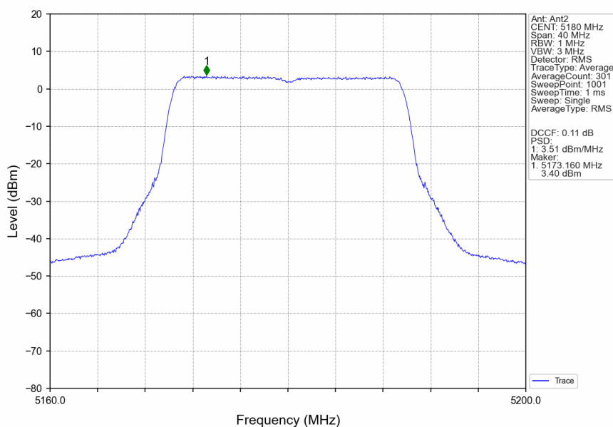
802.11ax(HEW20)_LCH_5180MHz_RU242_Left_Ant2_NTNV
