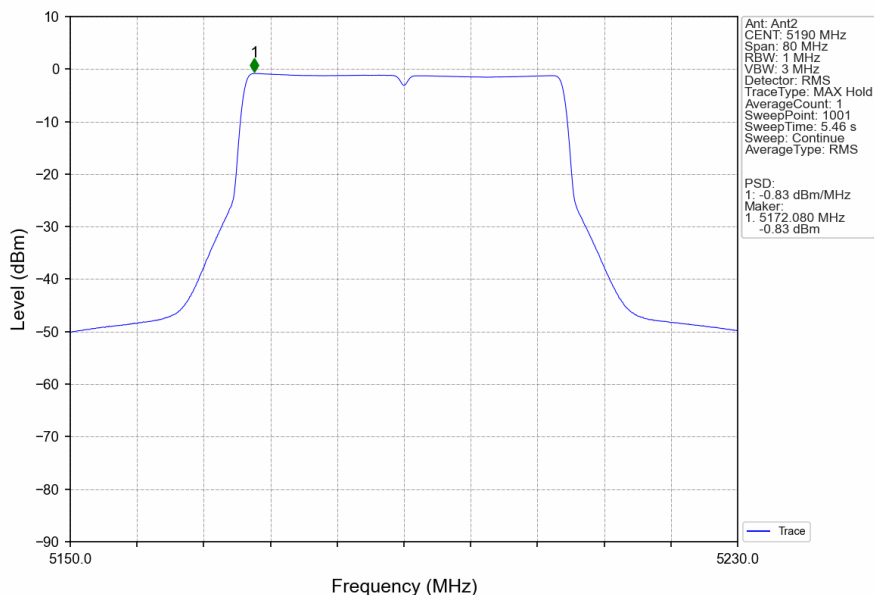
802.11ax(HEW40)_LCH_5190MHz_RU484_Left_Ant2_NTNV
