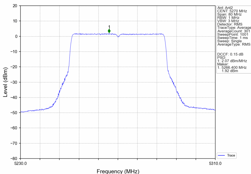
802.11ax(HEW40)_LCH_5270MHz_RU484_Left_Ant2_NTNV
