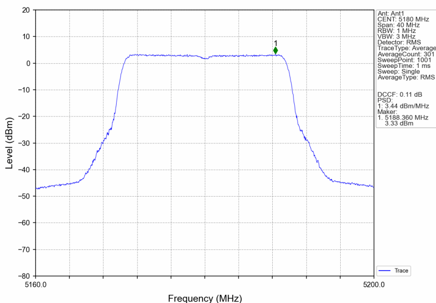
802.11ax(HEW20)_LCH_5180MHz_RU242_Left_Ant1_NTNV
