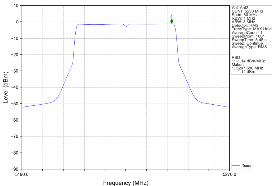
802.11ax(HEW40)_HCH_5230MHz_RU484_Left_Ant2_NTNV
