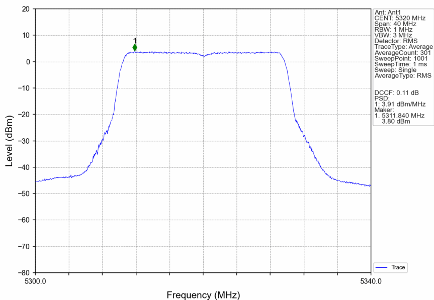
802.11ax(HEW20)_HCH_5320MHz_RU242_Left_Ant1_NTNV
