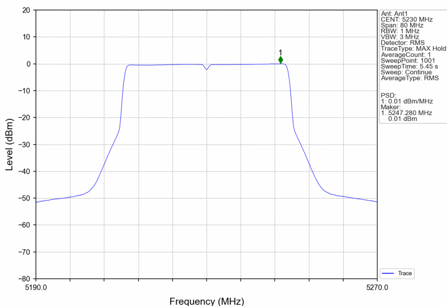
802.11ax(HEW40)_HCH_5230MHz_RU484_Left_Ant1_NTNV
