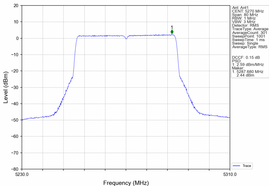
802.11ax(HEW40)_LCH_5270MHz_RU484_Left_Ant1_NTNV
