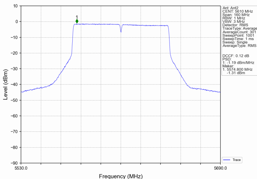
802.11ac(VHT80)_HCH_5610MHz_Ant2_NTNV
