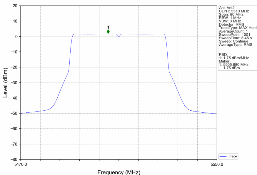
802.11ax(HEW40)_LCH_5510MHz_RU484_Left_Ant2_NTNV
