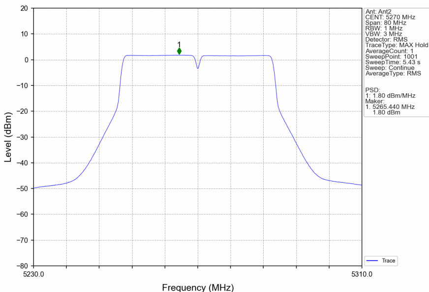
802.11ac(VHT40)_LCH_5270MHz_Ant2_NTNV
