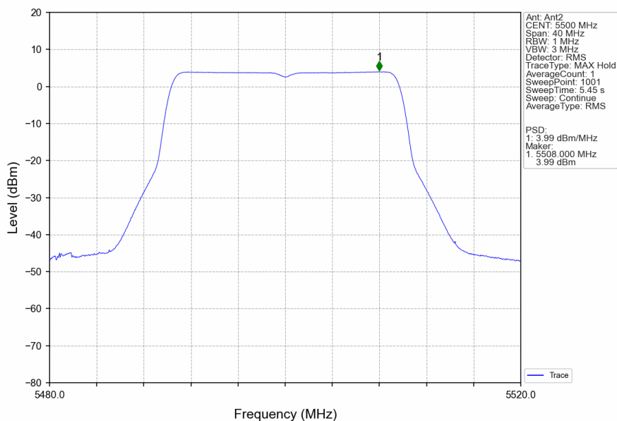
802.11ax(HEW20)_LCH_5500MHz_RU242_Left_Ant2_NTNV
