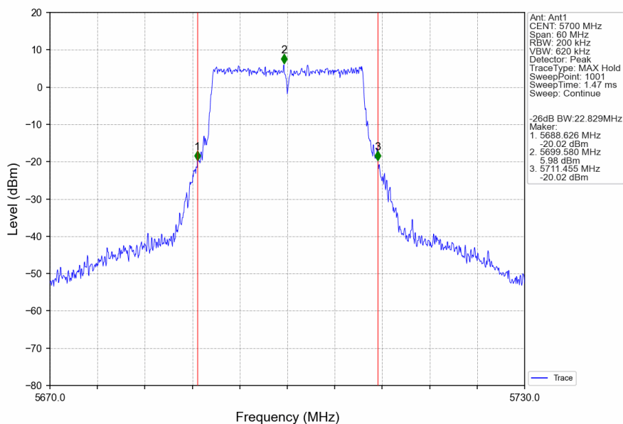
802.11be(EHT20)_HCH_5700MHz_RU242_Left_Ant1_NTNV
