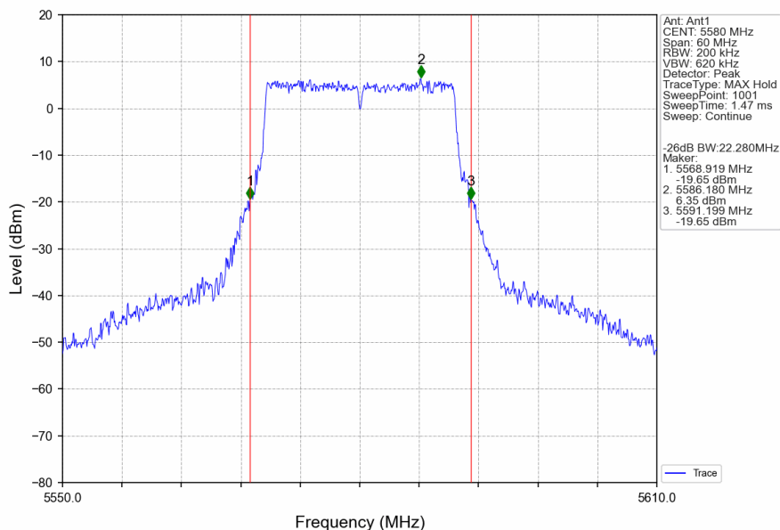
802.11be(EHT20)_MCH_5580MHz_RU242_Left_Ant1_NTNV
