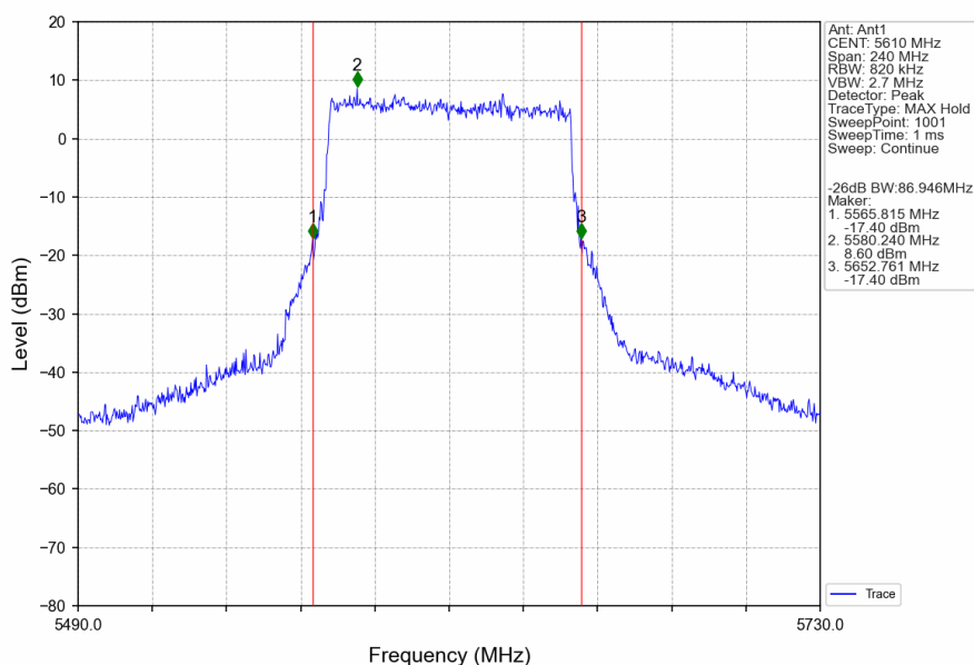
802.11ax(HEW80)_HCH_5610MHz_RU996_Left_Ant1_NTNV
