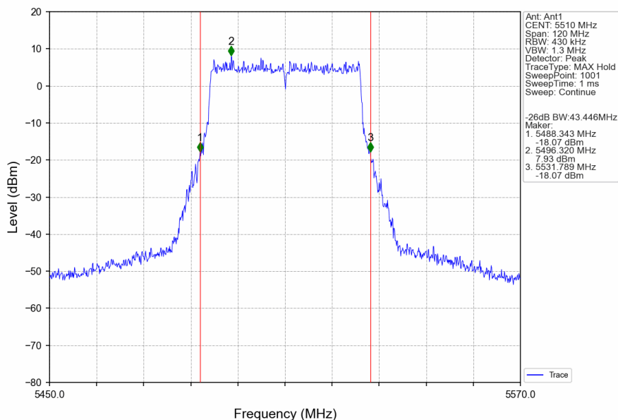
802.11ax(HEW40)_LCH_5510MHz_RU484_Left_Ant1_NTNV
