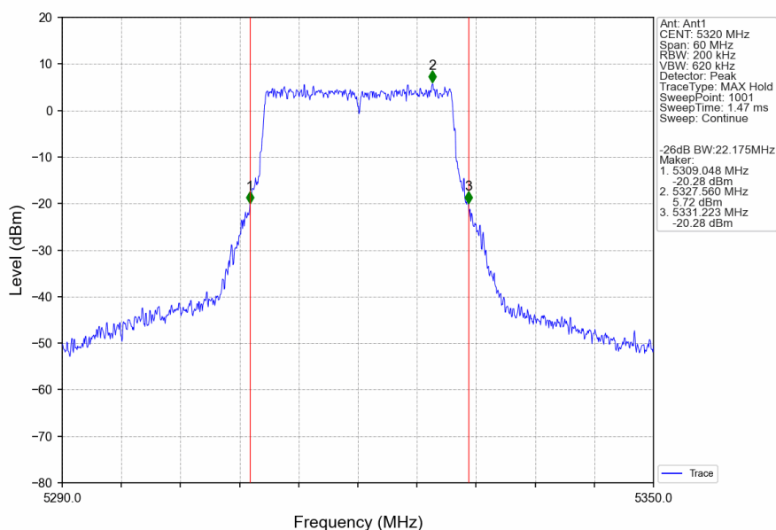
802.11ax(HEW20)_HCH_5320MHz_RU242_Left_Ant1_NTNV
