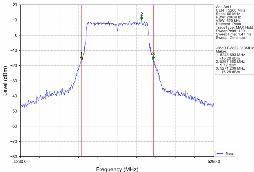
802.11ax(HEW20)_LCH_5260MHz_RU242_Left_Ant1_NTNV
