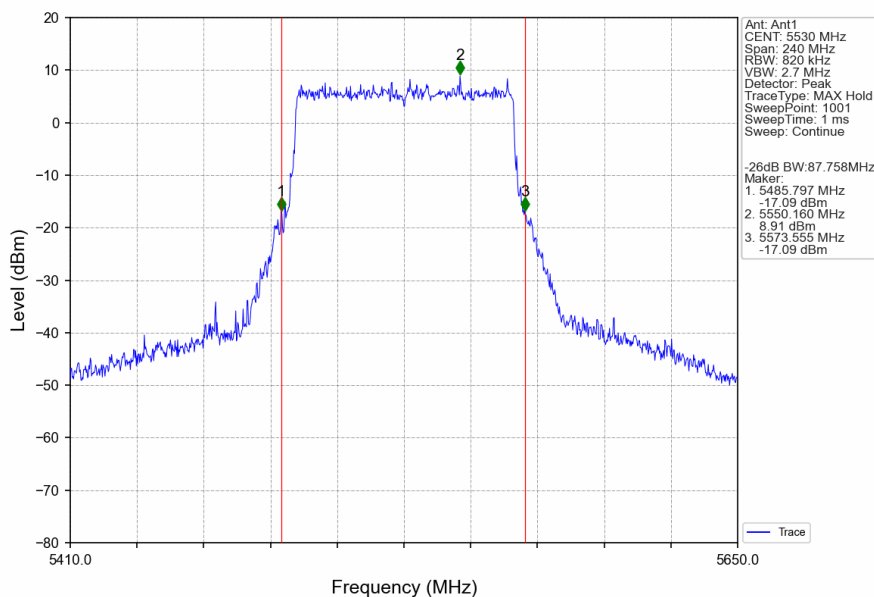
802.11ax(HEW80)_LCH_5530MHz_RU996_Left_Ant1_NTNV
