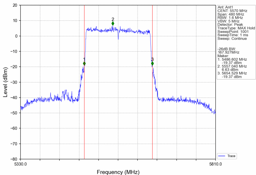
802.11ax(HEW160)_MCH_5570MHz_2xRU996_Left_Ant1_NTNV
