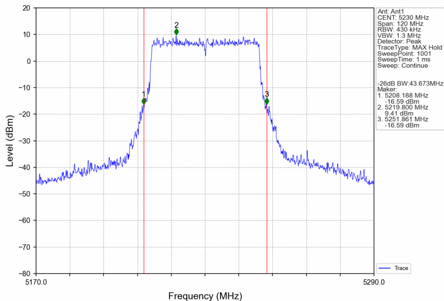
802.11ax(HEW40)_HCH_5230MHz_RU484_Left_Ant1_NTNV
