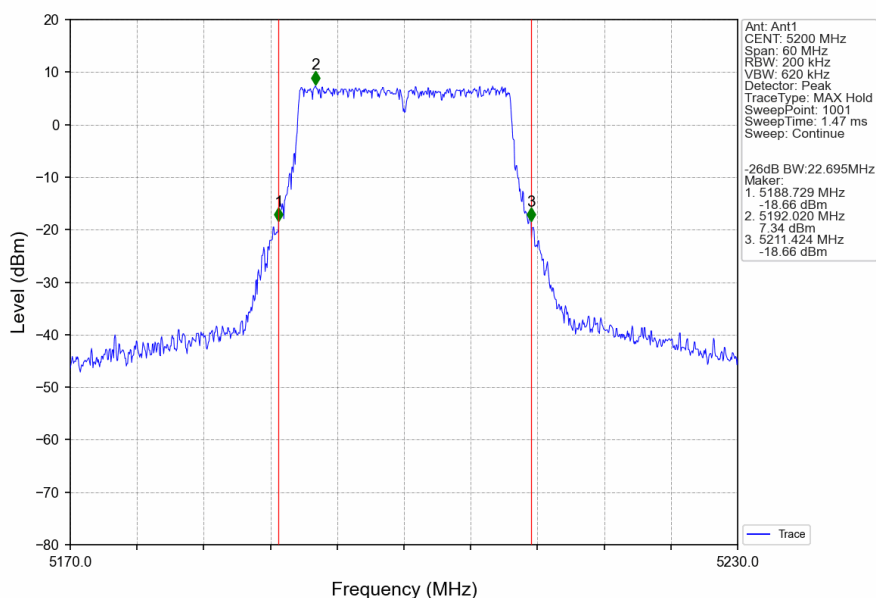
802.11be(EHT20)_MCH_5200MHz_RU242_Left_Ant1_NTNV
