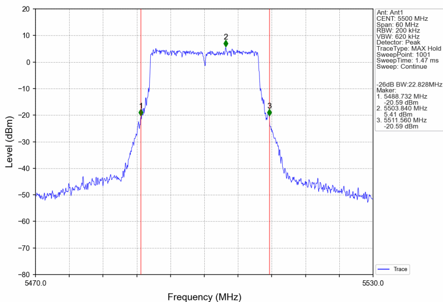
802.11ax(HEW20)_LCH_5500MHz_RU242_Left_Ant1_NTNV
