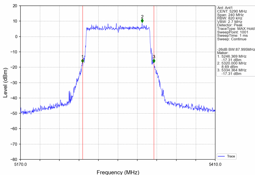
802.11ax(HEW80)_MCH_5290MHz_RU996_Left_Ant1_NTNV
