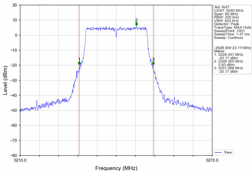
802.11be(EHT20)_HCH_5240MHz_RU242_Left_Ant1_NTNV
