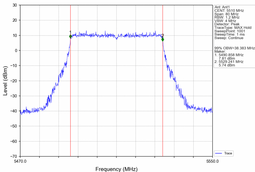
802.11ax(HEW40)_LCH_5510MHz_RU484_Left_Ant1_NTNV
