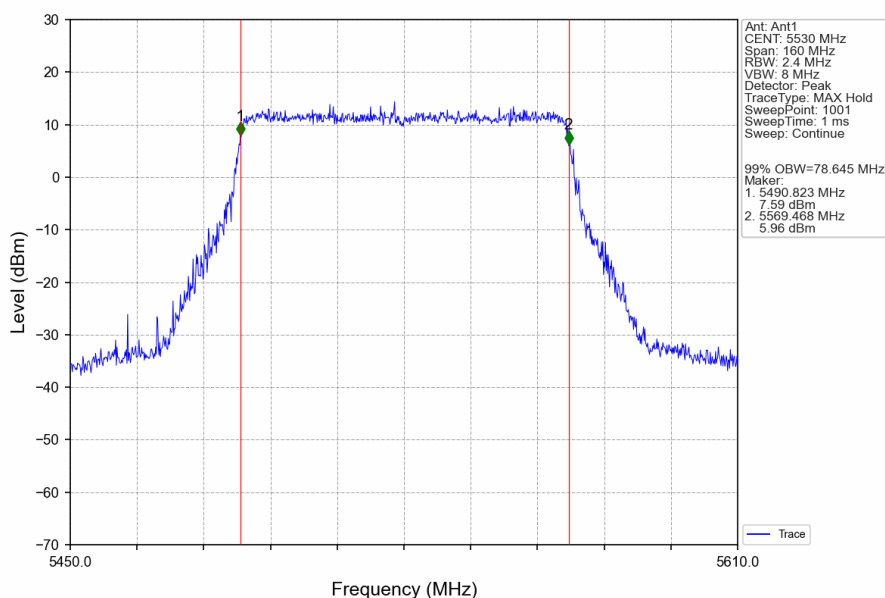
802.11ax(HEW80)_LCH_5530MHz_RU996_Left_Ant1_NTNV
