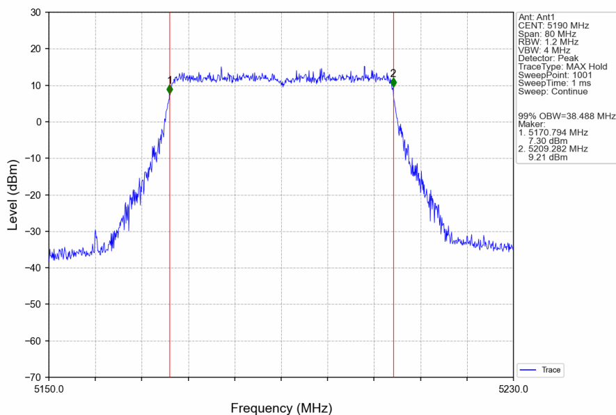
802.11ax(HEW40)_LCH_5190MHz_RU484_Left_Ant1_NTNV
