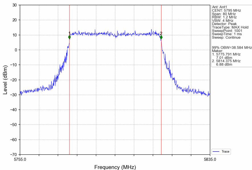
802.11ax(HEW40)_HCH_5795MHz_RU484_Left_Ant1_NTNV
