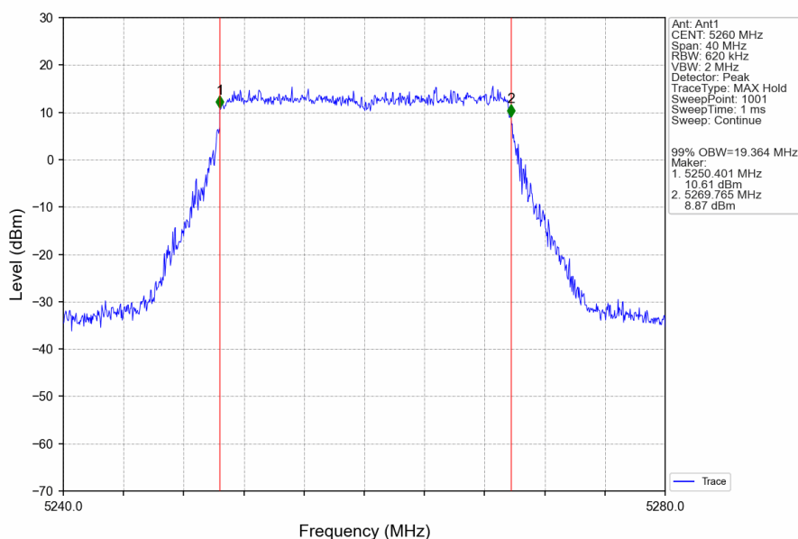
802.11ax(HEW20)_LCH_5260MHz_RU242_Left_Ant1_NTNV
