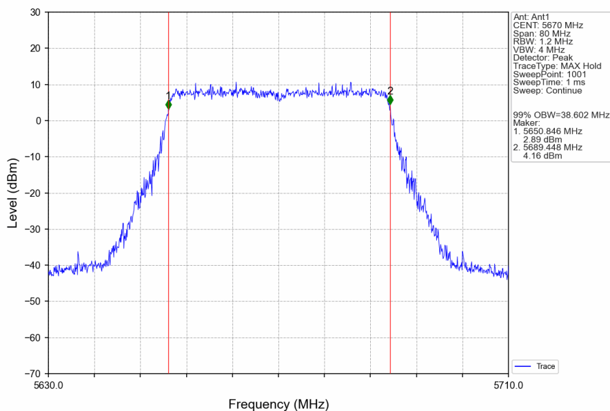
802.11ax(HEW40)_HCH_5670MHz_RU484_Left_Ant1_NTNV
