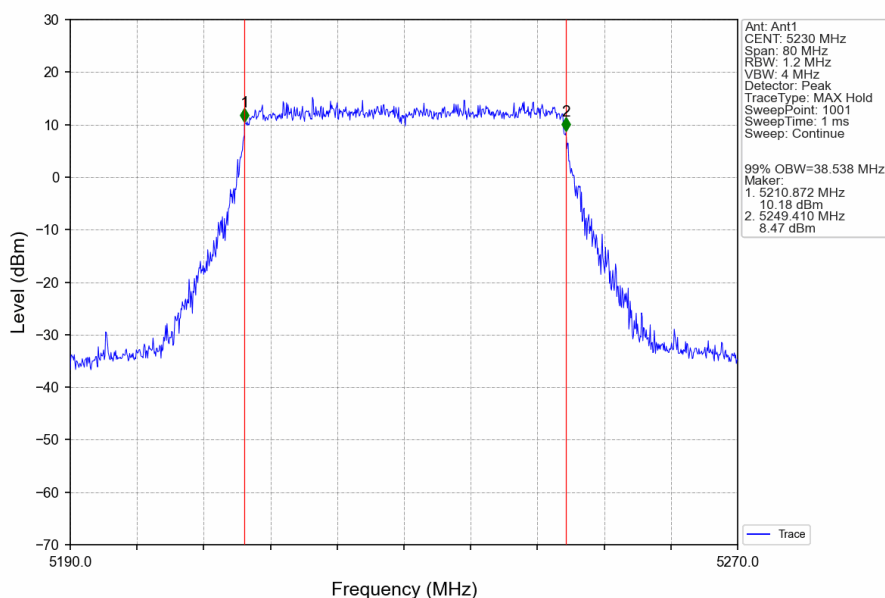
802.11ax(HEW40)_HCH_5230MHz_RU484_Left_Ant1_NTNV
