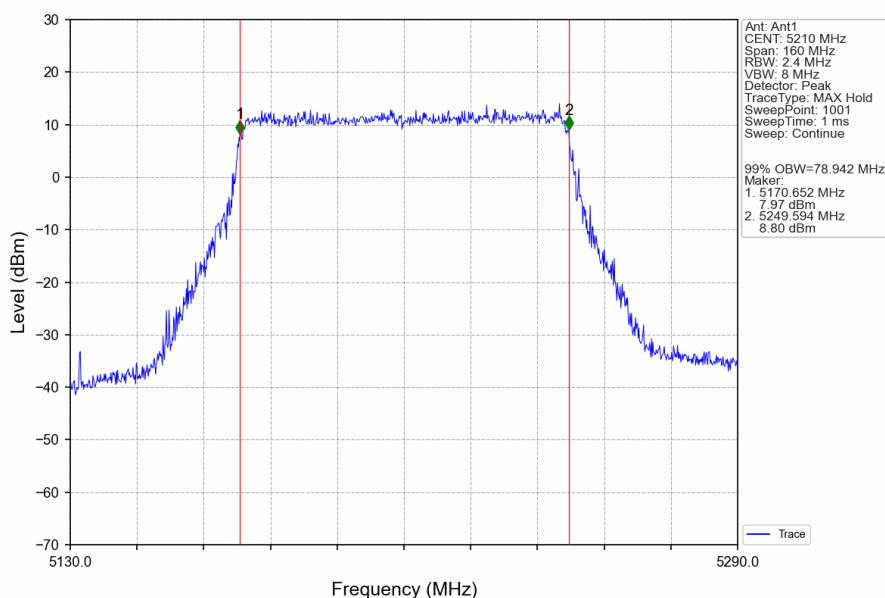
802.11ax(HEW80)_MCH_5210MHz_RU996_Left_Ant1_NTNV
