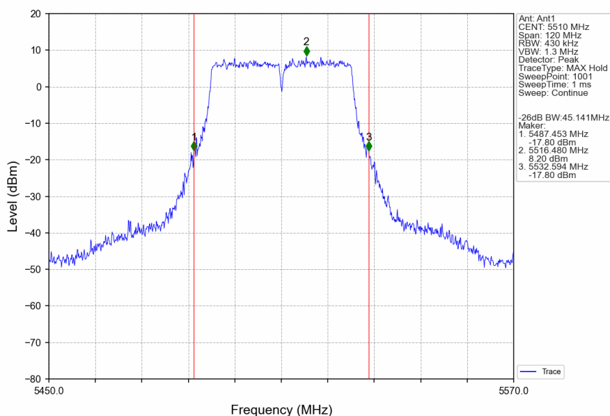
802.11n(HT40)_LCH_5510MHz_Ant1_NTNV
