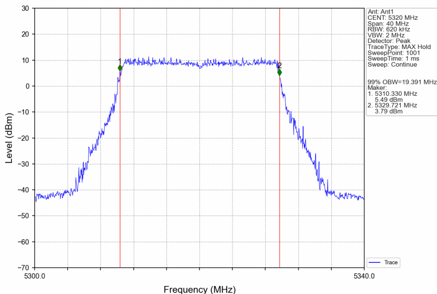
802.11be(EHT20)_HCH_5320MHz_RU242_Left_Ant1_NTNV
