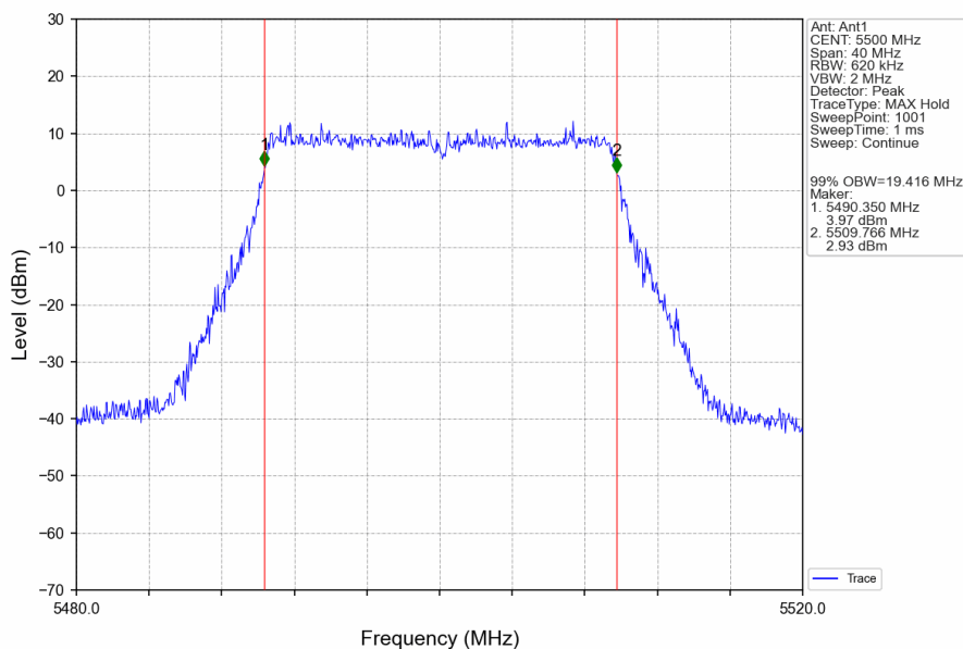
802.11ax(HEW20)_LCH_5500MHz_RU242_Left_Ant1_NTNV
