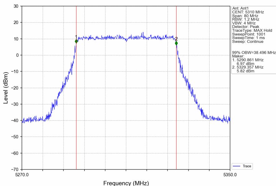
802.11ax(HEW40)_HCH_5310MHz_RU484_Left_Ant1_NTNV
