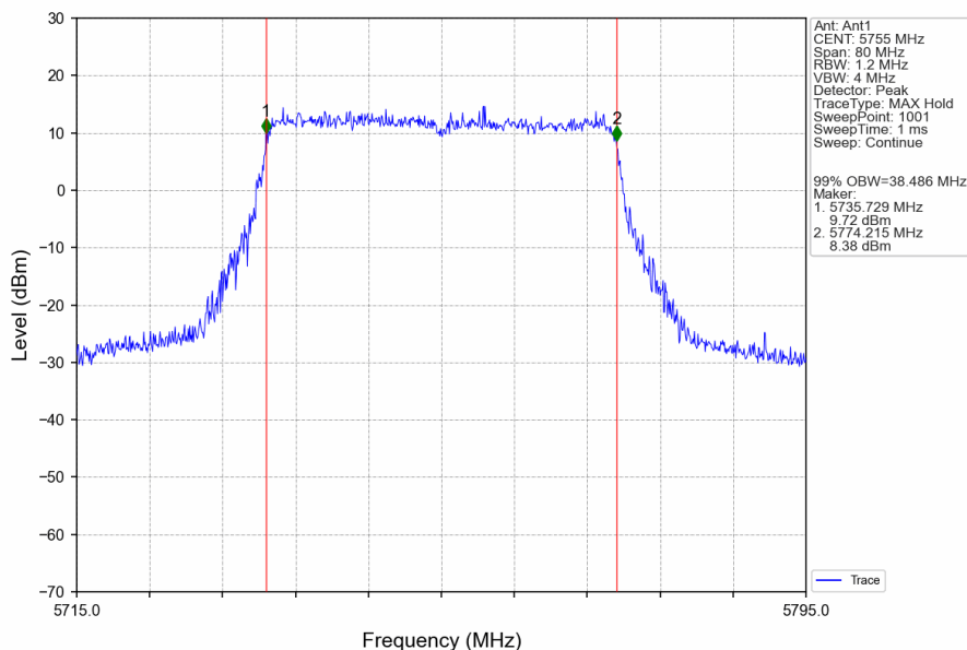
802.11ax(HEW40)_LCH_5755MHz_RU484_Left_Ant1_NTNV
