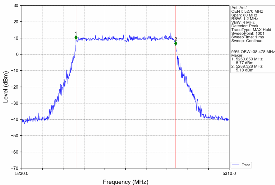
802.11ax(HEW40)_LCH_5270MHz_RU484_Left_Ant1_NTNV
