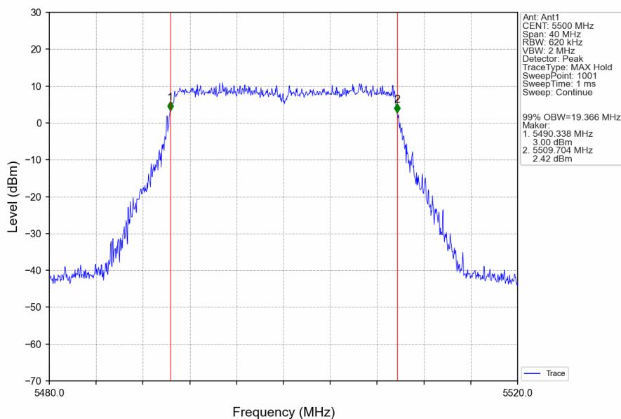
802.11be(EHT20)_LCH_5500MHz_RU242_Left_Ant1_NTNV
