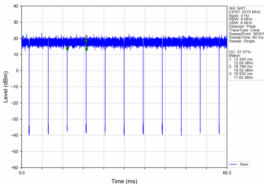
802.11n(HT40)_LCH_5270MHz_Ant1_NTNV
