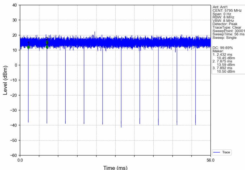
802.11ax(HEW40)_HCH_5795MHz_RU484_Left_Ant1_NTNV
