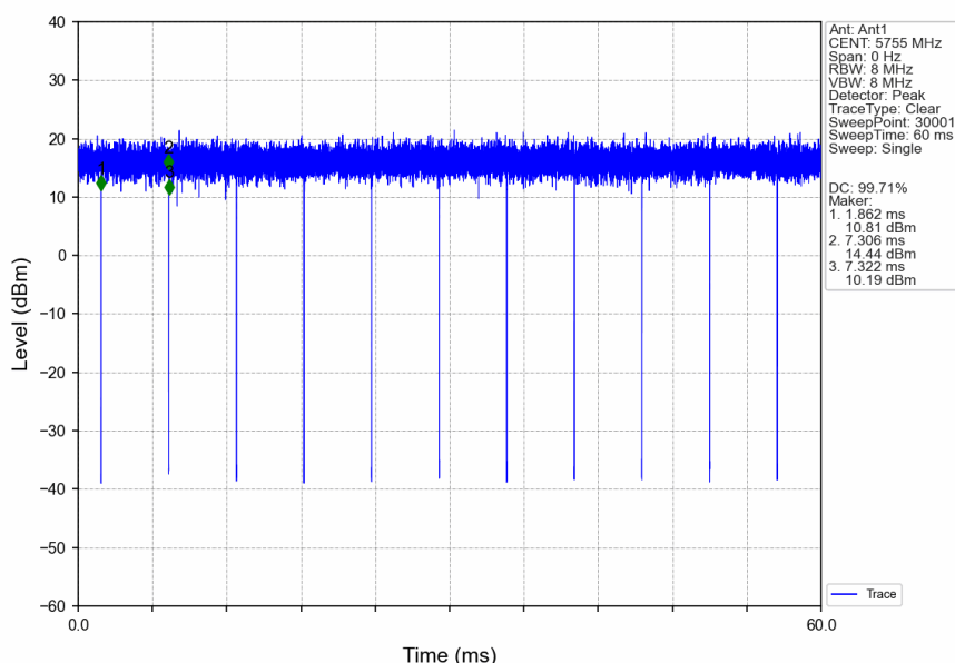
802.11ax(HEW40)_LCH_5755MHz_RU484_Left_Ant1_NTNV
