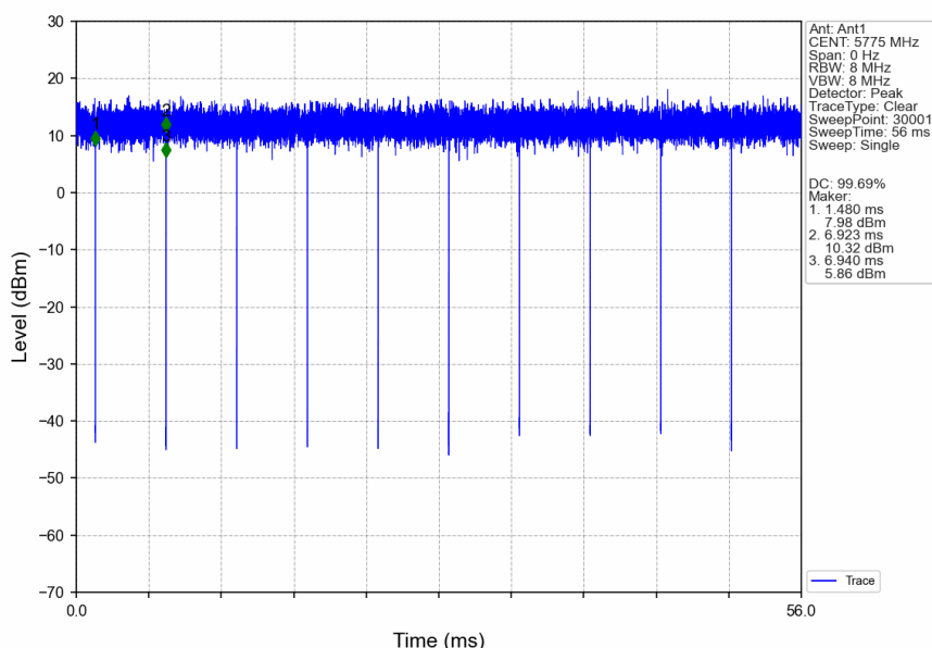
802.11ax(HEW80)_MCH_5775MHz_RU996_Left_Ant1_NTNV
