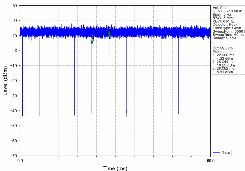
802.11ax(HEW80)_MCH_5210MHz_RU996_Left_Ant1_NTNV
