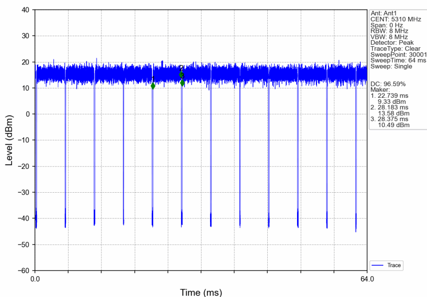
802.11ax(HEW40)_HCH_5310MHz_RU484_Left_Ant1_NTNV
