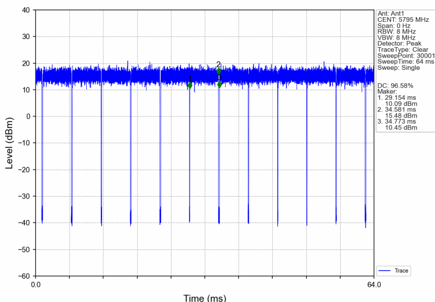
802.11n(HT40)_HCH_5795MHz_Ant1_NTNV
