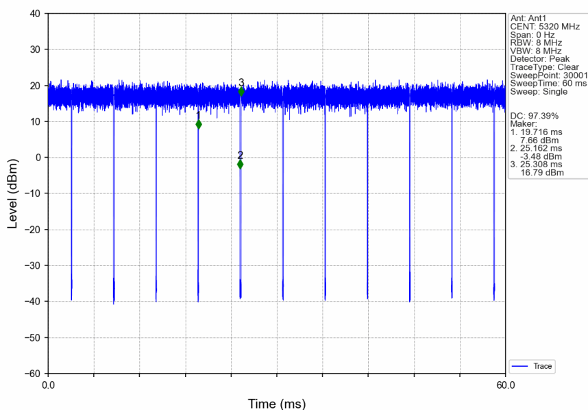
802.11ax(HEW20)_HCH_5320MHz_RU242_Left_Ant1_NTNV
