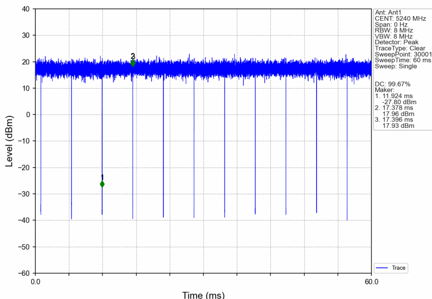
802.11be(EHT20)_HCH_5240MHz_RU242_Left_Ant1_NTNV
