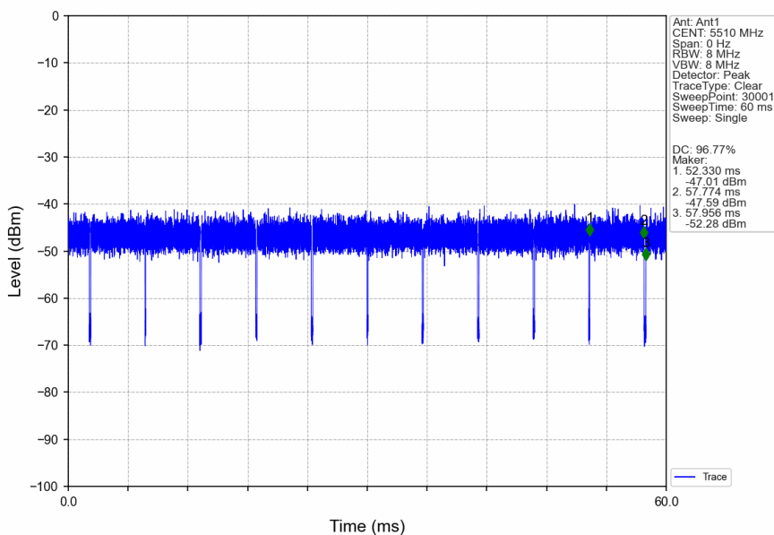
802.11ax(HEW40)_LCH_5510MHz_RU484_Left_Ant1_NTNV
