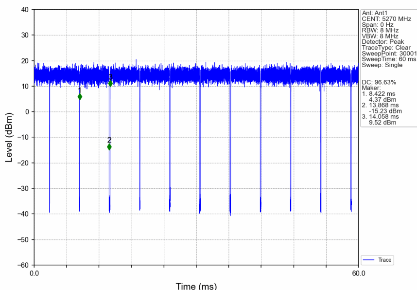
802.11ax(HEW40)_LCH_5270MHz_RU484_Left_Ant1_NTNV
