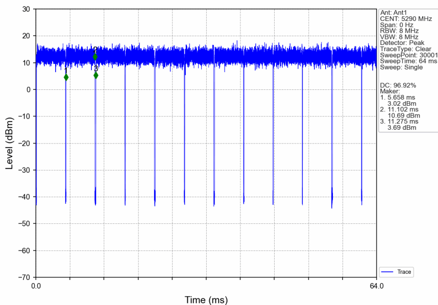
802.11ax(HEW80)_MCH_5290MHz_RU996_Left_Ant1_NTNV
