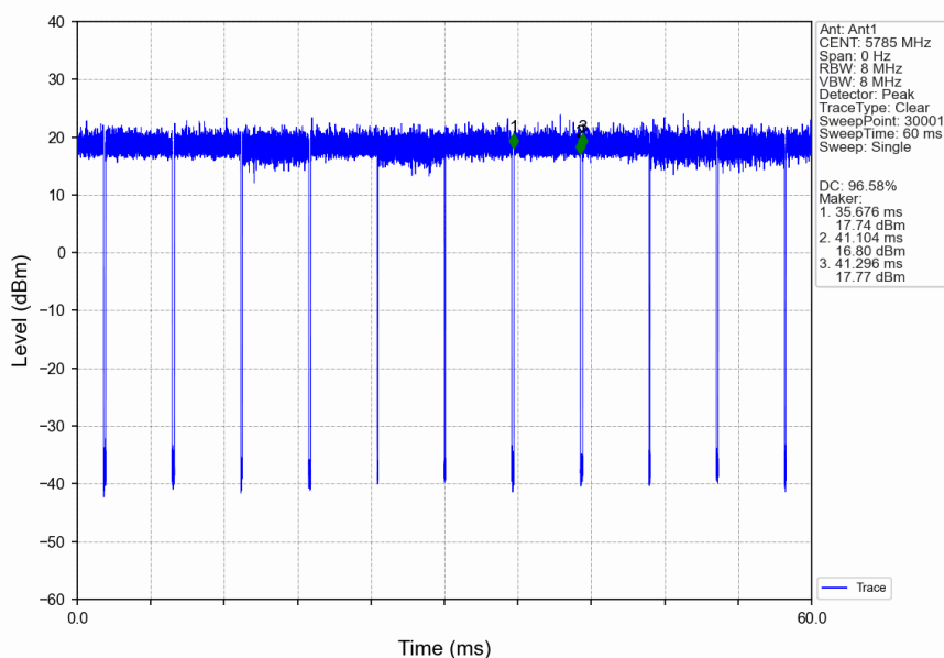
802.11n(HT20)_MCH_5785MHz_Ant1_NTNV
