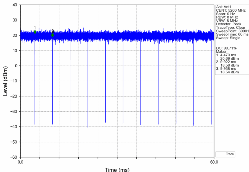
802.11be(EHT20)_MCH_5200MHz_RU242_Left_Ant1_NTNV
