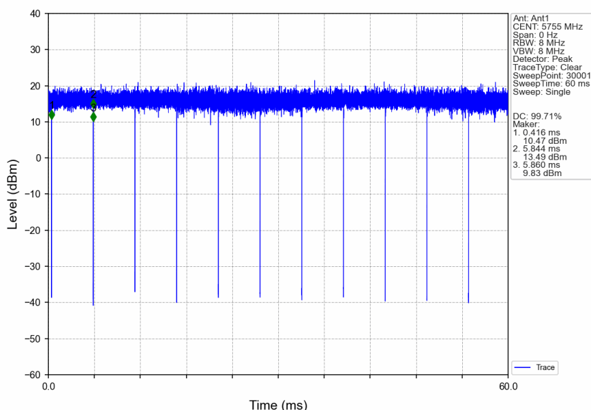
802.11ac(VHT40)_LCH_5755MHz_Ant1_NTNV
