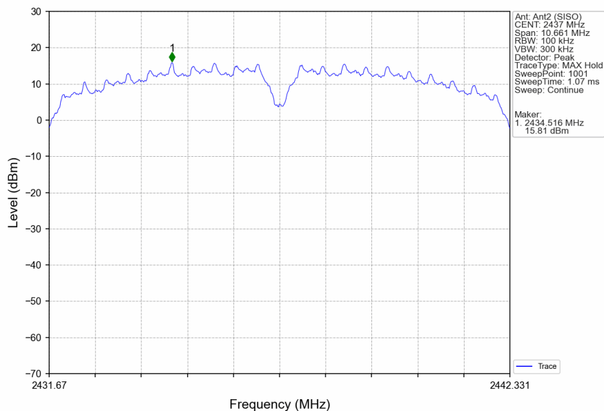
802.11b_MCH_2437MHz_Ant2 (SISO)_NTNV
