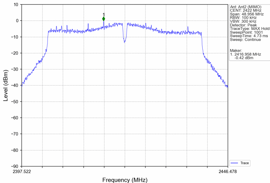
802.11n(HT40)_LCH_2422MHz_Ant2 (MIMO)_NTNV
