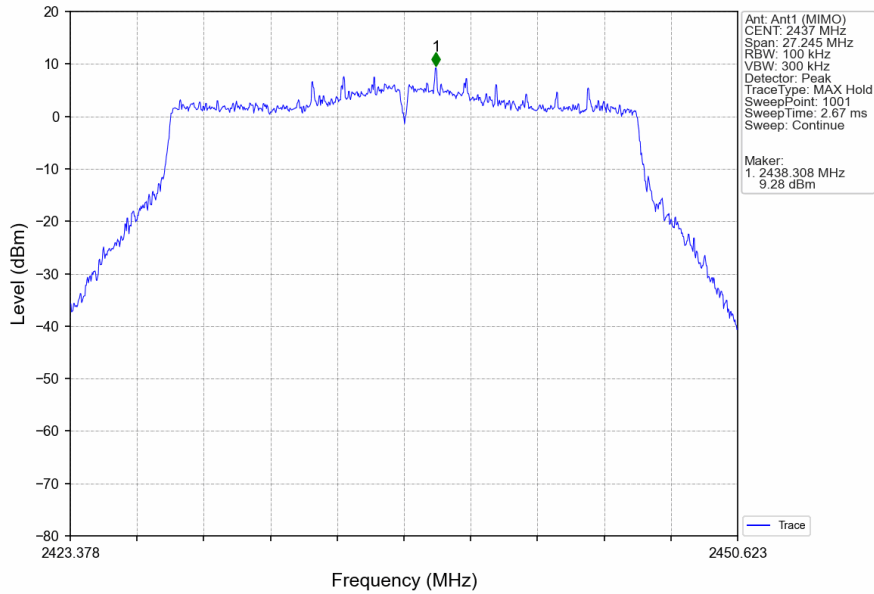
802.11ax(HEW20)_MCH_2437MHz_SU_/_Ant1 (MIMO)_NTNV
