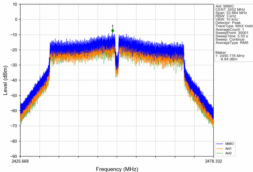
802.11n(HT40)_HCH_2452MHz_MIMO_NTNV
