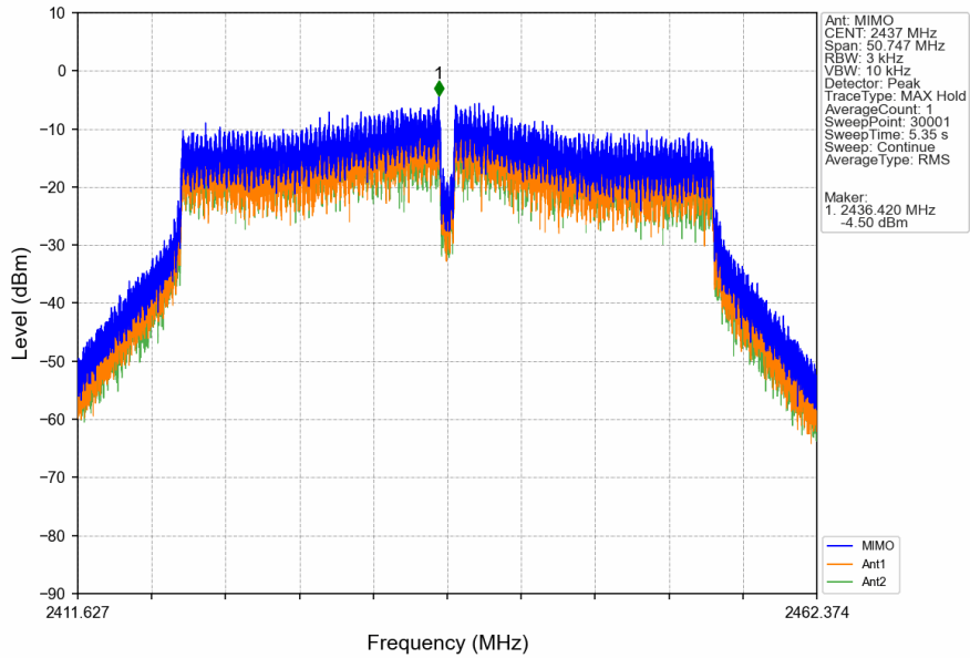
802.11n(HT40)_MCH_2437MHz_MIMO_NTNV
