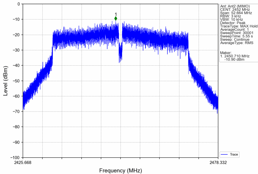
802.11n(HT40)_HCH_2452MHz_Ant2 (MIMO)_NTNV
