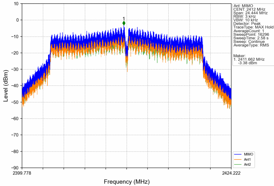
802.11n(HT20)_LCH_2412MHz_MIMO_NTNV
