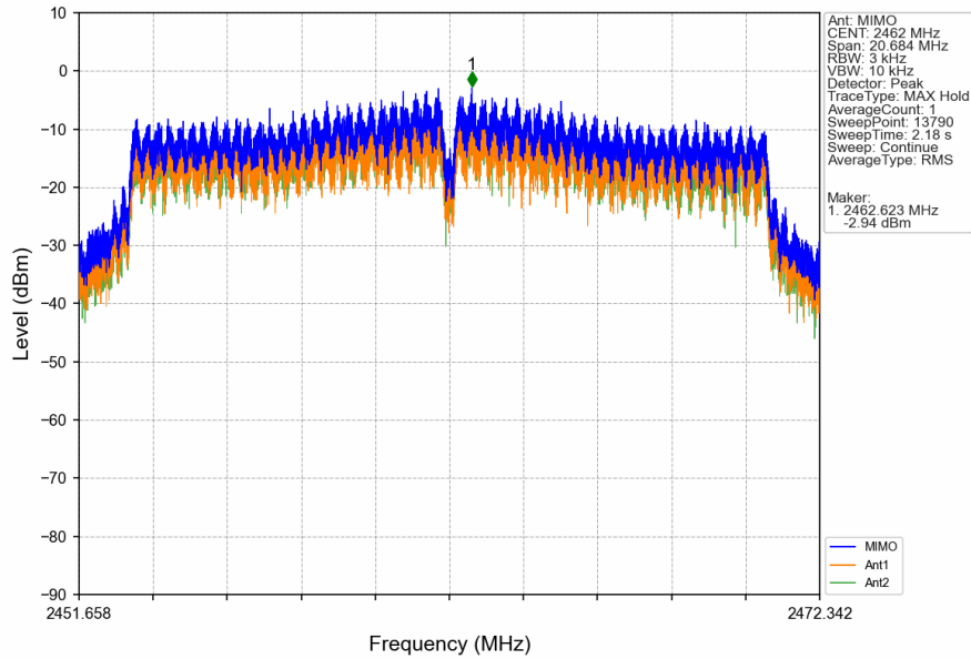
802.11n(HT20)_HCH_2462MHz_MIMO_NTNV
