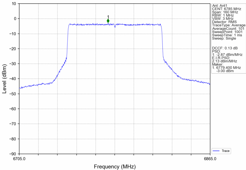
802.11be(EHT80)_HCH_6785MHz_RU996_Left_Ant1_NTNV
