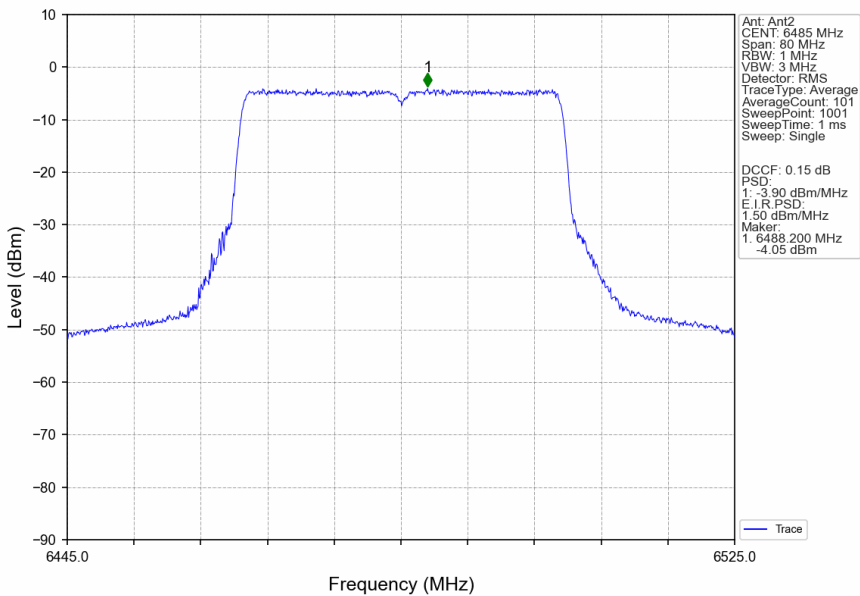
802.11be(EHT40)_MCH_6485MHz_RU484_Left_Ant2_NTNV
