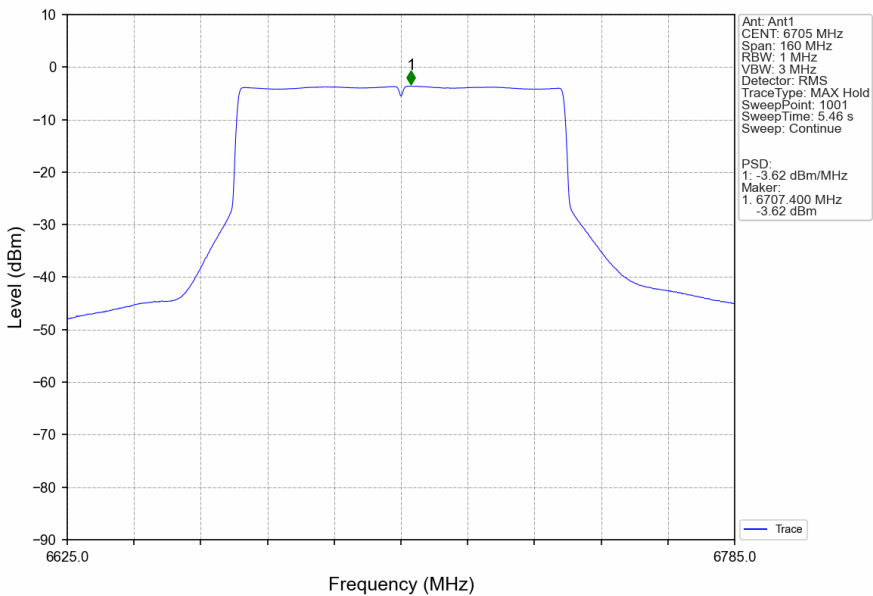
802.11be(EHT80)_MCH_6705MHz_RU996_Left_Ant1_NTNV
