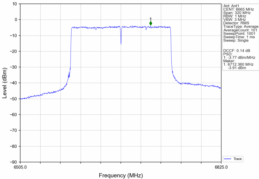
802.11be(EHT160)_MCH_6665MHz_2xRU996_Left_Ant1_NTNV
