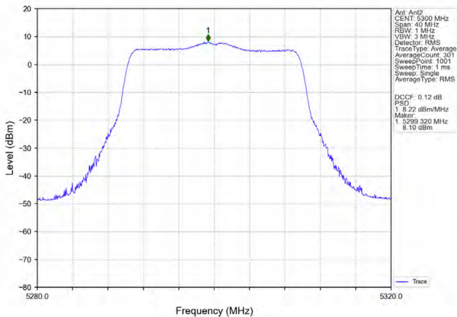
802.11be(EHT20)_MCH_5300MHz_SU_/_Ant2_NTNV
