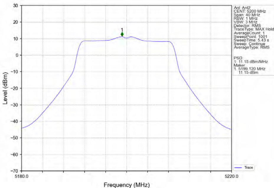
802.11n(HT20)_MCH_5200MHz_MIMO_NTNV
