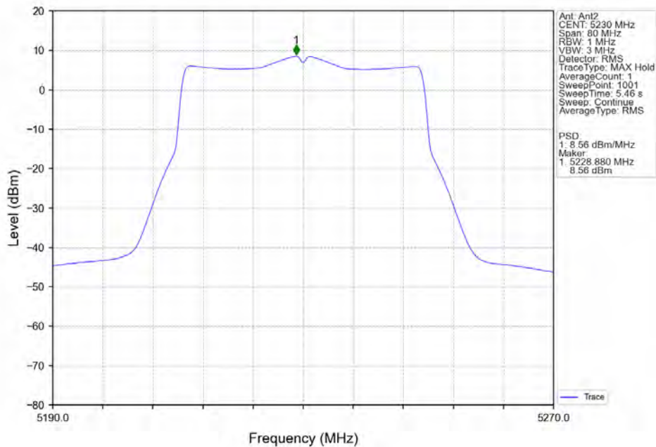
802.11be(EHT40)_HCH_5230MHz_SU_/_Ant2_NTNV
