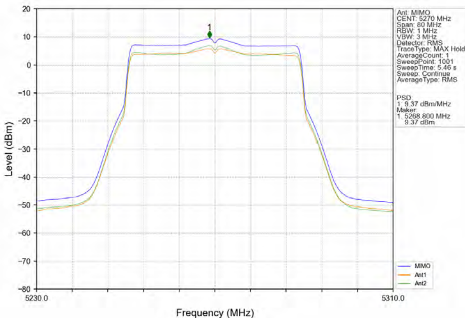
802.11be(EHT40)_LCH_5270MHz_SU_/_MIMO_NTNV
