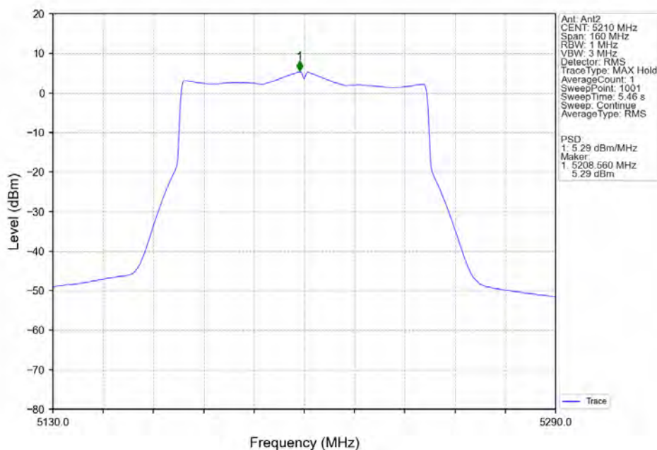
802.11be(EHT80)_MCH_5210MHz_SU_ / _Ant2_NTNV
