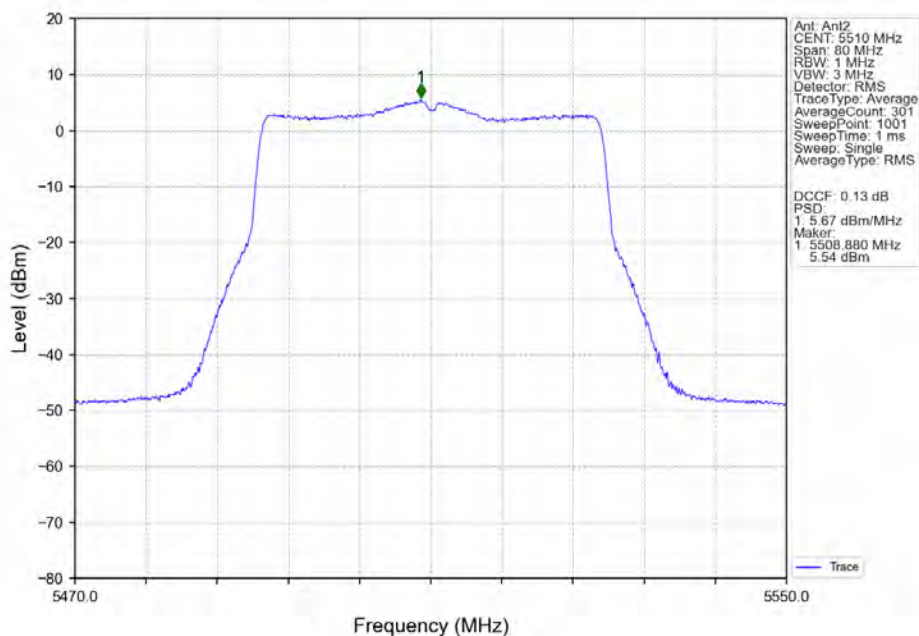
802.11be(EHT40)_LCH_5510MHz_SU_/_MIMO_NTNV
