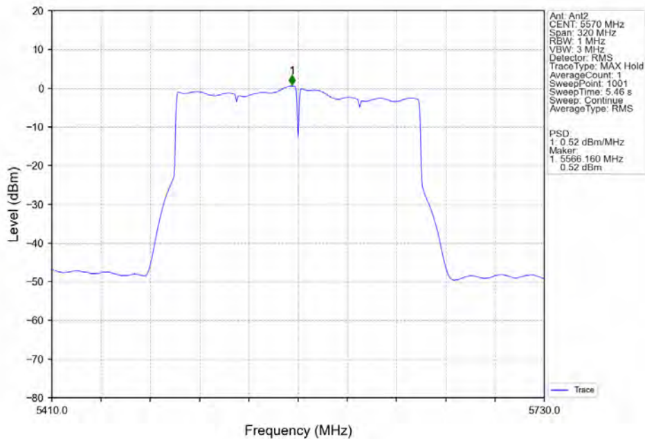
802.11be(EHT160)_MCH_5570MHz_SU_ / _Ant2_NTNV
