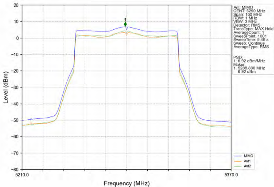
802.11be(EHT80)_MCH_5290MHz_SU_/_MIMO_NTNV
