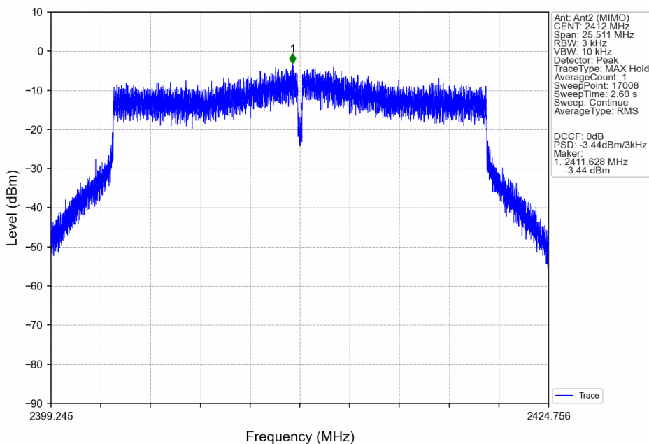
802.11be(EHT20)_LCH_2412MHz_SU_ / _Ant2 (MIMO)_NTNV
