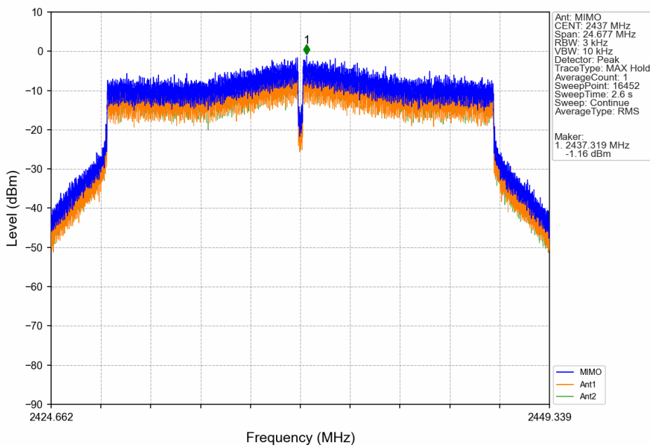
802.11ax(HEW20)_MCH_2437MHz_SU_/_MIMO_NTNV
