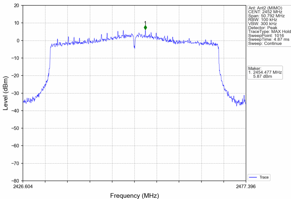
802.11ax(HEW40)_HCH_2452MHz_RU484_Left_Ant2 (MIMO)_NTNV
