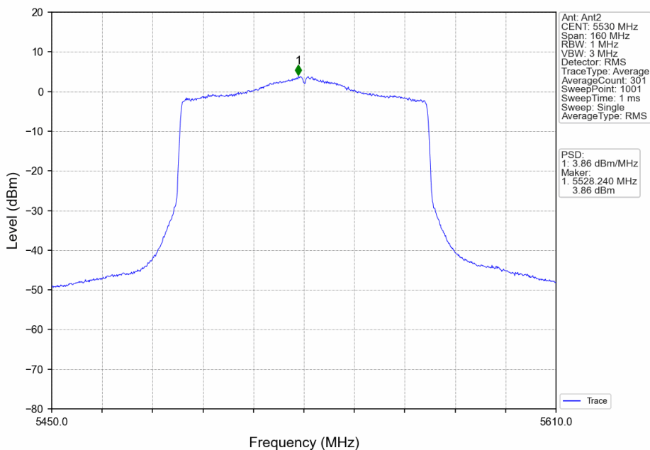
802.11ax(HEW80)_LCH_5530MHz_RU996_Left_Ant2_NTNV
