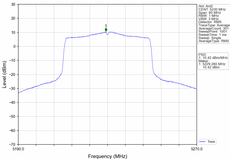
802.11ax(HEW40)_HCH_5230MHz_RU484_Left_Ant2_NTNV
