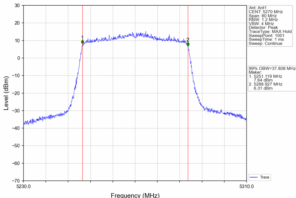
802.11ax(HEW40)_LCH_5270MHz_RU484_Left_Ant1_NTNV
